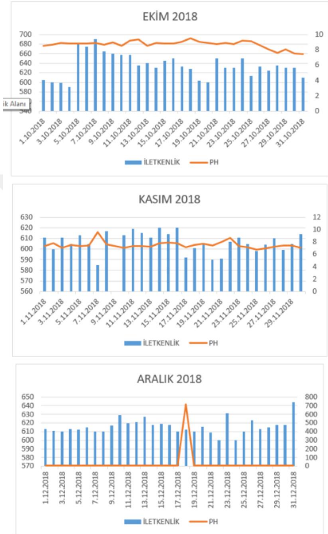
Şekil 5.8. Hamsu pH ve İletkenlik Ekim-Kasım-Aralık Ayı Değişim Grafiği
