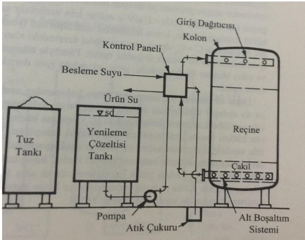
Şekil 6.7. Sodayum yüklü bir reçine kullanılarak yumuşatma için sabit yataklı kolon sistemi
