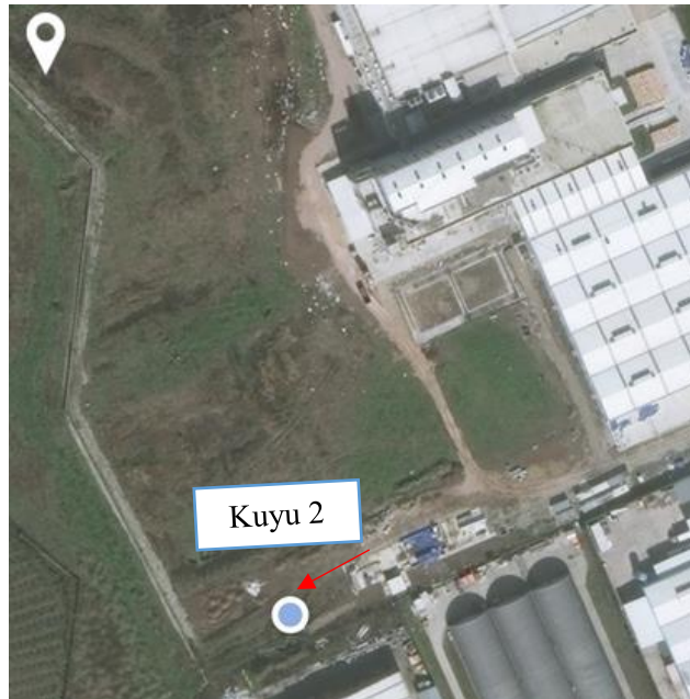
Şekil 2.3. İnceleme alanına ait uydu fotoğrafı Kuyu-2 (Google,2019) Enlem: 40°45.727' Boylam: 30° 38. 454'
