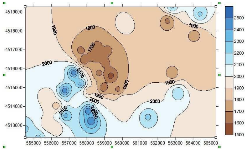
Şekil 4.3. 2. tabakalara ait boyuna dalga hız (P) haritası.
