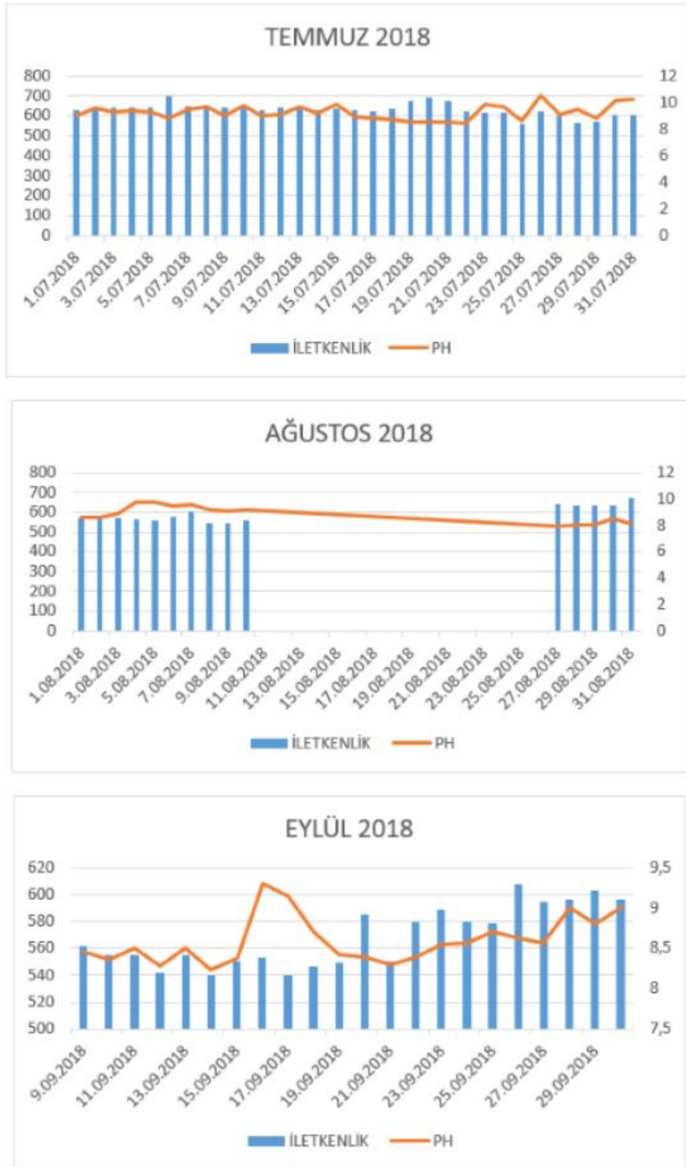
Şekil 5.7. Hamsu pH ve İletkenlik Temmuz-Ağustos-Eylül Ayı Değişim Grafiği
