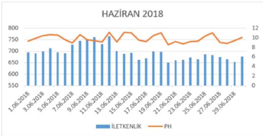
Şekil 5.6. Hamsu pH ve İletkenlik Nisan-Mayıs-Haziran Ayı Değişim Grafiği
