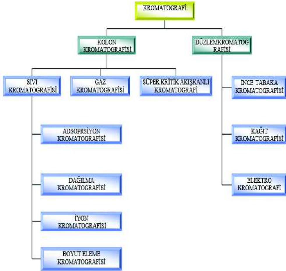
Şekil 4.1. Kromatografik yöntemlerin sınıflandırılması [24].
