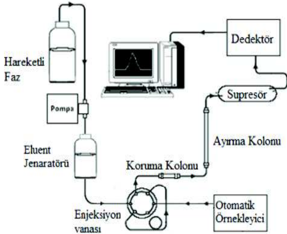
Şekil 5.1. İyon kromatografi cihazının kısımları [20].
