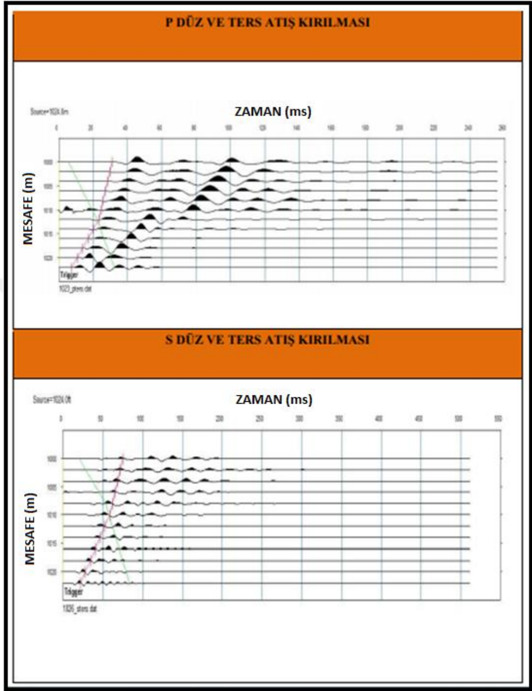
Şekil 3.16. Sismik-5 düz ve ters atış kırılma verileri
