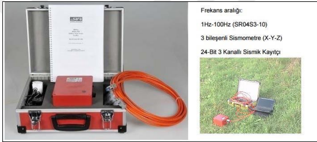
Şekil 3.21. Mikrotremör ölçümlerinde kullanılan cihazın görüntüsü ve özellikleri
