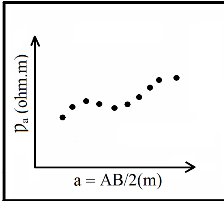
Şekil 3.28. DES ölçümü sonucu elde edilen görünür özdirenç eğrisi
