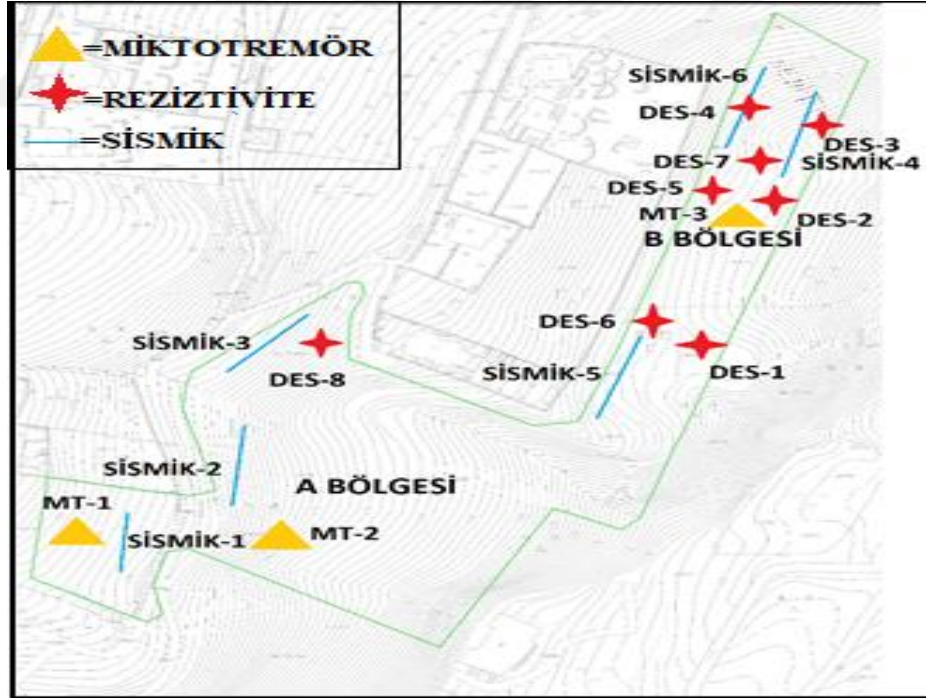
Şekil 3.1. Jeofizik Ölçülerin Sismik, Rezistivite ve Mikrotremör Sahadaki Konumu
