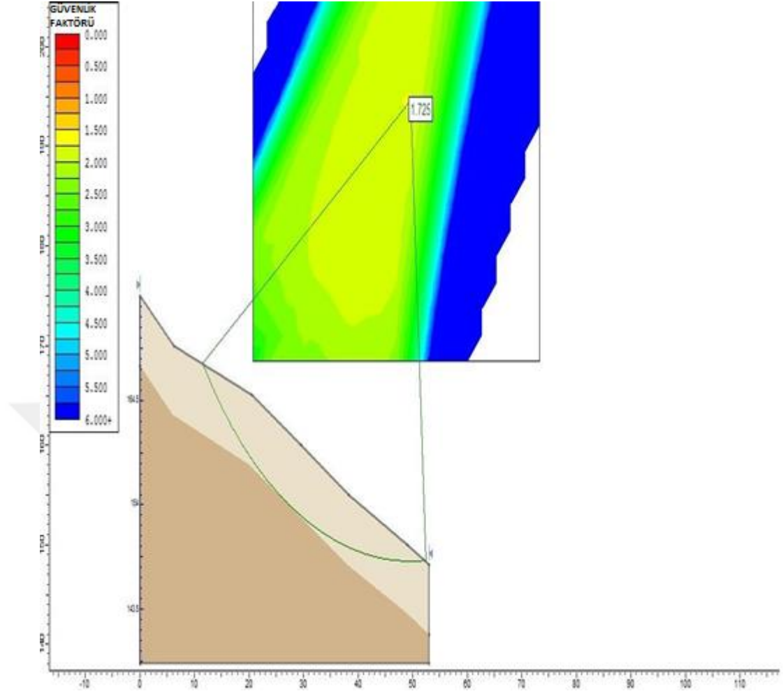
Şekil 3.55. Kesit-1(şev stabilite analizi)
