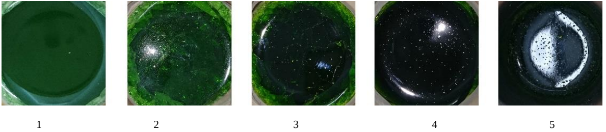
Görsel 4.13. 1150^\circ\text{C} 'de krom(III)oksit ( \text{Cr}_2\text{O}_3 ) kullanarak üretilen yeşil camlar. Sırayla soldan : 1: %0.1, 2: %0.3, 3: %0.5, 4: %1 ve 5: %3.
