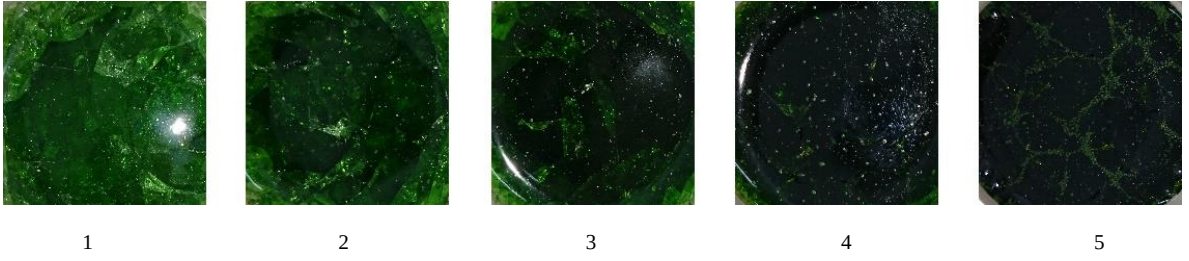
Görsel 4.14. 1100°C’de krom(III)oksit ( \text{Cr}_2\text{O}_3 ) kullanarak üretilen yeşil camlar. Sırayla soldan : 1: %0.1, 2: %0.3, 3: %0.5, 4: %1 ve 5: %3.
