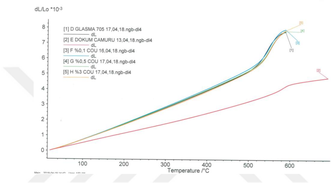
Görsel 4.35. Lacivert serisi, Glasma 705 ve döküm çamuru Dilatometre analizlerin karşılaştırılması
