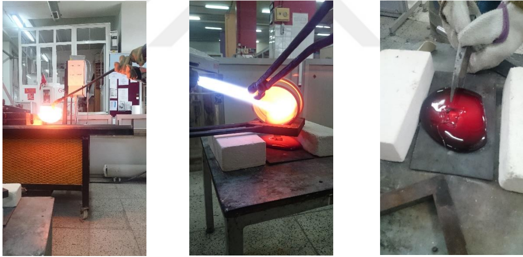
Görsel 4.6. Sıcak cam döküm aşamaları
