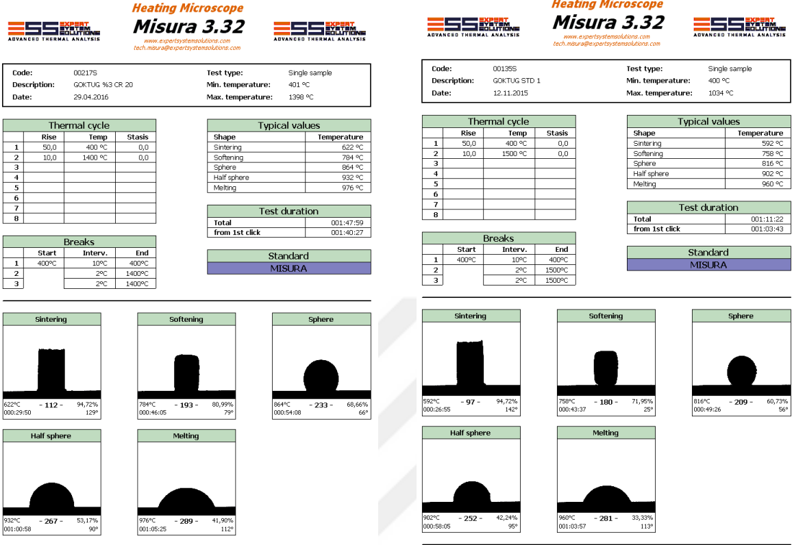
Görsel 5.16. %3 Krom oksit içerikli yeşil cam ve Glasma 705 camın Isı Mikroskobu analizlerin karşılaştırılması
