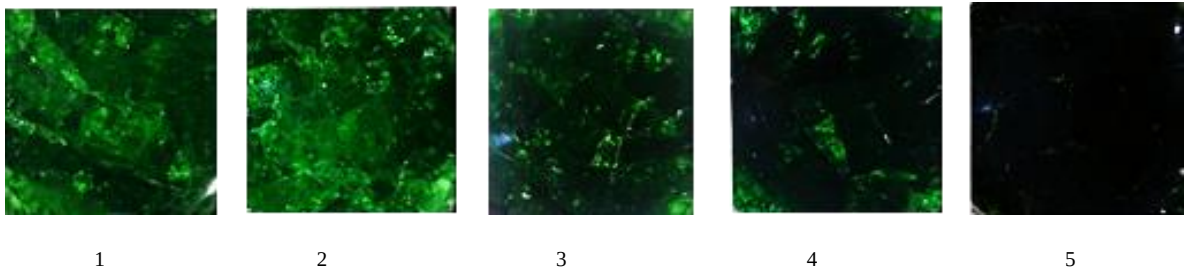
Görsel 4.21. 1200 °C'de üretilen camlar; 1: 0.1% Cr_2O_3 + 0.1% Fe_2O_3 , 2: 0.1% Cr_2O_3 + 0.1% CuO, 3: 0.3% Cr_2O_3 + 0.3 Fe_2O_3 , 4: 0.3% Cr_2O_3 + 0.3% CuO, 5: 2.5% Cr_2O_3 + 2.5% Fe_2O_3
