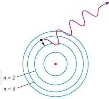
Grsel 3.12. Foton emisyonu (yayılımı)
