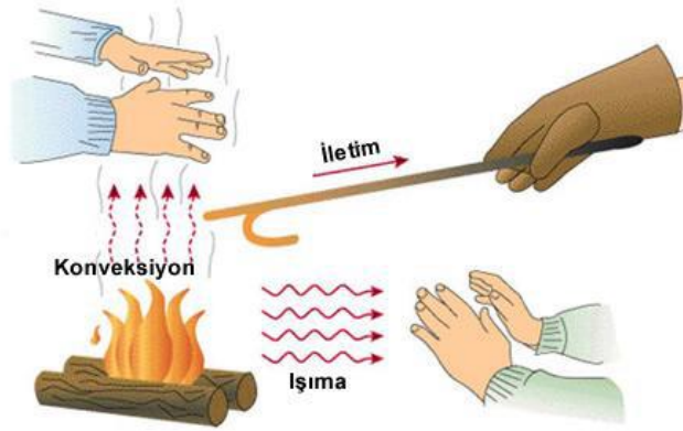
Görsel 5.17. Isının yayılma yolları
