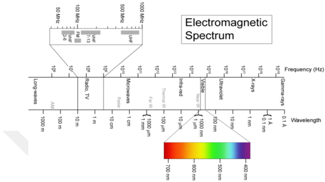
Görsel 3.2. Elektromanyetik spektrumun şematik gösterimi.
