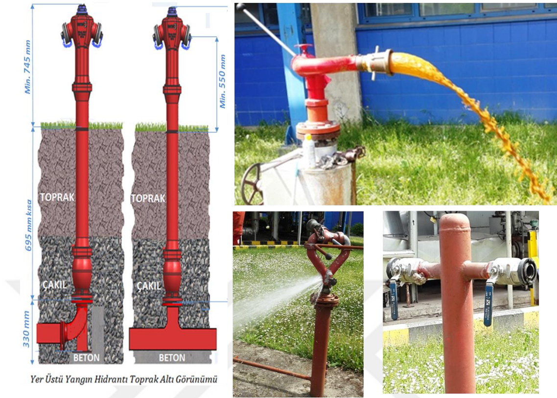
Şekil 2.47. Yangın hidrant ve monitörler
