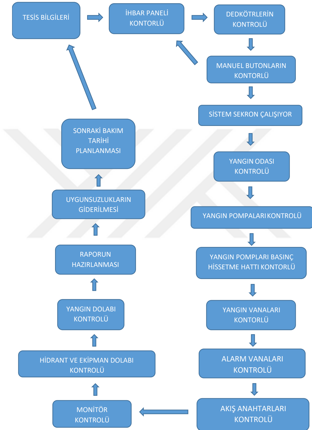
Şekil 2.56. Yangın söndürme sistemi bakımlarının yapılması
