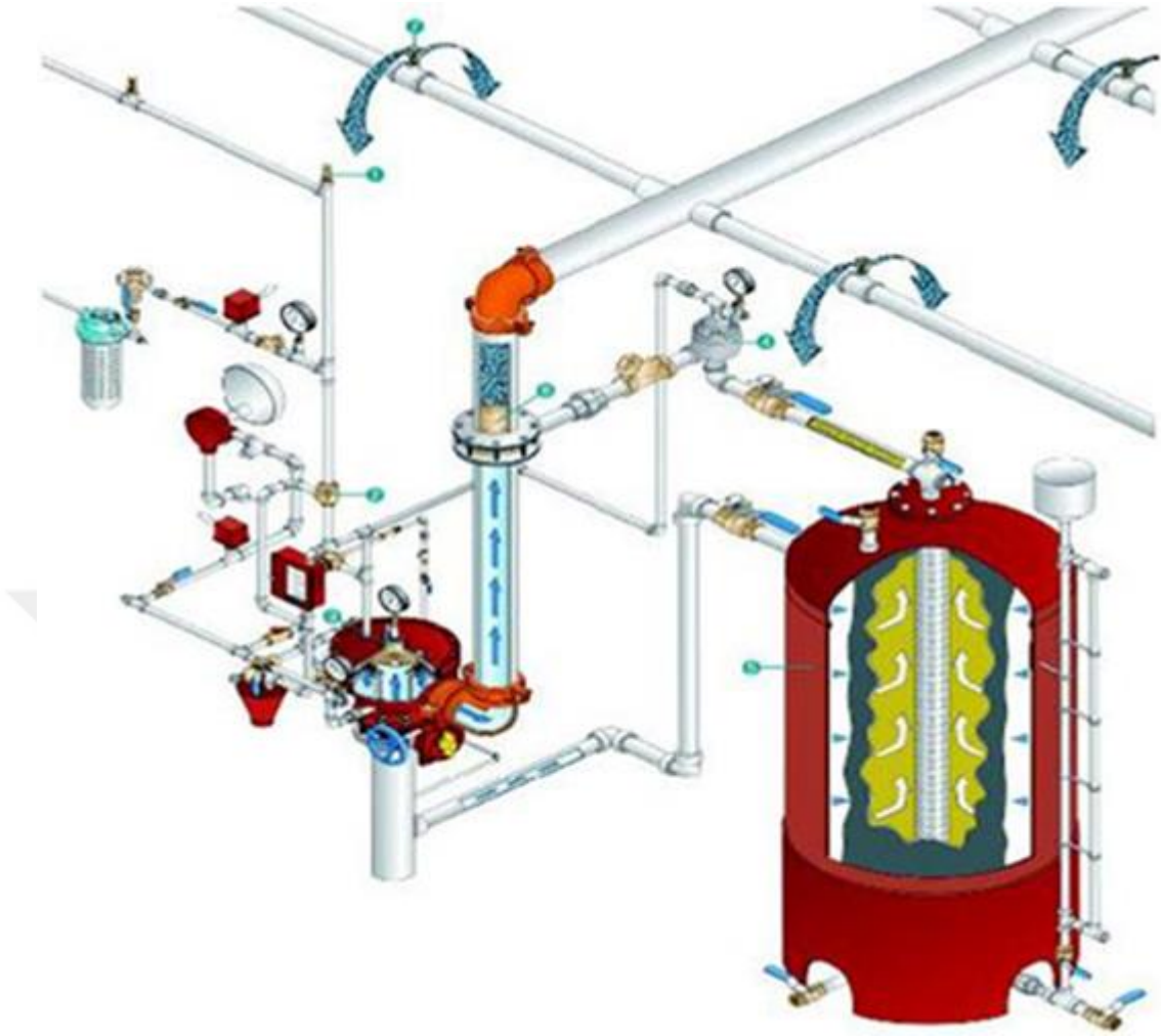
Şekil 2.10. Köpük sistemi genel görünümü
