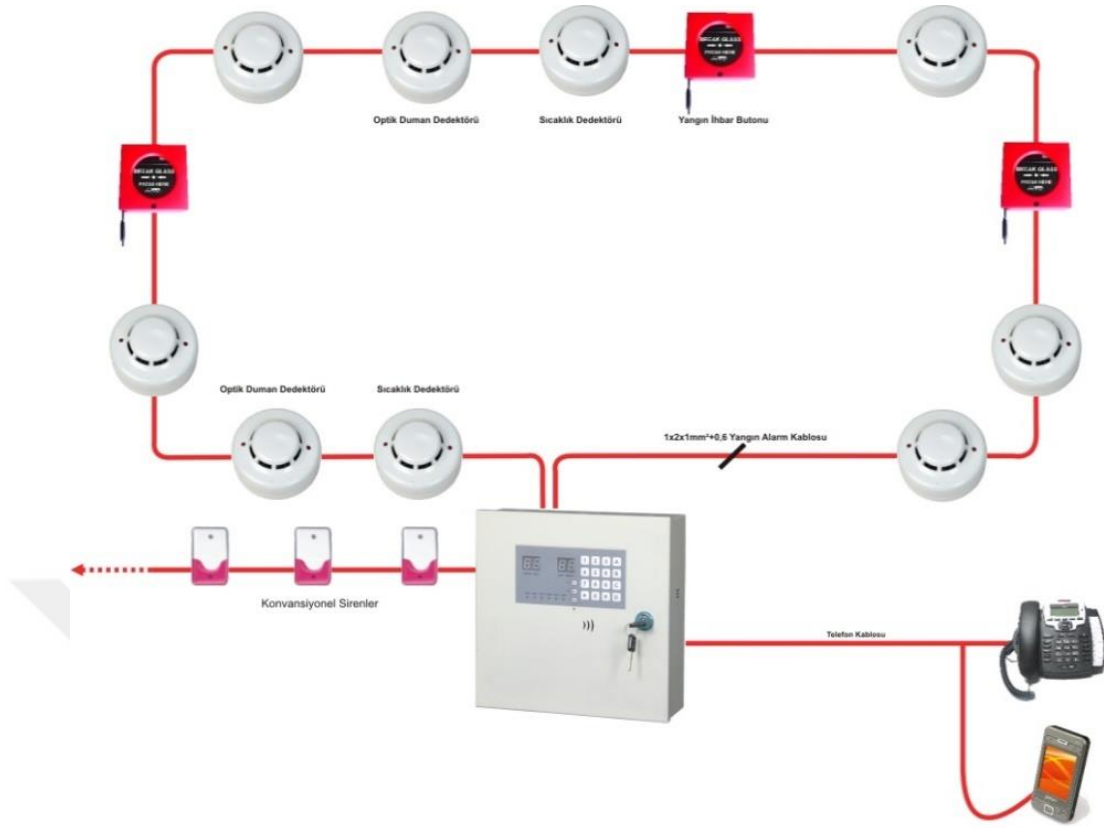
Şekil 2.16. Yangın algılama sistemi genel gösterimi
