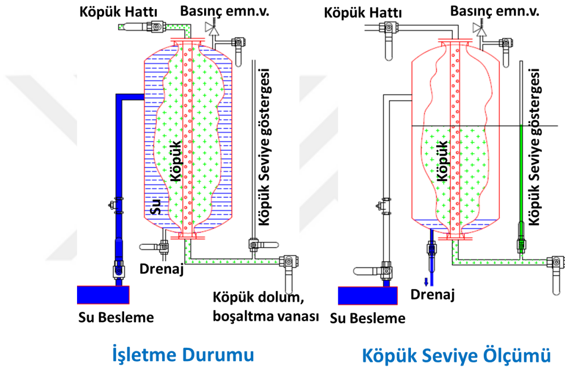
Şekil 2.43. Blader tank köpük seviye ölçümü görseli
