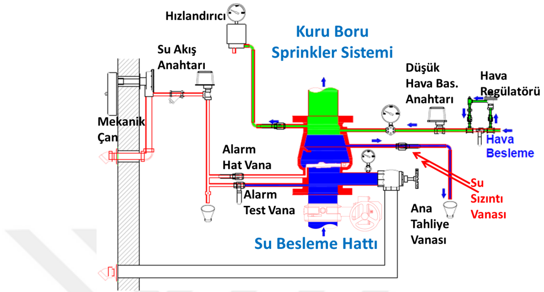
Şekil 2.38. Kuru alarm vanası aylık kontrol
