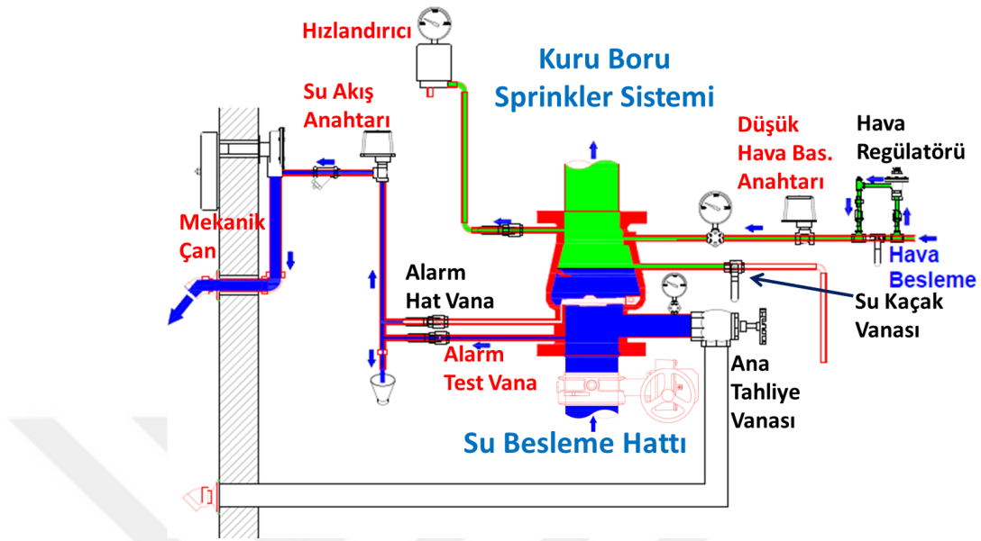
Şekil 2.39. Kuru alarm vanası 3 aylık kontrol
