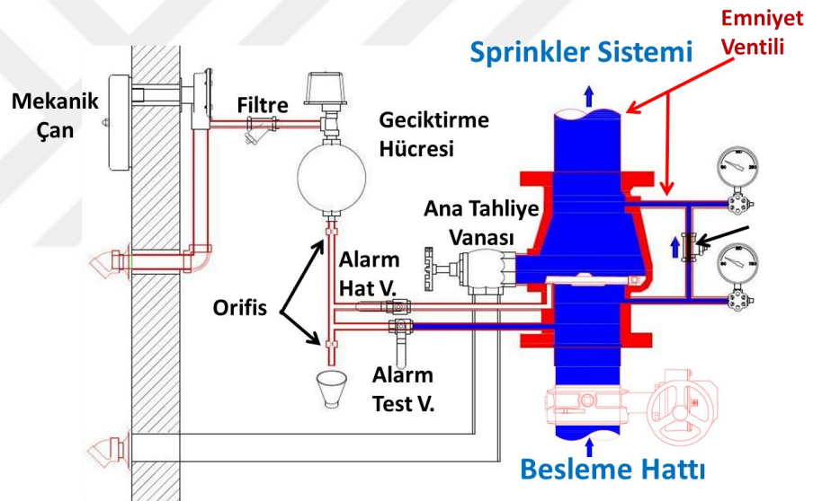
Şekil 2.35. Islak alarm vanası aylık kontrol
