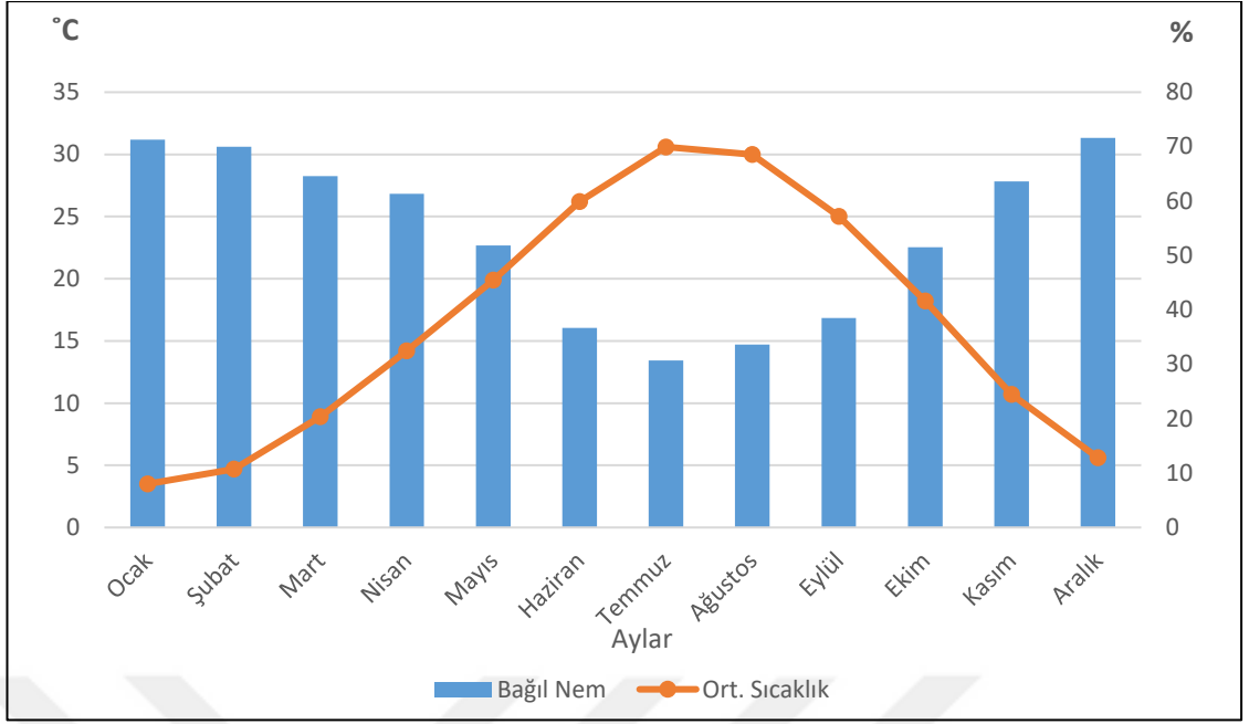
Grafik 6: Siverek'te Bağıl Nem ve Ortalama Sıcaklık Grafiği (1963-2015, Tablo 1 ve Tablo 8'e göre)
