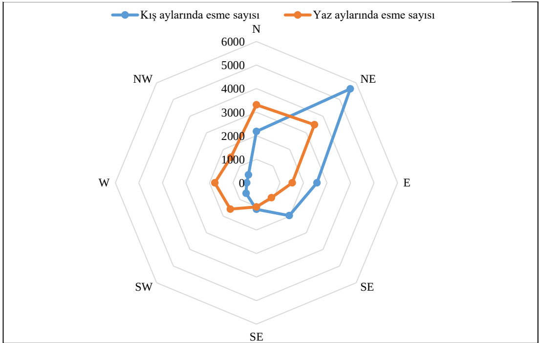
Grafik 5: Siverek'te Rüzgarların Yaz ve Kış Aylarına Göre Esme Sayısı Ortalamaları (1963-2015, Tablo 4'e göre)
