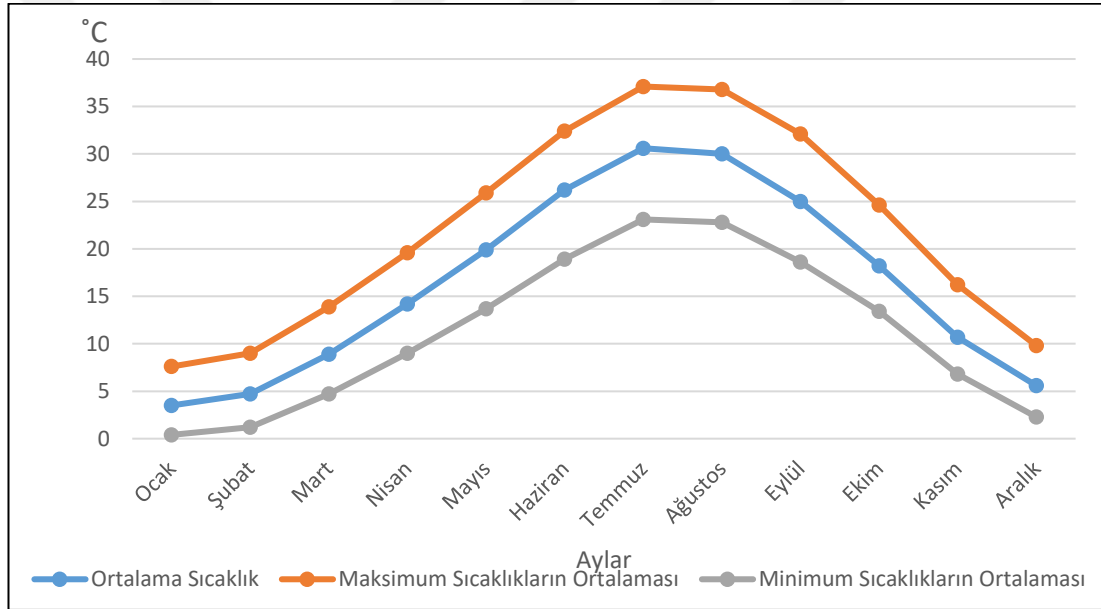
Grafik 2: Siverek'in Sıcaklık Değerlerinin Grafiği (1963-2015, Tablo 1'e göre)
