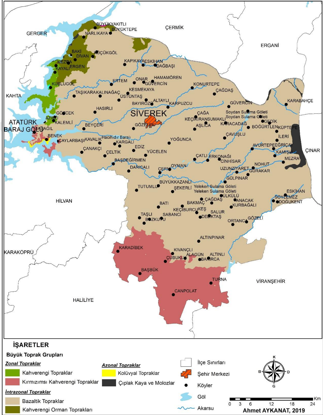
Harita 8: Siverek İlçesinde Yer Alan Büyük Toprak Grupları Haritası
