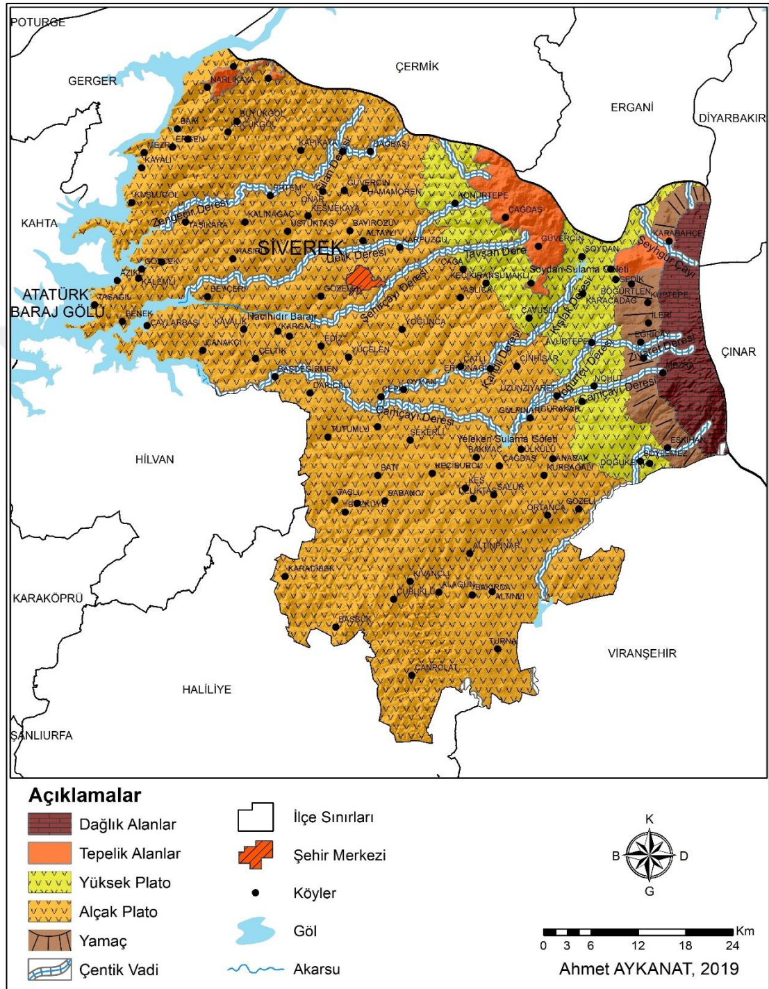
Harita 3: Siverek İlçesi Jeomorfoloji Haritası
