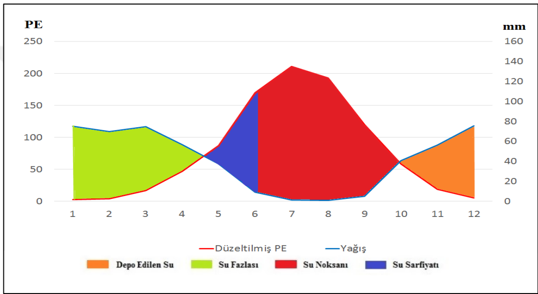
Grafik 9: Siverek'in Thornthwaite'e Göre Su Bilançosu Grafiği (1963-2015)
