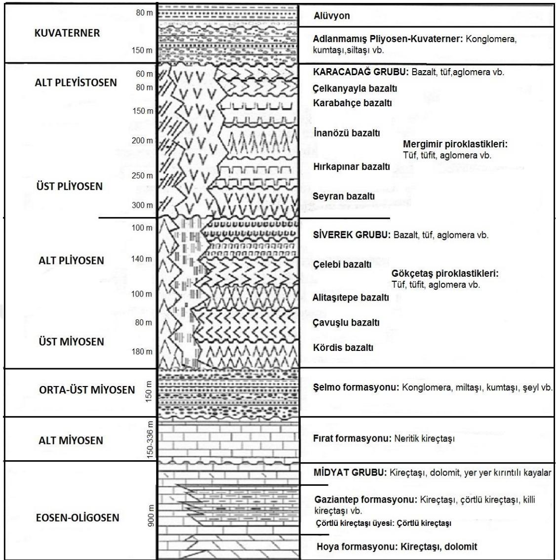
Grafik 1: Siverek İlçesi Stratigrafik Kesiti (Sütçü, 2009'dan yararlanılmıştır.)
