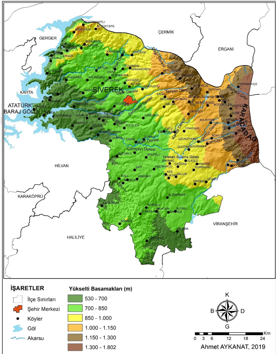
Harita 4: Siverek İlçesi Fiziki Haritası
