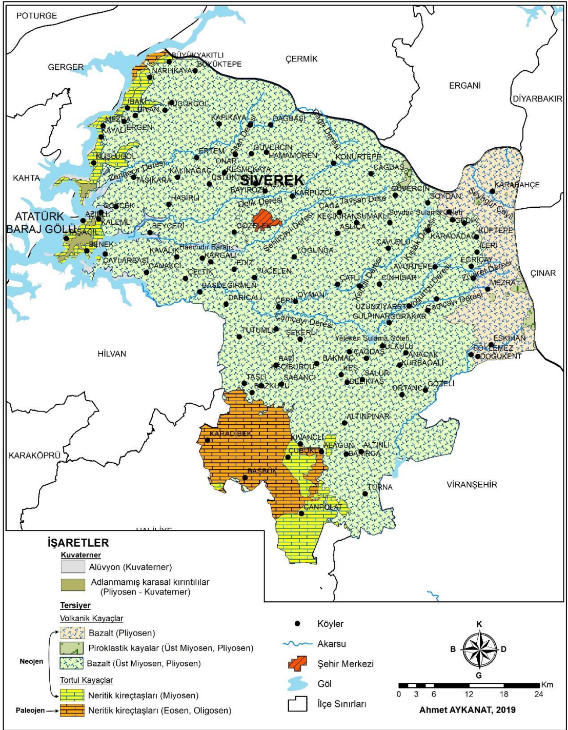
Harita 2: Siverek İlçesi Jeoloji Haritası (MTA, 2009'dan yararlanılmıştır.)
