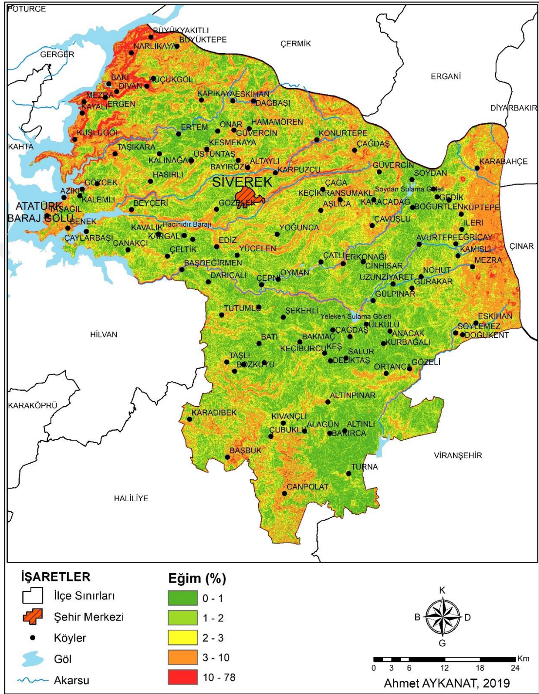
Harita 9: Siverek İlçesi Eğim Haritası
