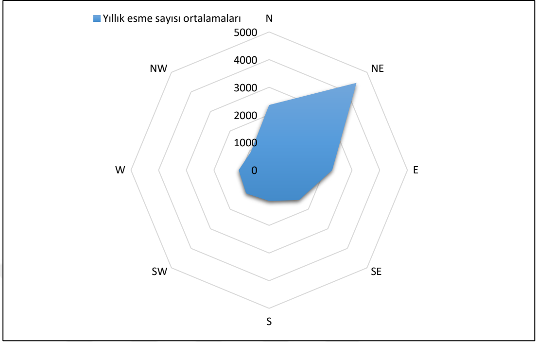
Grafik 4: Siverek'te Rüzgarların Yıllık Esme Sayısı Ortalamaları (1963-2015, Tablo 4'e göre)
