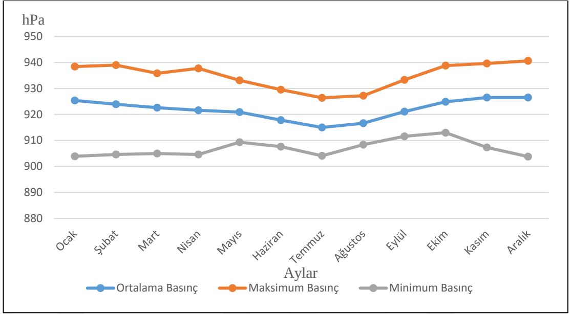
Grafik 3: Siverek'in Basınç Değerleri Grafiği (1963-2015)
