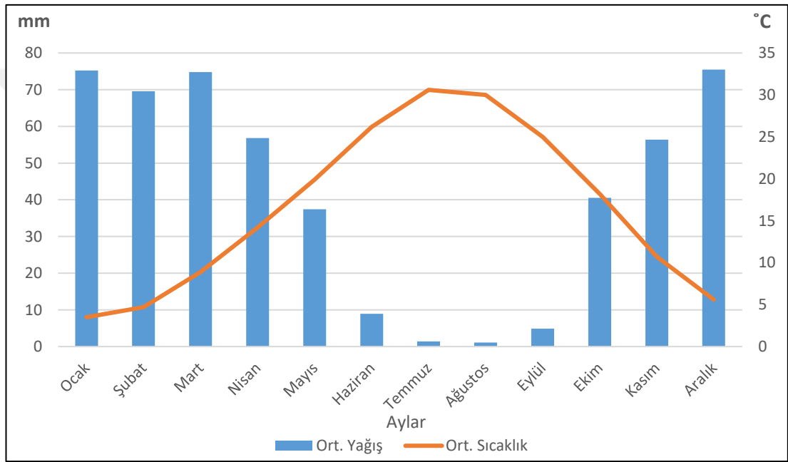
Grafik 7: Siverek’te Ortalama Yağış ve Sıcaklık Grafiği (1963-2015, Tablo 1 ve Tablo 9’a göre)
