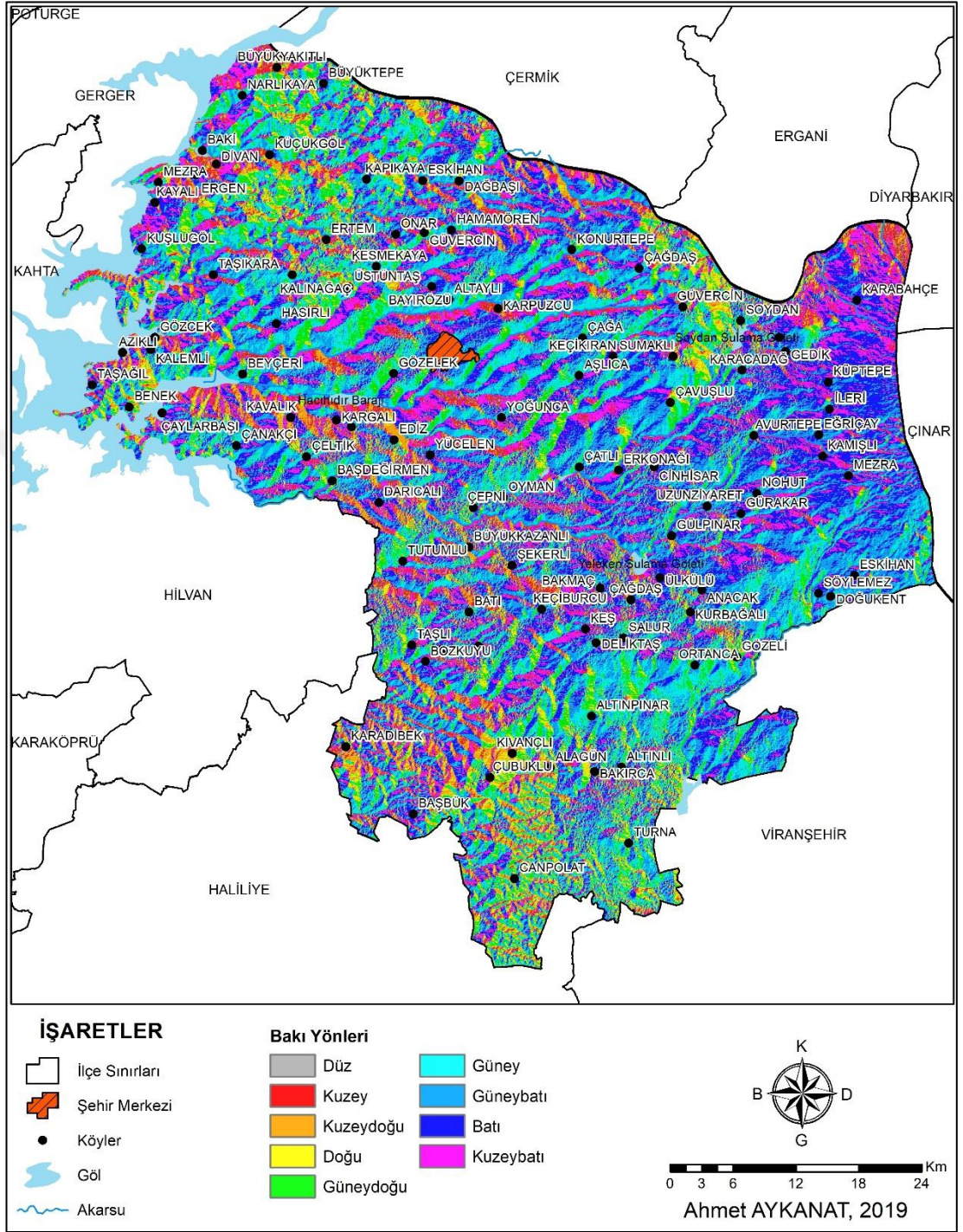
Harita 10: Çalışma Alanının Bakı Haritası
