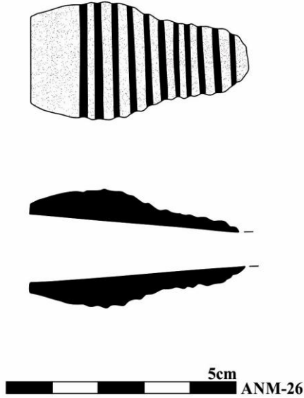
Çizim 7.42. Sol görünüm ve kesit çizimi
