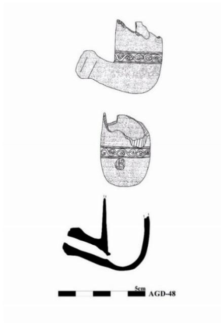
Çizim 7.32. Sağ görünüm, alt görünüm ve kesit çizimi
