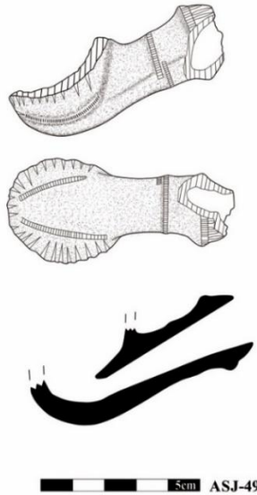
Çizim 7.24. Sol görünüm, alt görünüm ve kesit çizimi
