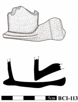
Çizim 7.50. Sol görünüm, alt görünüm ve kesit çizimi görünüm
