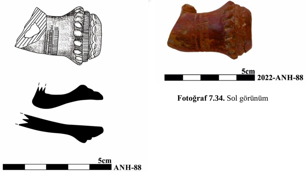
Çizim 7.40. Sol görünüm ve kesit çizimi
