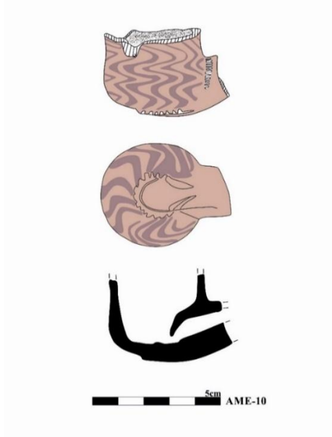
Çizim 7.21. Sol görünüm, alt görünüm ve kesit çizimi
