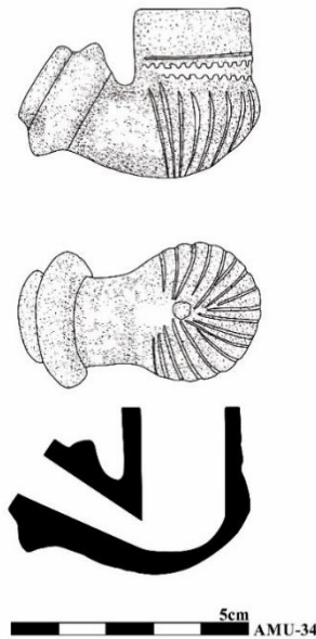
Çizim 7.6. Sol görünüm, alt görünüm ve kesit çizimi
