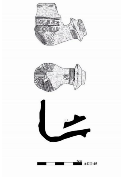
Çizim 7.31. Sol görünüm, Alt görünüm ve Kesit çizimi
