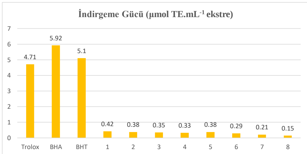
Şekil 4.3. Trolox, BHT, BHA standartları ile isot numunelerinin indirgenme gücü aktiviteleri
