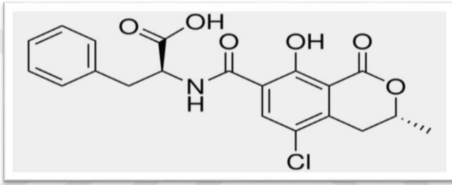
Şekil 2.5. Okratoksin bileşiğinin açık formül görseli
