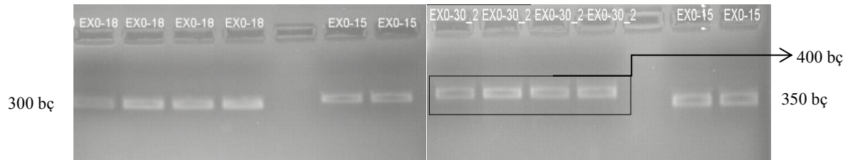
Şekil 4.2. KDR geninin ekzon 6, ekzon 7 ve ekzon 10 ampikonlarının agaroz jel görüntüsü.
