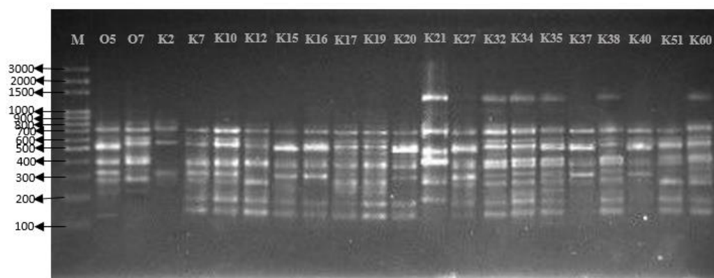
Figure 3.15. The amplification product of H. opuntiae using M13 primer. Lane M, 100-bp molecular marker; lane O5 (OA 4-CM NS2), H. opuntiae ; lane O7 (OA 4-CM NS4), H. opuntiae ; lane K2 (KA 0-CM NS2), H. opuntiae ; lane K7 (KB 0-CM NS2), H. opuntiae ; lane K10 (KB 0-CM NS5), H. opuntiae ; lane K12 (KA 4-CM NS2), H. opuntiae ; lane K15 (KA 4-CM NS5), H. opuntiae ; lane K16 (KB 4-CM NS1), H. opuntiae ; lane K17 (KB 4-CM NS2), H. opuntiae ; lane K19 (KB 4-CM NS4), H. opuntiae ; lane K20 (KB 4-CM NS5), H. opuntiae ; lane K21 (KA 2-NM NS1), H. opuntiae ; lane K27 (KB 2-NM NS4), H. opuntiae ; lane K32 (KA 4-NM NS4), H. opuntiae ; lane K34 (KA 4-NM NS8), H. opuntiae ; lane K35 (KA 4-NM NS10), H. opuntiae ; lane K37 (KB 4-NM NS3), H. opuntiae ; lane K38 (KB 4-NM NS5), H. opuntiae ; lane K40 (KB 4-NM NS9), H. opuntiae ; lane K51 (KA 2NM NS2), H. opuntiae ; lane K60 (KB 2-NM NS9), H. opuntiae .
