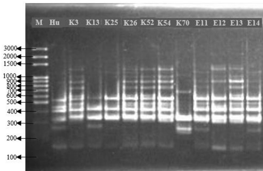
Figure 3.12. The amplification product of H. uvarum using (ATG) 5 primer Lane M, 100-bp molecular marker; lane Hu, reference strain H. uvarum (DSMZ); lane K3 (KA 0-CM NS3), H. uvarum ; lane K13 (KA 4-CM NS3), H. uvarum ; lane K25 (KA 2-NM NS9), H. uvarum ; lane K26 (KB 2-NM NS2), H. uvarum ; lane K52 (KA 2-NM NS4), H.
