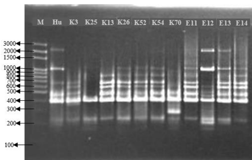
Figure 3.13. The amplification product of H. uvarum using (GTG) 5 primer. Lane M, 100-bp molecular marker; lane Hu, reference strain H. uvarum (DSMZ); lane K3 (KA 0-CM NS3), H. uvarum ; lane K25 (KA 2-NM NS9), H. uvarum ; lane K13 (KA 4-CM NS3), H. uvarum ; lane K26 (KB 2-NM NS2), H. uvarum ; lane K52 (KA 2-NM NS4), H. uvarum ; lane 54 (KA 2-NM NS8), H. uvarum ; lane K70 (KB 4-NM NS10), H. uvarum ; lane E11 (EA 1.W NS1), H. uvarum ; lane E12 (EA 1.W NS2), H. uvarum ; lane E13 (EA 1.W NS3), H. uvarum ; lane E14 (EA 1.W NS4), H. uvarum .
