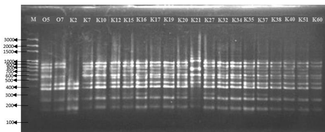
Figure 3.14. The amplification product of H. opuntiae using OPA-03 primer. Lane M, 100-bp molecular marker; lane O5 (OA 4-CM NS2), H. opuntiae ; lane O7 (OA 4-CM NS4), H. opuntiae ; lane K2 (KA 0-CM NS2), H. opuntiae ; lane K7 (KB 0-CM NS2), H. opuntiae ; lane K10 (KB 0-CM NS5), H. opuntiae ; lane K12 (KA 4-CM NS2), H. opuntiae ; lane K15 (KA 4-CM NS5), H. opuntiae ; lane K16 (KB 4-CM NS1), H. opuntiae ; lane K17 (KB 4-CM NS2), H. opuntiae ; lane K19 (KB 4-CM NS4), H. opuntiae ; lane K20 (KB 4-CM NS5), H. opuntiae ; lane K21 (KA 2-NM NS1), H. opuntiae ; lane K27 (KB 2-NM NS4), H. opuntiae ; lane K32 (KA 4-NM NS4), H. opuntiae ; lane K34 (KA 4-NM NS8), H. opuntiae ; lane K35 (KA 4-NM NS10), H. opuntiae ; lane K37 (KB 4-NM NS3), H. opuntiae ; lane K38 (KB 4-NM NS5), H. opuntiae ; lane K40 (KB 4-NM NS9), H. opuntiae ; lane K51 (KA 2NM NS2), H. opuntiae ; lane K60 (KB 2-NM NS9), H. opuntiae .
