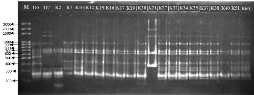
Figure 3.16. The amplification product of H. opuntiae using (ATG) 5 primer Lane M, 100-bp molecular marker; lane O5 (OA 4-CM NS2), H. opuntiae ; lane O7 (OA 4-CM NS4), H. opuntiae ; lane K2 (KA 0-CM NS2), H. opuntiae ; lane K7 (KB 0-CM NS2), H. opuntiae ; lane K10 (KB 0-CM NS5), H. opuntiae ; lane K12 (KA 4-CM NS2), H. opuntiae ; lane K15 (KA 4-CM NS5), H. opuntiae ; lane K16 (KB 4-CM NS1), H. opuntiae ; lane K17 (KB 4-CM NS2), H. opuntiae ; lane K19 (KB 4-CM NS4), H. opuntiae ; lane K20 (KB 4-CM NS5), H. opuntiae ; lane K21 (KA 2-NM NS1), H. opuntiae ; lane K27 (KB 2-NM NS4), H. opuntiae ; lane K32 (KA 4-NM NS4), H. opuntiae ; lane K34 (KA 4-NM NS8), H. opuntiae ; lane K35 (KA 4-NM NS10), H. opuntiae ; lane K37 (KB 4-NM NS3), H. opuntiae ; lane K38 (KB 4-NM NS5), H. opuntiae ; lane K40 (KB 4-NM NS9), H. opuntiae ; lane K51 (KA 2NM NS2), H. opuntiae ; lane K60 (KB 2-NM NS9), H. opuntiae
