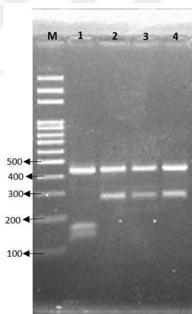
Figure 3.7. Gel image of PCR products cut with DraI restriction enzyme M, 100 bp marker; 1, H. guilliermondii K1 (KA 0CM NS1); 2, H. opuntiae K2 (KA 0CM NS2); 3, reference strain H. uvarum (DSMZ); 4, H. uvarum K13 (KA 4CM NS3)
