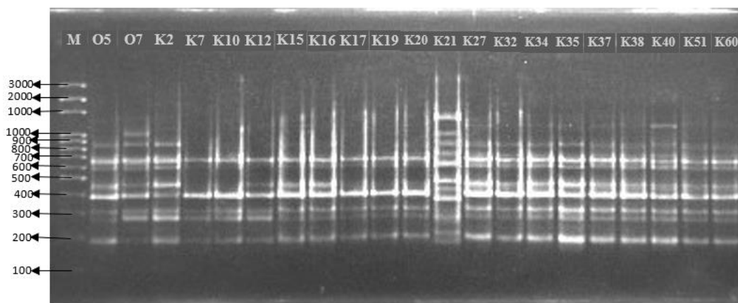
Figure 3.17. The amplification product of H. opuntiae using (GTG) 5 primer. Lane M, 100-bp molecular marker; lane O5 (OA 4-CM NS2), H. opuntiae ; lane O7 (OA 4-CM NS4), H. opuntiae ; lane K2 (KA 0-CM NS2), H. opuntiae ; lane K7 (KB 0-CM NS2), H. opuntiae ; lane K10 (KB 0-CM NS5), H. opuntiae ; lane K12 (KA 4-CM NS2), H. opuntiae ; lane K15 (KA 4-CM NS5), H. opuntiae ; lane K16 (KB 4-CM NS1), H. opuntiae ; lane K17 (KB 4-CM NS2), H. opuntiae ; lane K19 (KB 4-CM NS4), H. opuntiae ; lane K20 (KB 4-CM NS5), H. opuntiae ; lane K21 (KA 2-NM NS1), H. opuntiae ; lane K27 (KB 2-NM NS4), H. opuntiae ; lane K32 (KA 4-NM NS4), H. opuntiae ; lane K34 (KA 4-NM NS8), H. opuntiae ; lane K35 (KA 4-NM NS10), H. opuntiae ; lane K37 (KB 4-NM NS3), H. opuntiae ; lane K38 (KB 4-NM NS5), H. opuntiae ; lane K40 (KB 4-NM NS9), H. opuntiae ; lane K51 (KA 2NM NS2), H. opuntiae ; lane K60 (KB 2-NM NS9), H. opuntiae .
