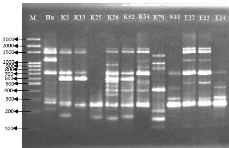
Figure 3.10. The amplification product of H. uvarum using primer OPA-03 Lane M, 100-bp molecular marker; lane Hu, reference strain H. uvarum (DSMZ); lane K3 (KA 0-CM NS3), H. uvarum ; lane K13 (KA 4-CM NS3), H. uvarum ; lane K25 (KA 2-NM NS9), H. uvarum ; lane K26 (KB 2-NM NS2), H. uvarum ; lane K52 (KA 2-NM NS4), H. uvarum ; lane 54 (KA 2-NM NS8), H. uvarum ; lane K70 (KB 4-NM NS10), H. uvarum ; lane E11 (EA 1.W NS1), H. uvarum , lane E12 (EA 1.W NS2), H. uvarum ; lane E13 (EA 1.W NS3), H. uvarum ; lane E14 (EA 1.W NS4), H. uvarum
