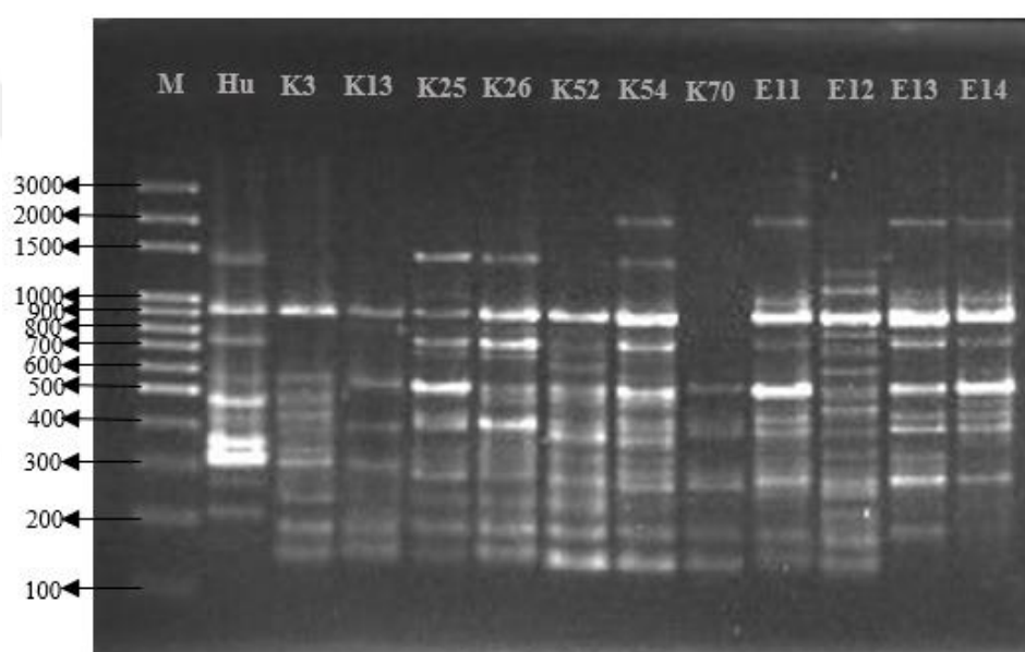
Figure 3.11. The amplification product of H. uvarum using M13 primer. Lane M, 100-bp molecular marker; lane Hu, reference strain H. uvarum (DSMZ); lane K3 (KA 0-CM NS3), H. uvarum ; lane K13 (KA 4-CM NS3), H. uvarum ; lane K25 (KA 2-NM NS9), H. uvarum ; lane K26 (KB 2-NM NS2), H. uvarum ; lane K52 (KA 2-NM NS4), H. uvarum ; lane 54 (KA 2-NM NS8), H. uvarum ; lane K70 (KB 4-NM NS10), H. uvarum ; lane E11 (EA 1.W NS1), H. uvarum ; lane E12 (EA 1.W NS2), H. uvarum ; lane E13 (EA 1.W NS3), H. uvarum ; lane E14 (EA 1.W NS4), H. uvarum .
