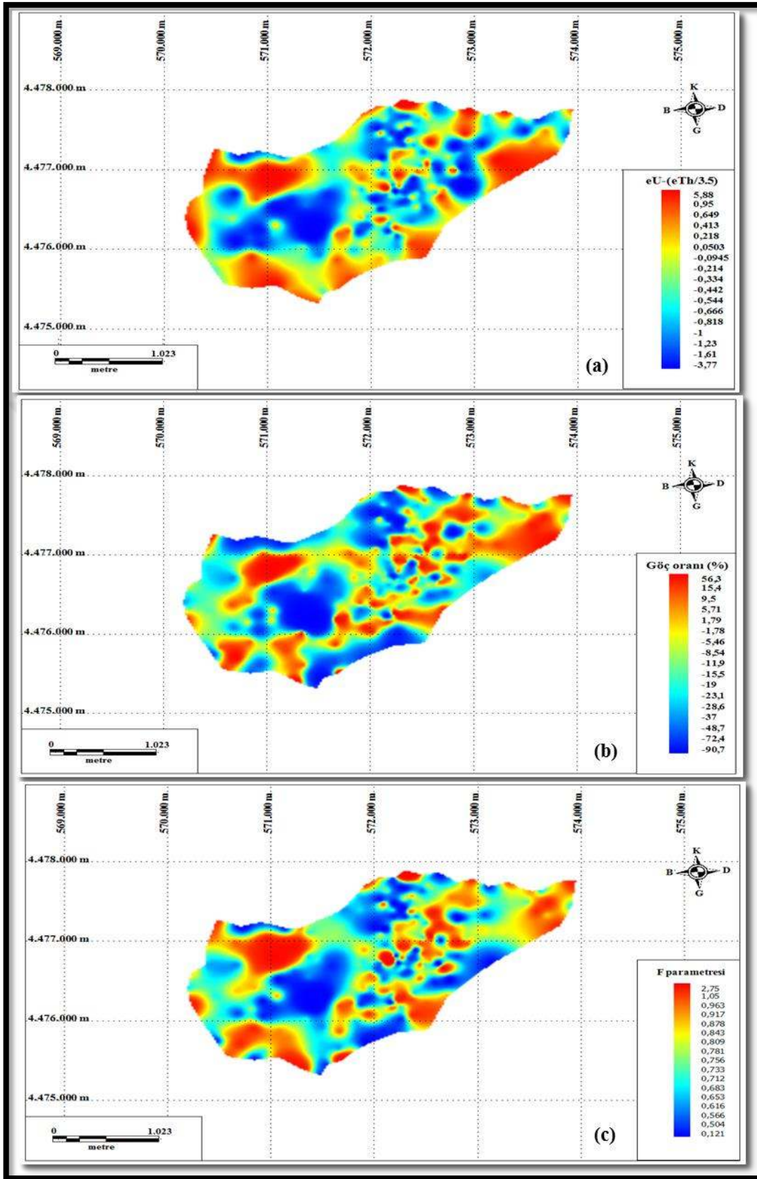
Şekil 4.6. Sarıçiçek granodiyoriti (Gümüşhane) ve çevresinde a) U değişim oranı, b) Göç oranı c) F parametresi dağılımı
