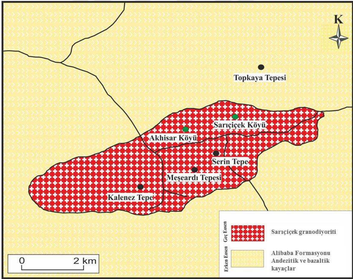
Şekil 2.10. Sarıççek granodiyoriti ve çevresinin yüzeylendiği alanının 1/25.000 ölçekli jeoloji haritası (Karşı, 2002).
