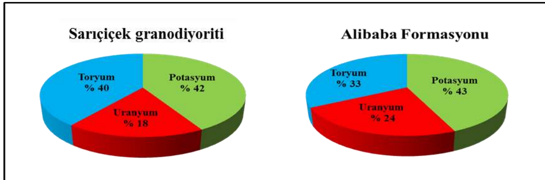
Şekil 5.2. Sarıçiçek granodiyoriti ve çevresi (Gümüşhane) için toplam absorbe edilen doza ^{232}\text{Th} , ^{238}\text{U} ve ^{40}\text{K} ' in katkıları
