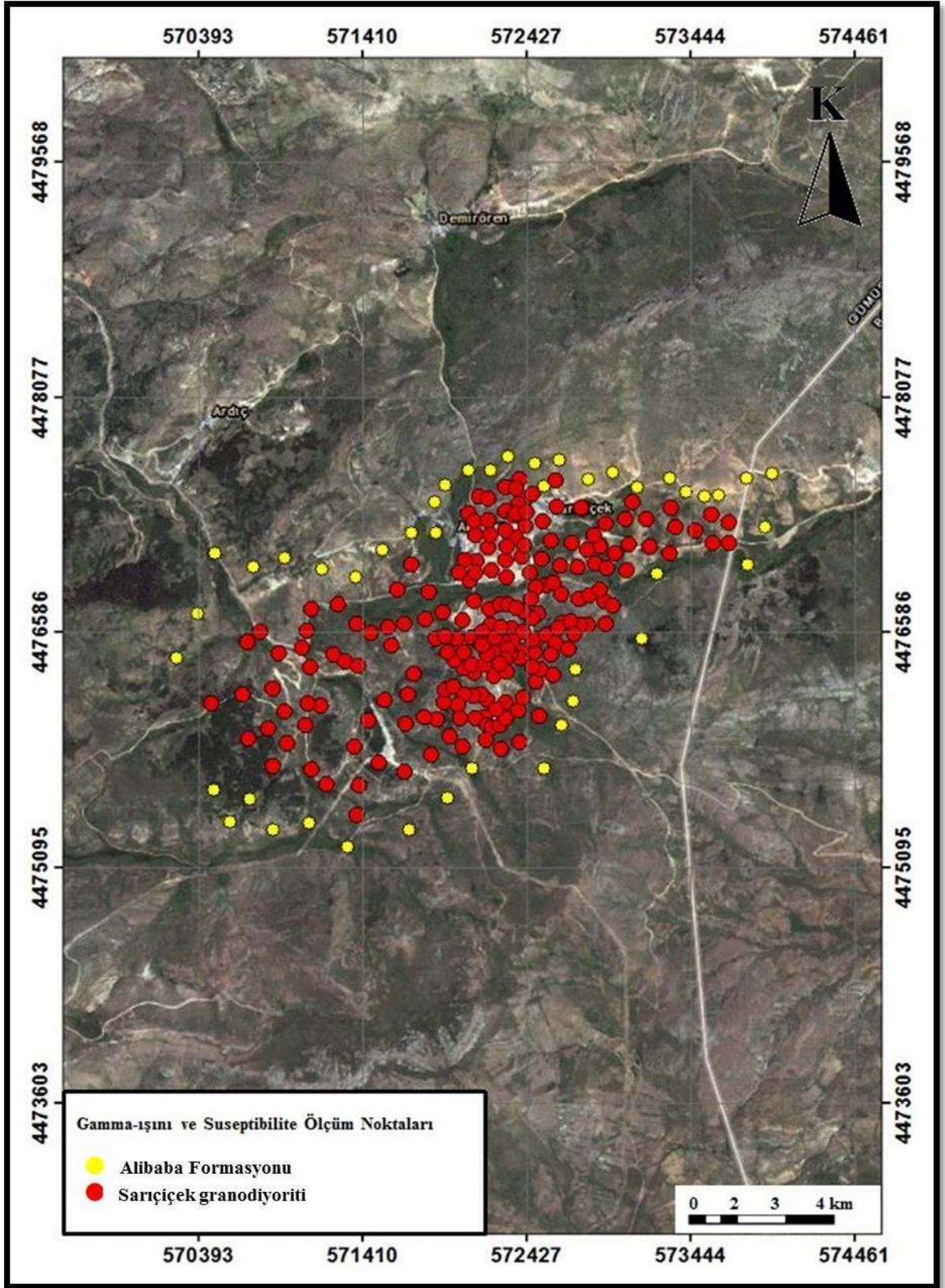
Şekil 4.1. Sarıççek granodioriti ve çevresinde alınan yerinde gama-ışını ve manyetik suseptibilite ölçüm noktalarının konumları
