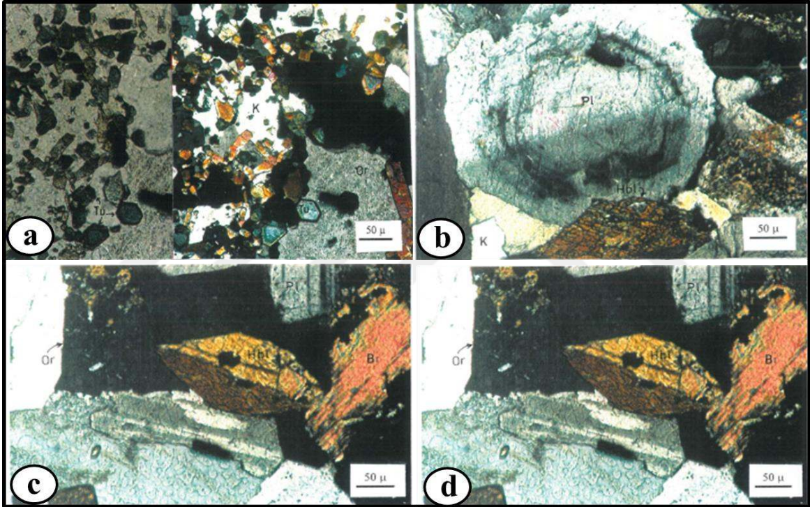
Şekil 2.9. Sarıhan granodiyoritinde bulunan (a) Özşekli turmalinler. Tu: Turmalin, Or: Ortoklas, K: Kuvars (b) Halkalı zonlu plajiyoklas. Pl: Plajiyoklas, Hbl: Hornblend (c) Hornblendlere ait h' (100) ikizi. Bi: Biotit, Or: Ortoklas (d) Granodiyoritteki biyotit kristali Bi: Biotit (Arslan, 1998).
