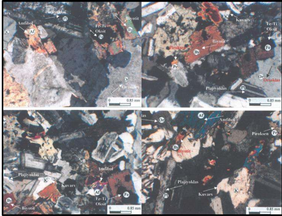
Şekil 2.12. Sarıçiçek granodiyoritindeki kayaçların dokusal görünümleri (Or: Ortoklas, Pl: Plajiyoklas, K: Kuvars, Af: Amfibol, By: Biyotit, Fe: Fe-Ti oksit) (Karşı, 2002).
