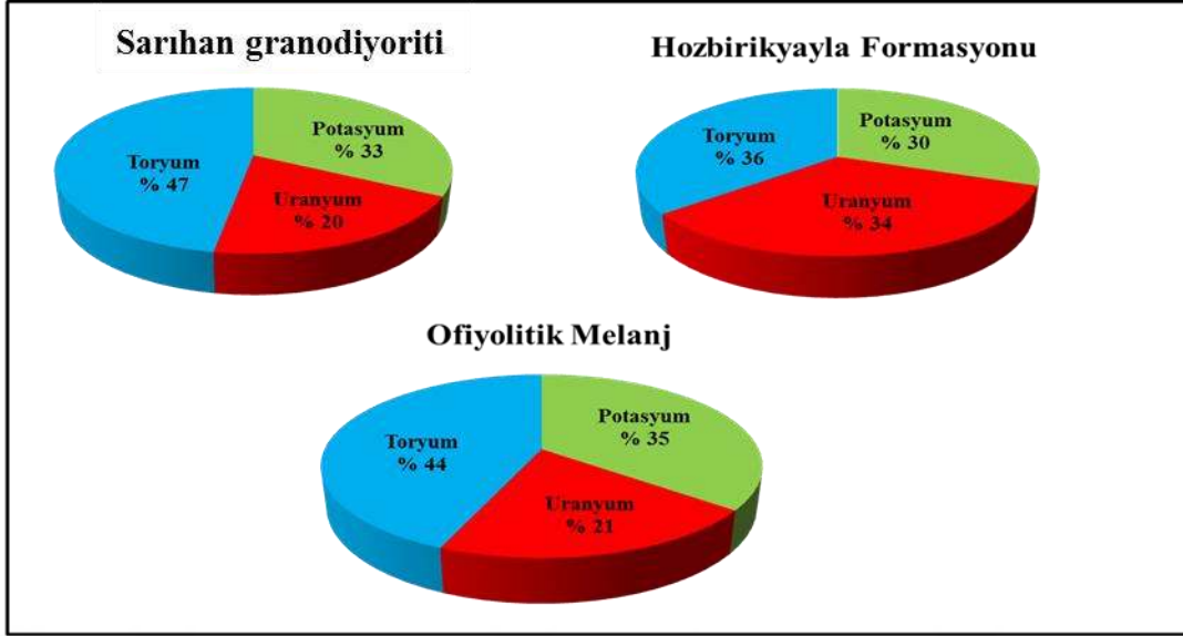
Şekil 5.9. Sarıhan granodioriti ve çevresi (Bayburt) için toplam absorbe edilen doza Th, U ve K'nın katkıları.
