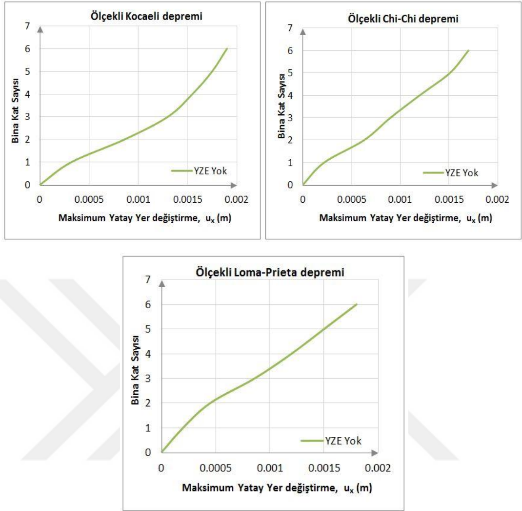
Şekil 3.10. Üç farklı deprem etkisindeki model yapının yükseklięi boyunca kat yatay yerdeęiřtirmeleri
