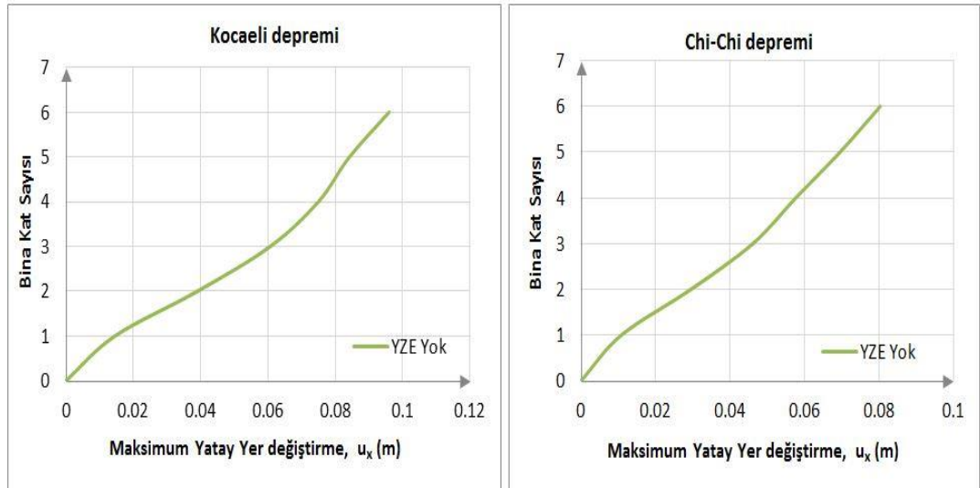
Şekil 3.8. Üç farklı deprem etkisinde gerçek yapının yüksekliği boyunca kat yatay yer değiştirmeleri
