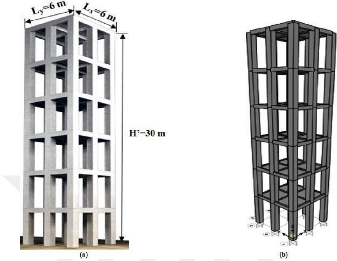
Şekil 3.7. (a) Gerçek yapının görüntüsü (b) Gerçek yapının sonlu elemanlar dayalı matematik modeli
