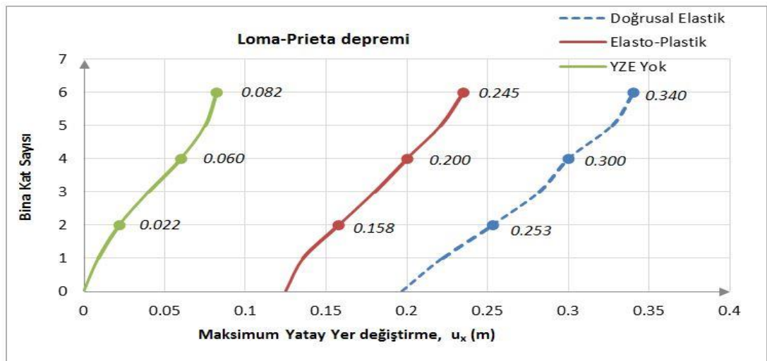
řekil 3.14. Loma-Prieta depremi etkisindeki gerek sistemde binanın ykseklięi boyunca kat ya yer deęiřtirmeleri
