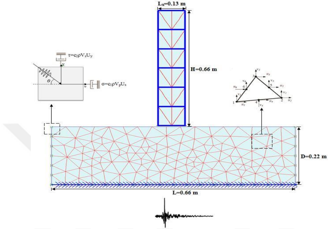
Şekil 3.15. Yapı-zemin etkileşim problemi için geliştirilen ölçekli sonlu eleman modeli
