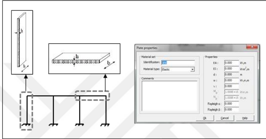
Şekil 2.4. Rijit eleman ve girdi parameterleri [24]
