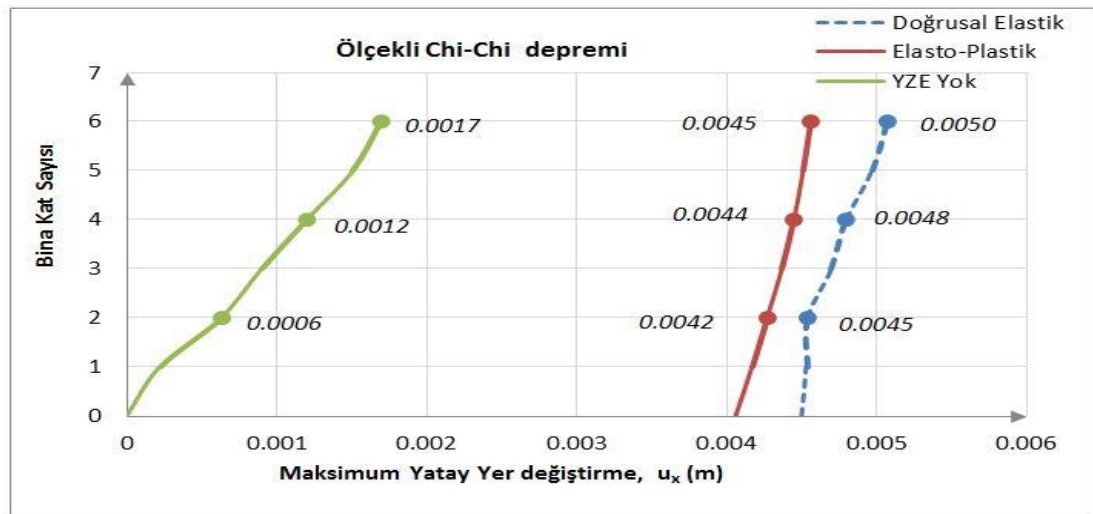
Şekil 3.17. Chi-Chi depremi etkisindeki modelde binanın yüksekliği boyunca kat yatay yer değiştirmeleri
