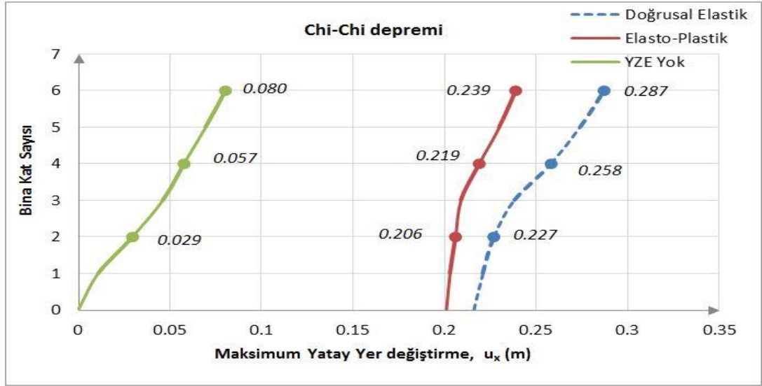
řekil 3.13. Chi-Chi depremi etkisindeki gerek sistemde binanın ykseklięi boyunca kat yatay yer deęiřtirmelerini
