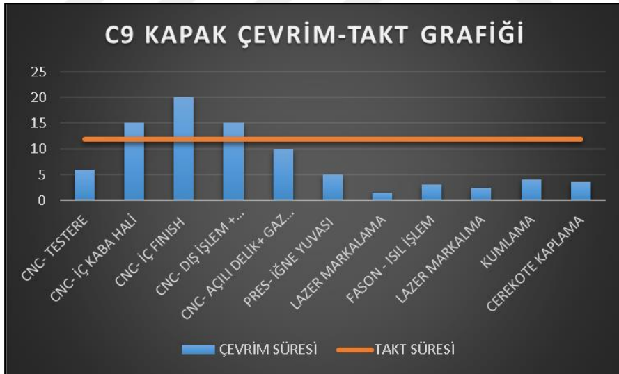
Şekil 4.8. Mevcut durum çevrim süresi grafiği(kapak).
