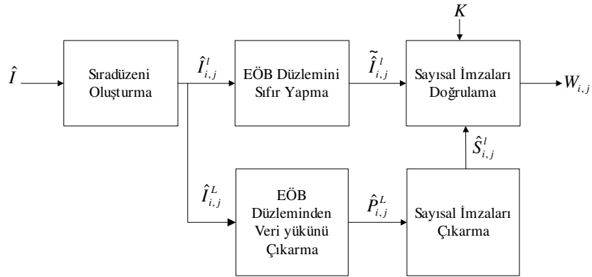
Şekil 4.15. Sıradüzensel Filigranlama Tekniğinin doğrulama yordamı
