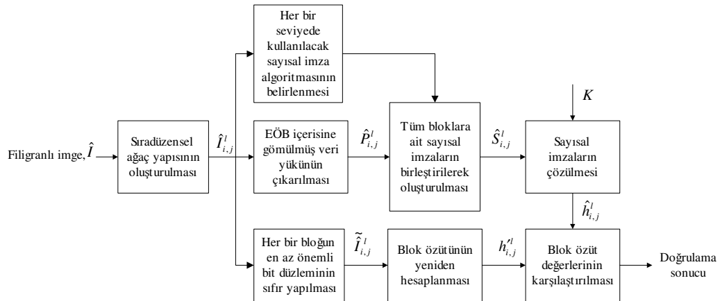
Şekil 5.4. Sıradüzensel Ağaç Yapılı Kırılğan Filigranlama Tekniği'nin doğrulama yordamı
