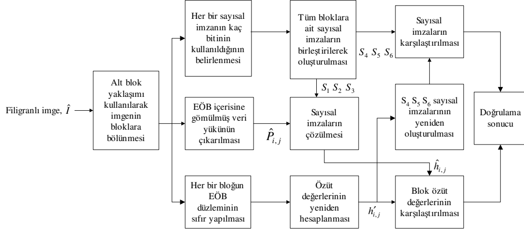
Şekil 6.5. Alt Blok Yaklaşımlı Kırılgan Filigranlama Tekniğinin doğrulama yordamı
