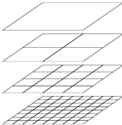
Şekil 4.14. Sıradüzensel 4 seviyeli blok yapısı
