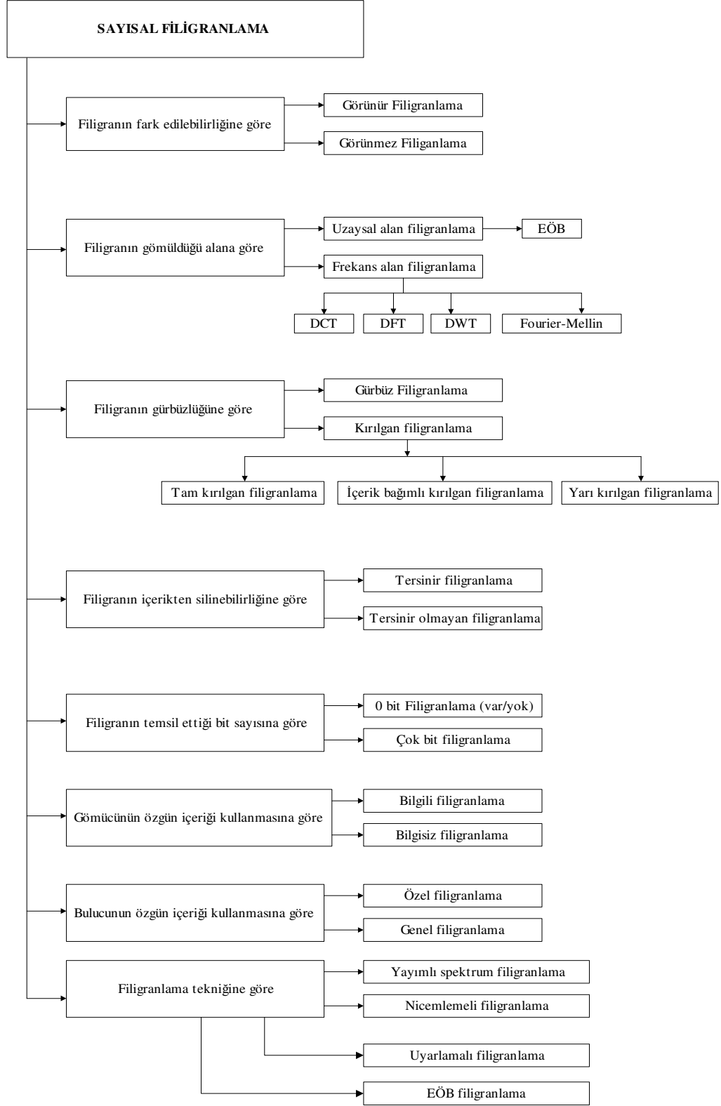
Şekil 3.12. Sayısal Filigranlama Sistemleri'nin sınıflandırılması
