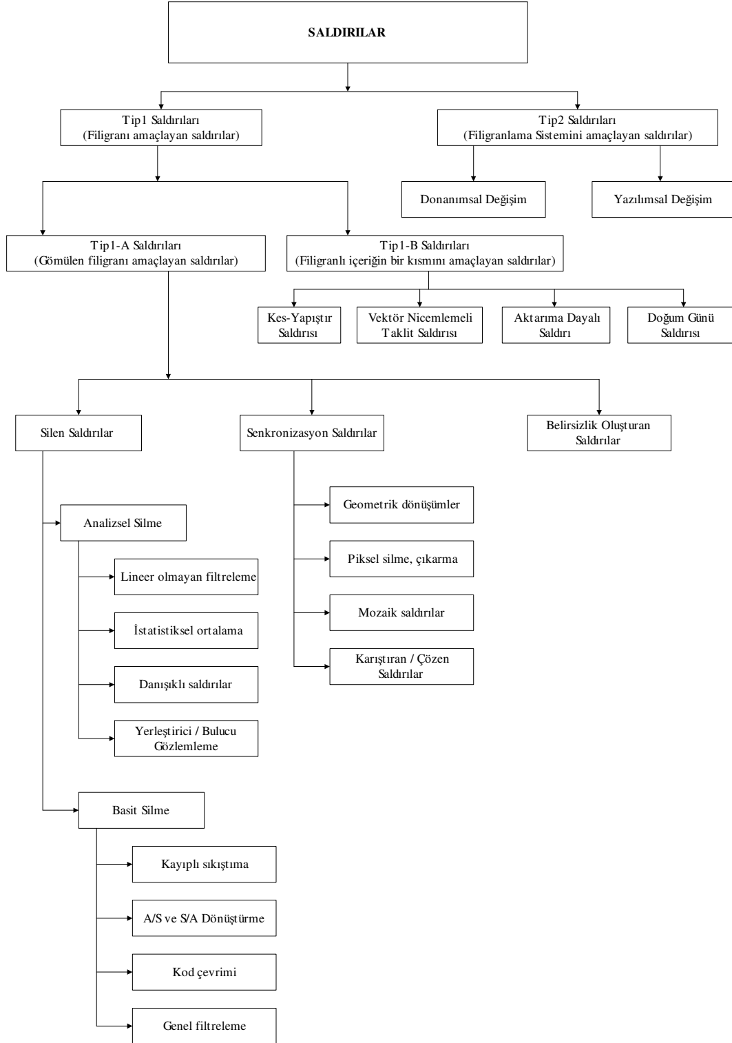
Şekil 3.15. Saldırıların sınıflandırılması
