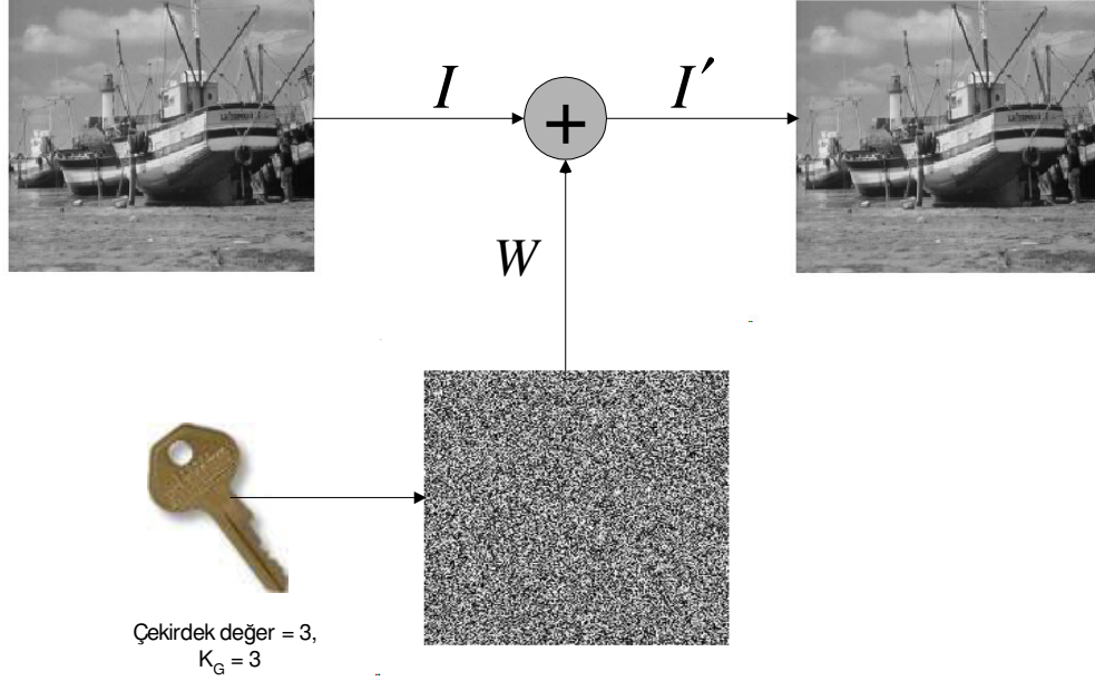
Şekil 3.10. Filigranın gömülmesi
