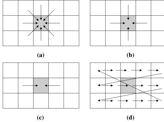
Şekil 4.10. Blok bağımlılıkları (a) 8 bağımlılık (b) 4 bağımlılık (c) 2 bağımlılık (d) 1 bağımlılık
