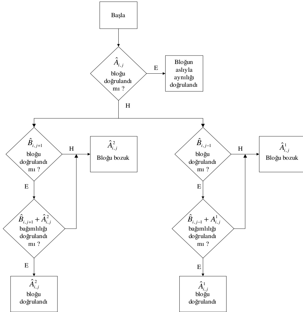
Şekil 6.6. Alt blokların doğrulanması için kullanılan algoritma
