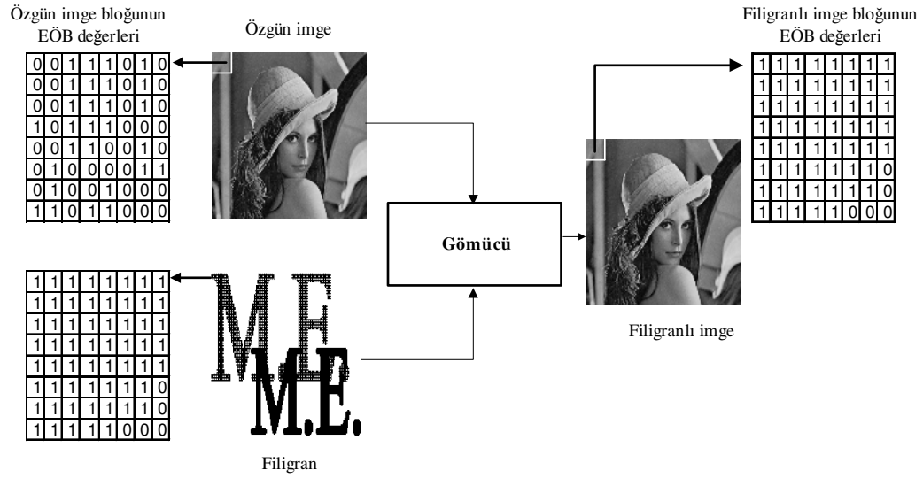
Şekil 3.8. İkili bir imgesel filigranın imgenin EÖB düzlemine gömülmesi
