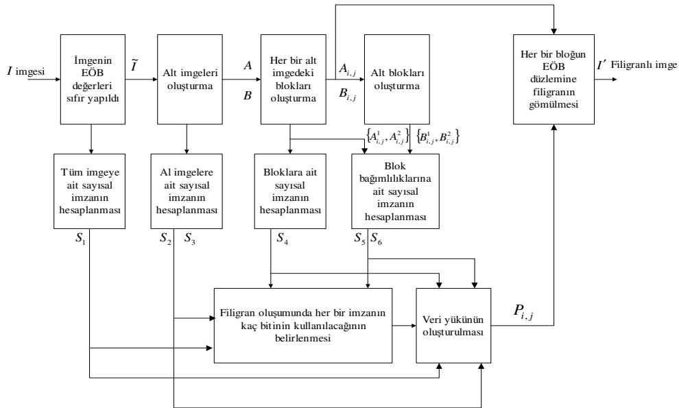
Şekil 6.1. Alt blok yaklaşımıyla kırılğan filigranlama tekniğinin filigranlama yordamı
