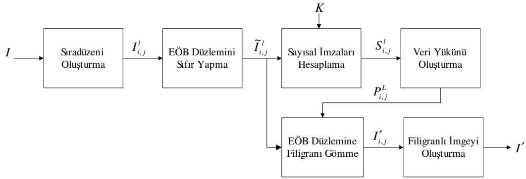
Şekil 4.13. Sıradüzensel Filigranlama Tekniğinin filigranlama yordamı
