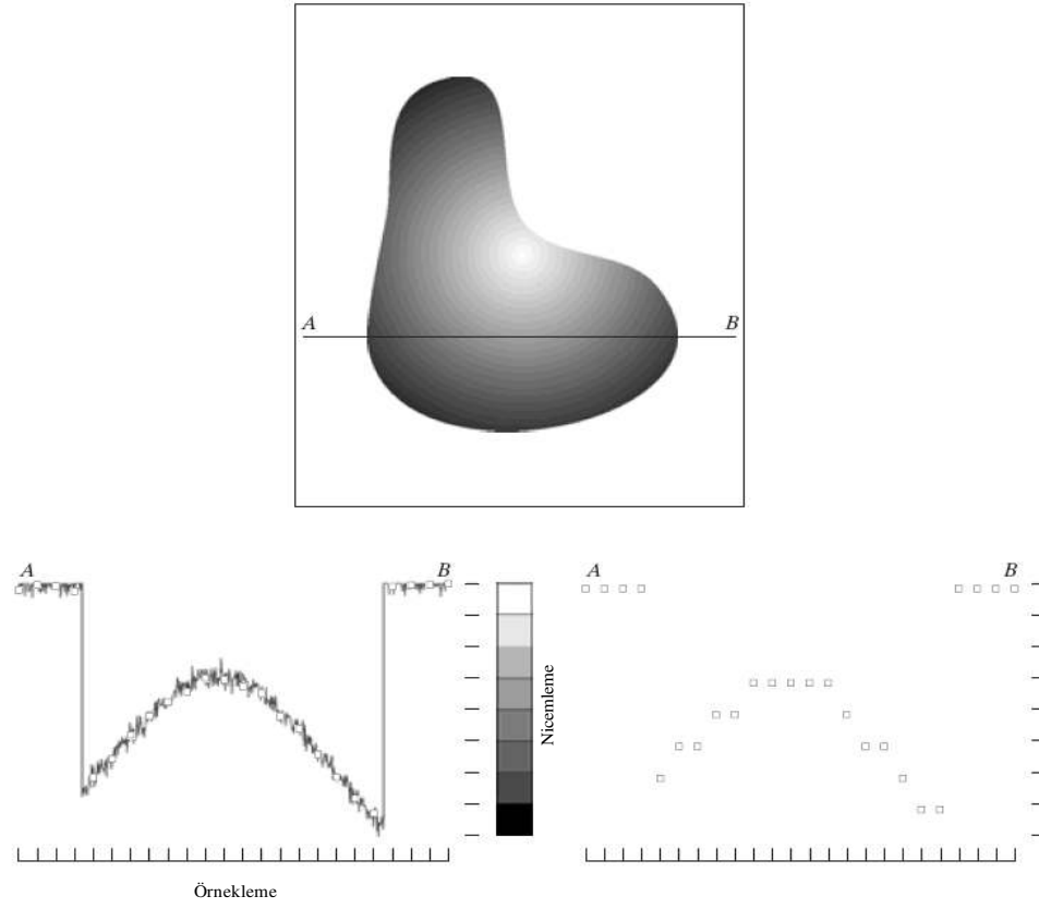
Şekil 3.3. İmgenin sayısallaştırılması
