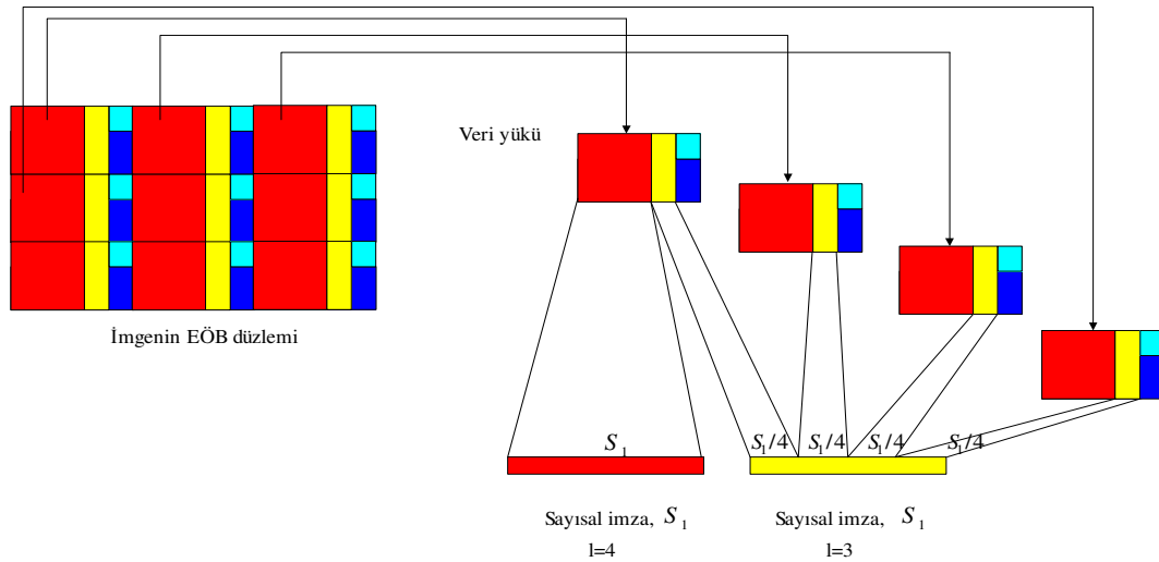
Şekil 5.5. Sıradüzensel ağaç yapısındaki 4. ve 3. seviyedeki blok imzalarının birleştirilerek oluşturulması
