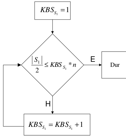
Şekil 6.3. Her blok içerisinde S_1 sayısal imzasının kaç bitinin gömüleceğinin belirlenmesi
