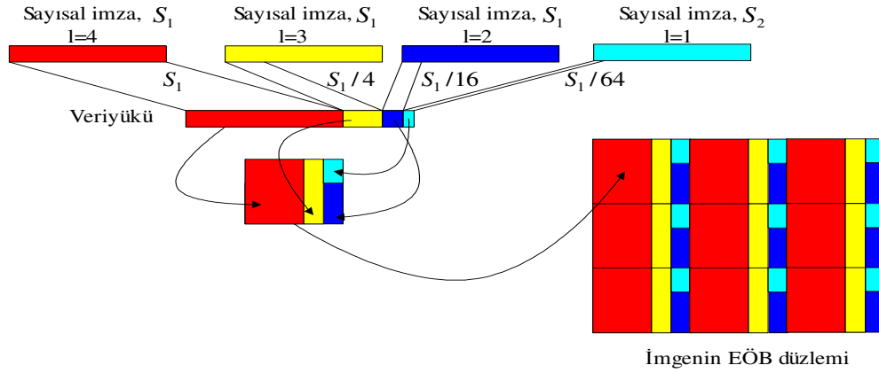
Şekil 5.3. 4 seviyeli sıradüzensel ağaç yapısında sayısal imzaların birleştirilmesiyle oluşturulan veri yükü
