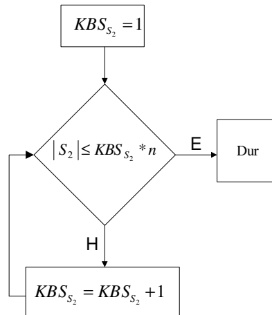
Şekil 6.4. Her blok içerisinde S_2 ve S_3 sayısal imzasının kaç bitinin gömüleceğinin belirlenmesi
