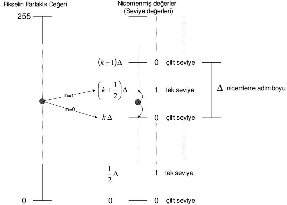
Şekil 3.9. Nicemlemeli gömme
