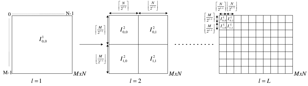
Şekil 5.2. Sıradüzensel ağaç yapısı kullanılarak imgenin bloklara bölünmesi
