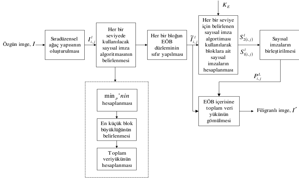
Şekil 5.1. Sıradüzensel Ağaç Yapılı Kırılğan Filigranlama Tekniği'nin filigranlama yordamı
