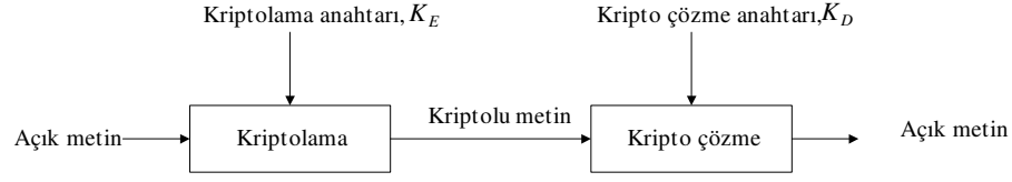
Şekil 4.3. Asimetrik anahtarlı kriptografi
