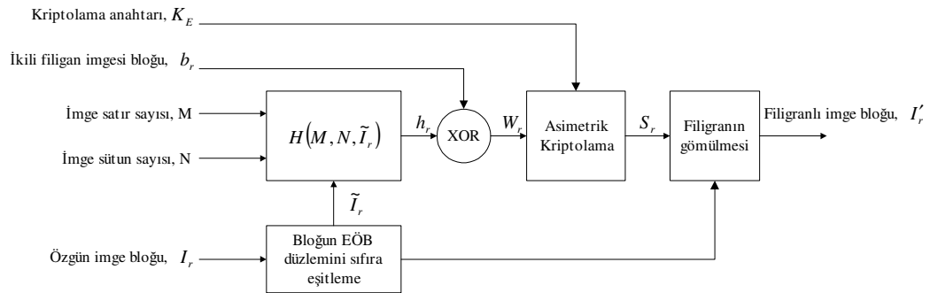
Şekil 4.5. Wong'un tekniğinin filigranlama yordamı
