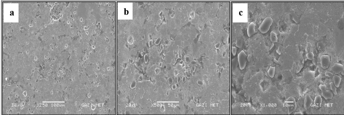
Şekil 3.18. Alumix-231+%10 B_4C 'ünSEM görüntüsü; a) x250 b) x500 c) x1000
