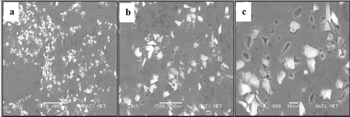
Şekil 3.17. Alumix-231+%10 Al_2O_3 'in SEM görüntüsü; a) x250 b) x500 c) x1000
