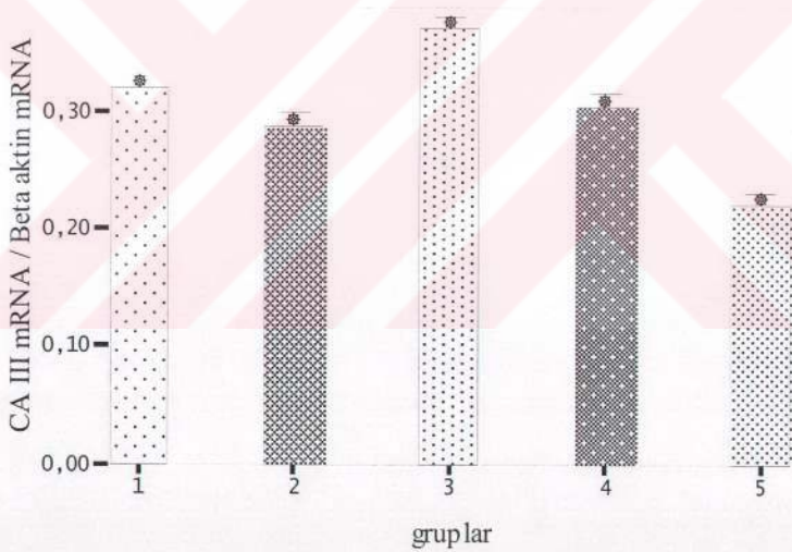
Şekil 12. Deney gruplarındaki ortalama CA III mRNA/ \beta -aktin mRNA oranları.1: bazal grup, 2:leptin grubu, 3:insulin grubu, 4:deksametazon grubu, 5:ins+lep grubu.
