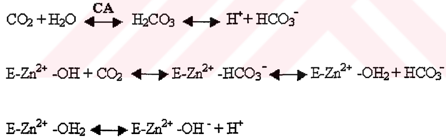
Şekil 1. Karbonik anhidraz tarafından katalizlenen \text{CO}_2 hidrasyonu reaksiyonunun mekanizması
