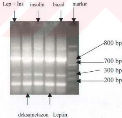
Şekil 10. Agarozelektroforezi fotoğrafı
