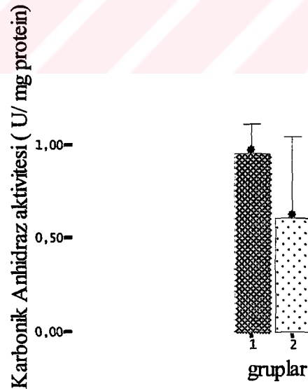
Şekil 9. Deney gruplarındaki ortalama karbonik anhidraz aktiviteri.
