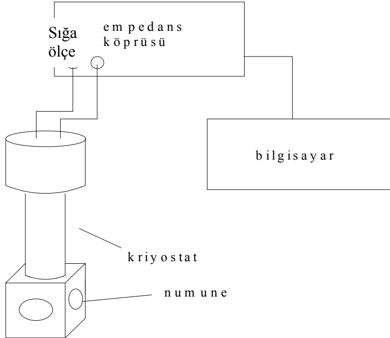
Şekil 3.6 Kapasite-gerilim ölçümleri için kullanılan düzenek
