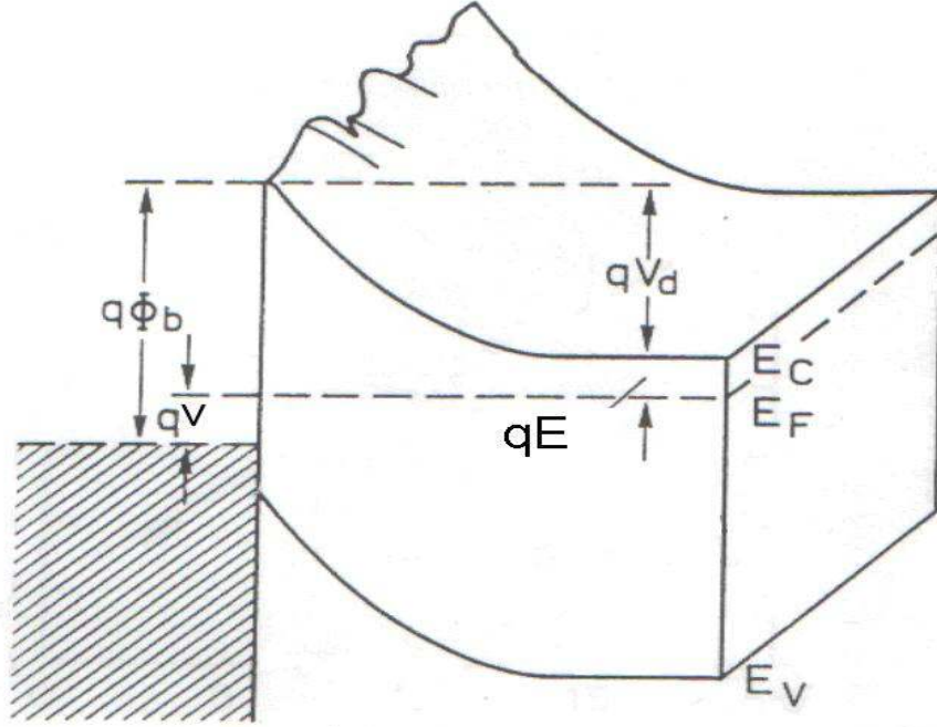
Şekil 4.9. Homojen olmayan bir Schottky kontağın iki boyutlu bant diyagramı V_d bant bükülmesi, \Phi_b Schottky engel yüksekliğidir
