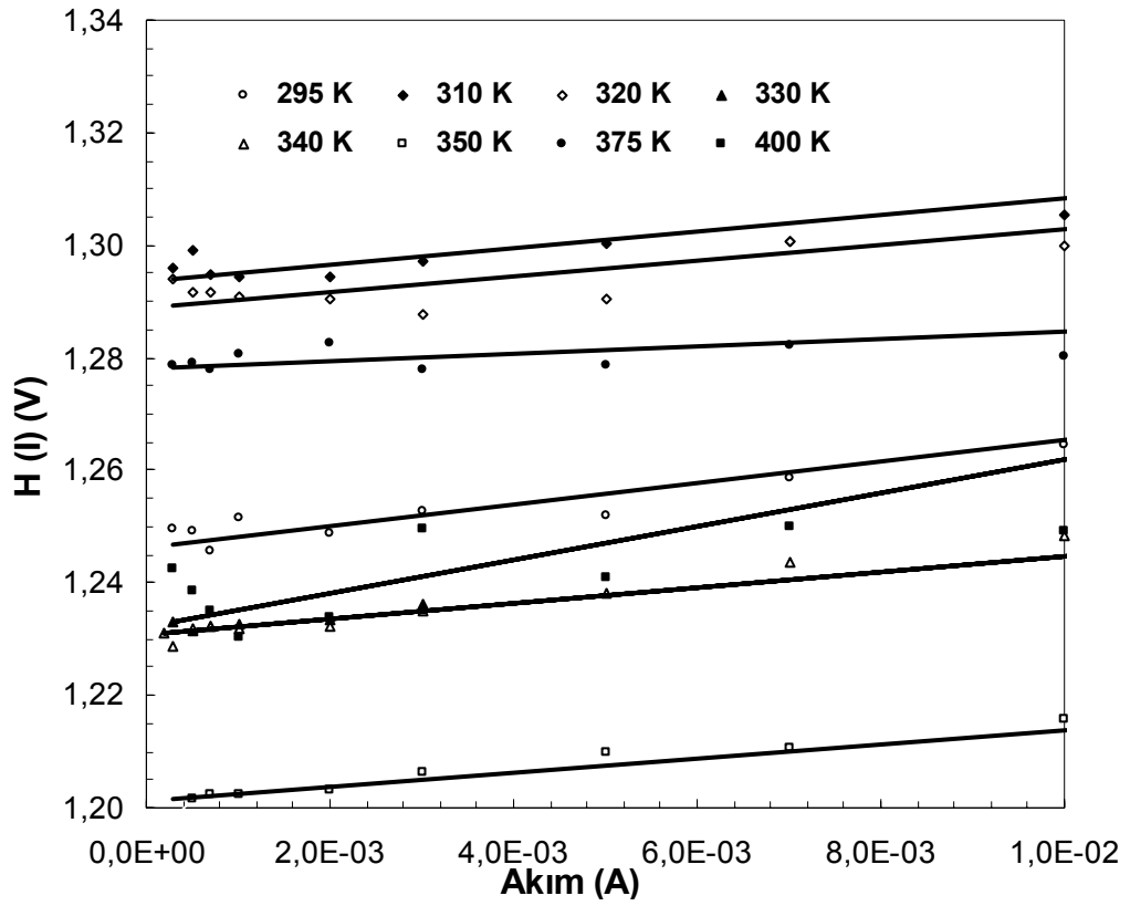
Şekil 4.12. Al/SiO_2/p-Si (MIS) Schottky diyotunun farklı sıcaklıklardaki [H(I)-I] grafiği
