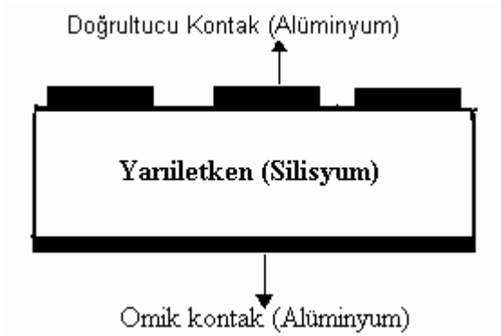
Şekil 2.1. Bir Schottky kontakın şematik görünümü
