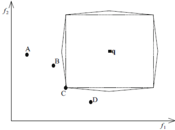
Şekil 5.10. Uzatılmış Chebyshev metriğinin tam sayılı programlama gösterimi
