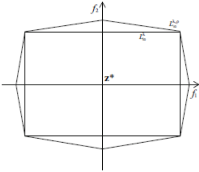
Şekil 5.5. L_\infty^\lambda ve L_\infty^{\lambda,p} metriklerine göre z^* 'dan eşit uzaklıktaki noktaların gösterimi
