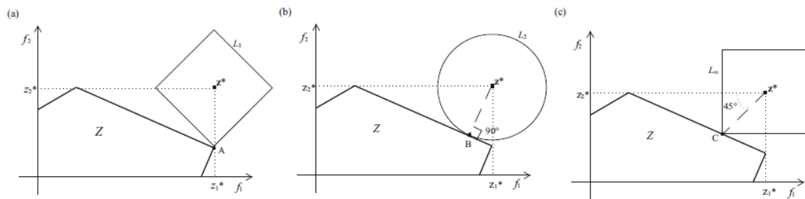
Şekil 5.3. L_1 , L_2 ve L_\infty metriklerine göre Z bölgesinin z^* 'a en yakın noktalarının gösterimi
