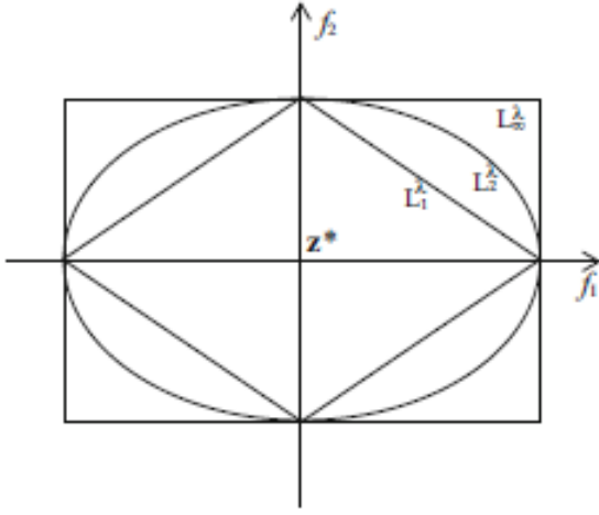
Şekil 5.4. L_1^\lambda , L_2^\lambda ve L_\infty^\lambda metrikleri için z^* 'a aynı uzaklıktaki noktaların gösterimi
