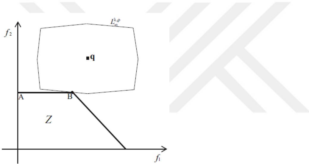
Şekil 5.8. Referans noktaya uzatılmış ağırlıklı Chebyshev uzaklığının en küçüklenmesi
