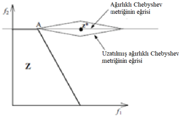
Şekil 5.7. Ağırlıklı Chebyshev ve uzatılmış ağırlıklı Chebyshev uzaklığının gösterimi
