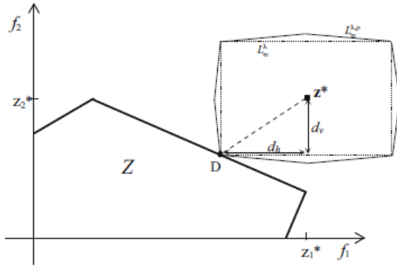
Şekil 5.6. Uzatılmış ağırlıklı Chebyshev uzaklığının en küçüklenmesi
