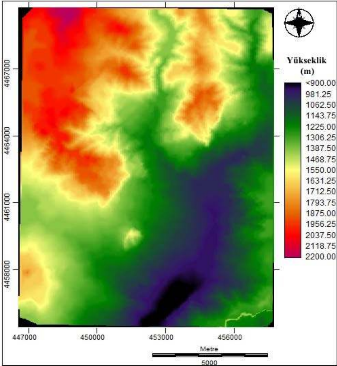
Şekil 7.2. İnceleme alanına ait Sayısal Yükseklik Modeli
