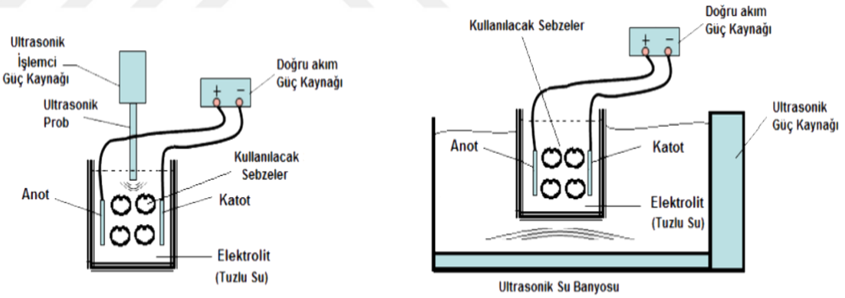
(a) Ultrasonik İşlemci + Elektrik Akımı Uygulaması
