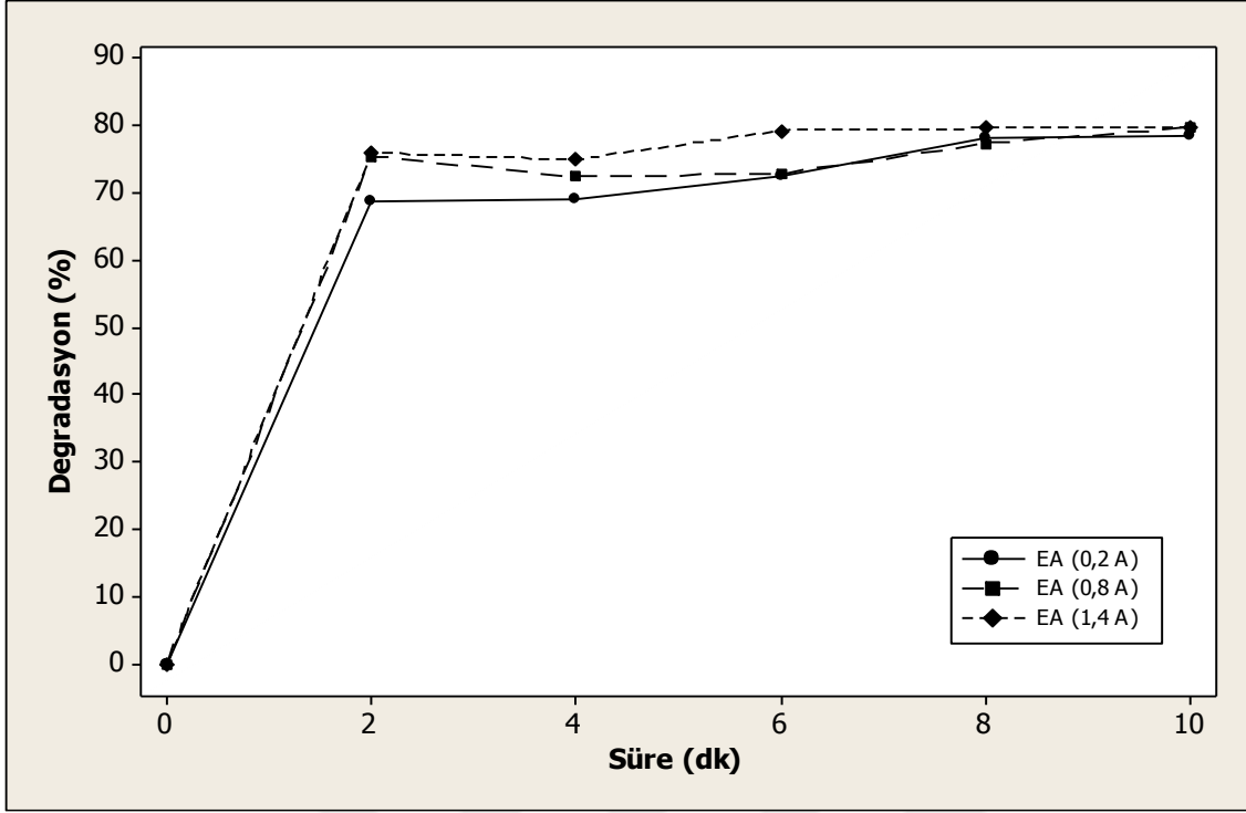
Şekil 4.22. Domates numunelerinde elektrik akımı uygulamaları ile elde edilen metalaxyl degradasyon oranları (%) (EA:Elektrik Akımı)
