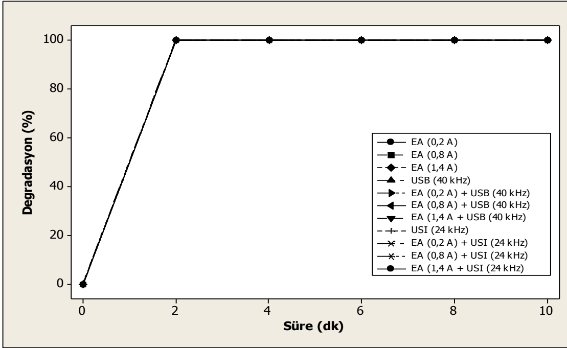
Şekil 4.6. Düşük konsantrasyon model sistemde (57,14 ppb) gerçekleştirilen deneyler ile elde edilen captan degradasyon oranları (%) (EA: Elektrik Akımı, USB: Ultrasonik Su Banyosu, USI: Ultrasonik İşlemci)
