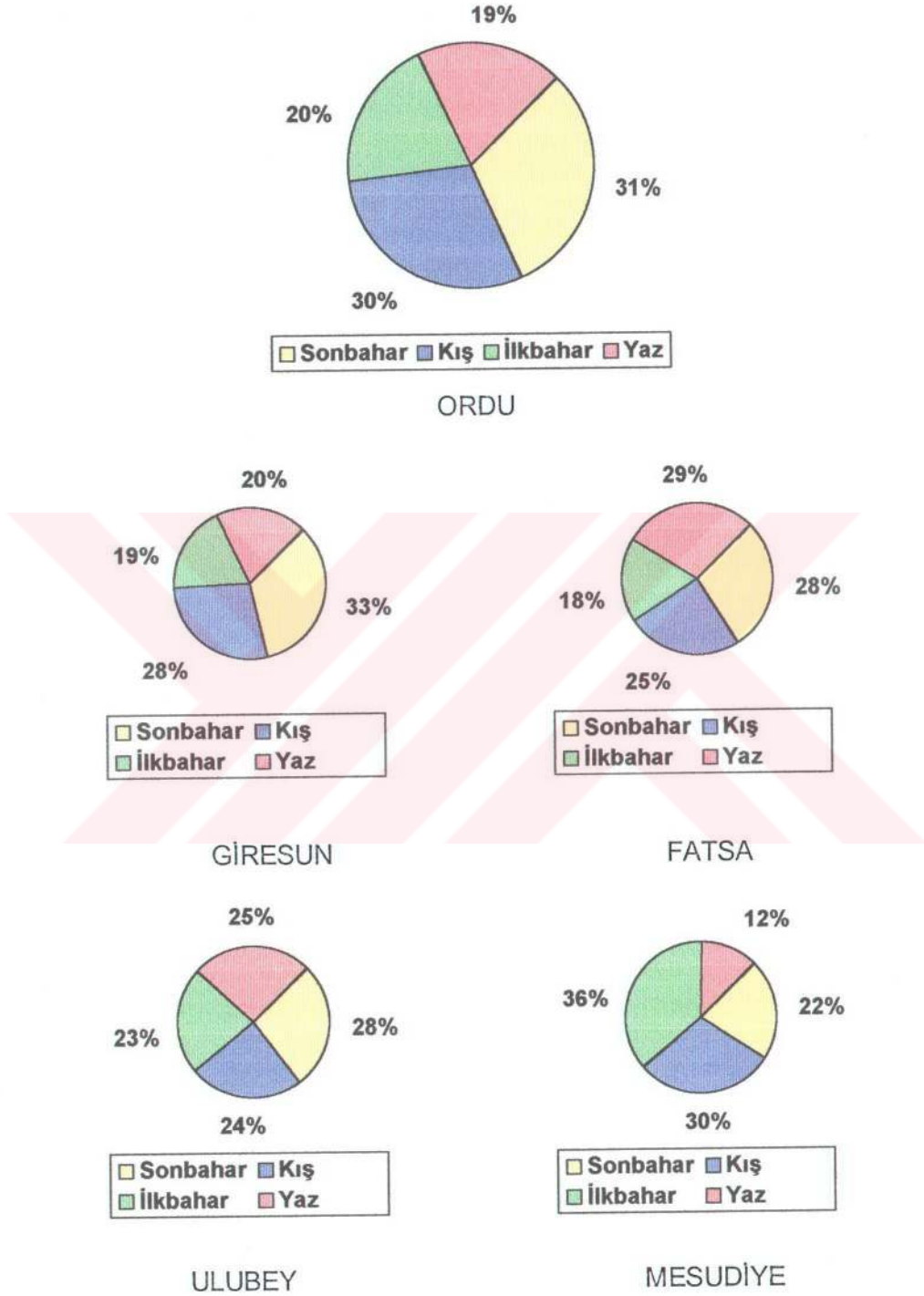
Grafik 4 : Ordu Şehri ve Çevre İstasyonlarda Yağış Miktarının Mevsimlere Göre Dağılışı.
