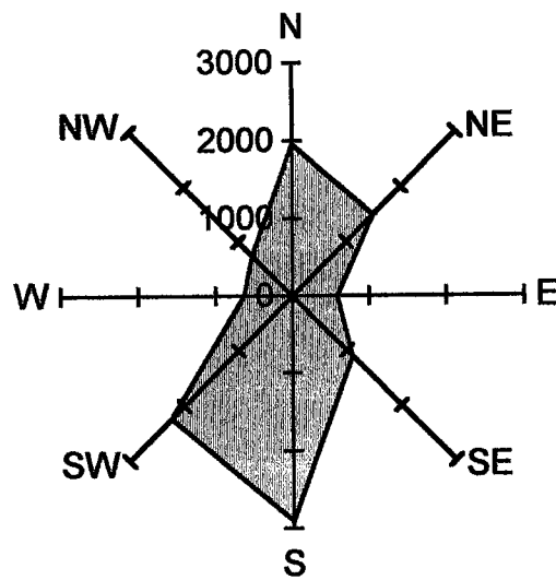
Grafik 2 : Ordu Şehri Rüzgar Gücü Diyagramı (1966-1990).
