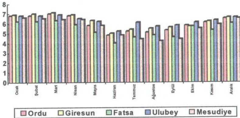
Grafik 6 : Ordu Şehri ve Çevre İstasyonlarda Ortalama Bulutluluk.
