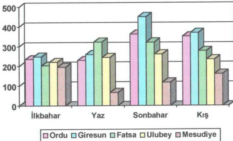
Grafik 3 : Ordu Şehri ve Çevre İstasyonlarda Yağış Miktarının Mevsimlere Göre Dağılışı.
