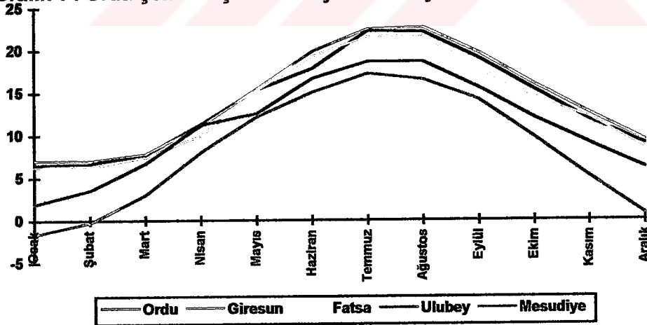
Grafik 1 : Ordu Şehri ve Çevre İstasyonlarda Aylık Ortalama Sıcaklık Diyagramı.
