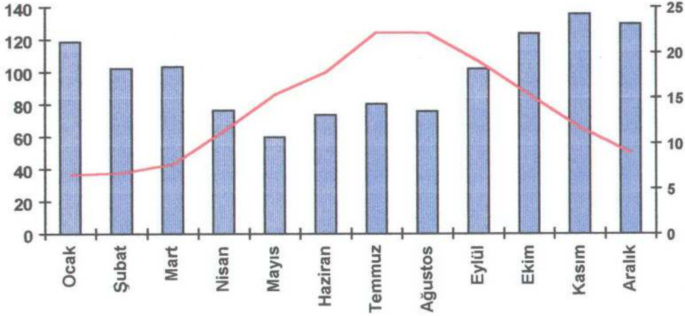
Grafik 7 : Ordu Şehri'nde Ortalama Sıcaklık ve Ortalama Yağış Diyagramı.
