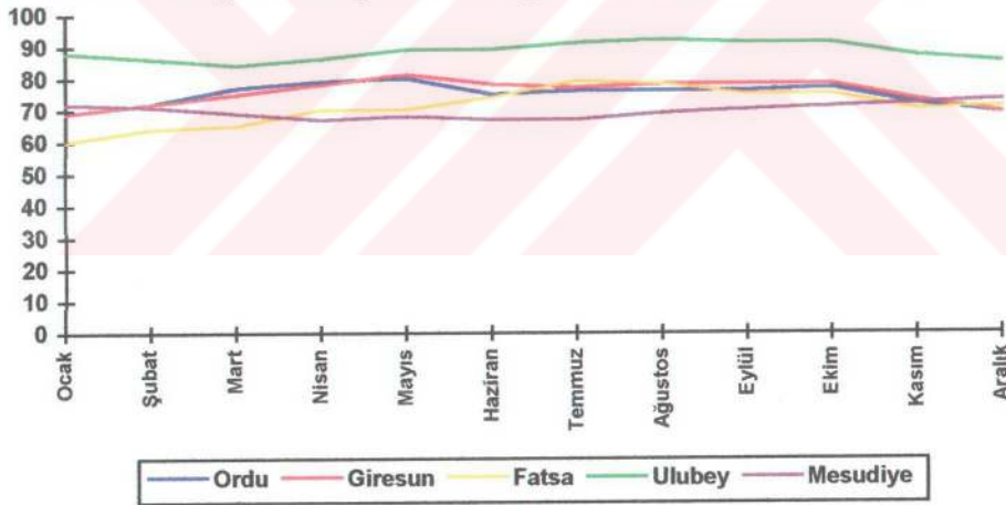
Grafik 5 : Ordu Şehri ve Çevre İstasyonlarda Aylara Göre Nispi Nem Dağılışı.
