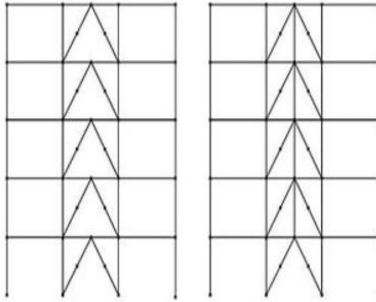
Figure 2.13 Brace configuration (Karimi et al., 2013)
