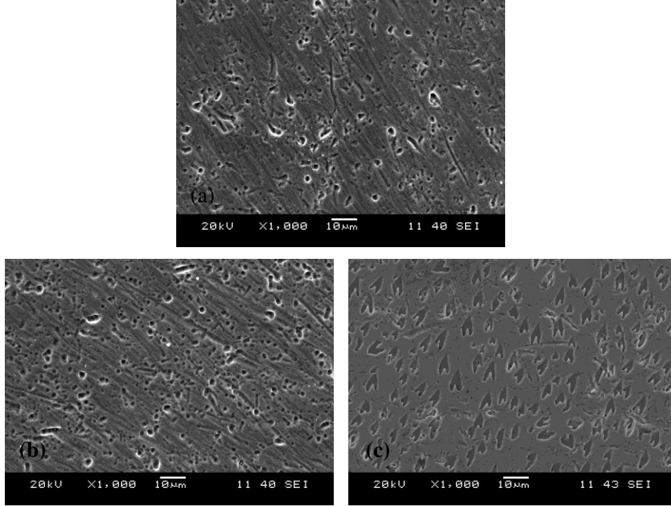
Şekil 6.23 Ti-Nb-Al alaşımının içyapı SEM görüntüleri (a) döküm sonrası, (b) 1000°C/ 2 saat + sıcak dövme, (c) 1000°C/ 5 saat ısıt işlem sonrasında gözlenen “kalp” şeklindeki bölgeler.
