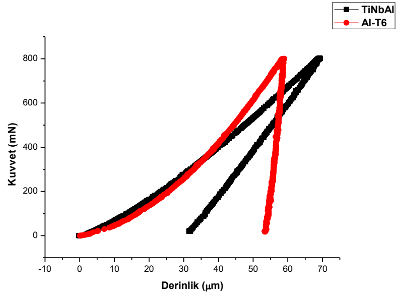
Şekil 6.27 Ti-Nb-Al alaşıımı ve Al-T6 alaşıımı için 800mN maksimum yükteki Kuvvet-Derinlik grafiği
