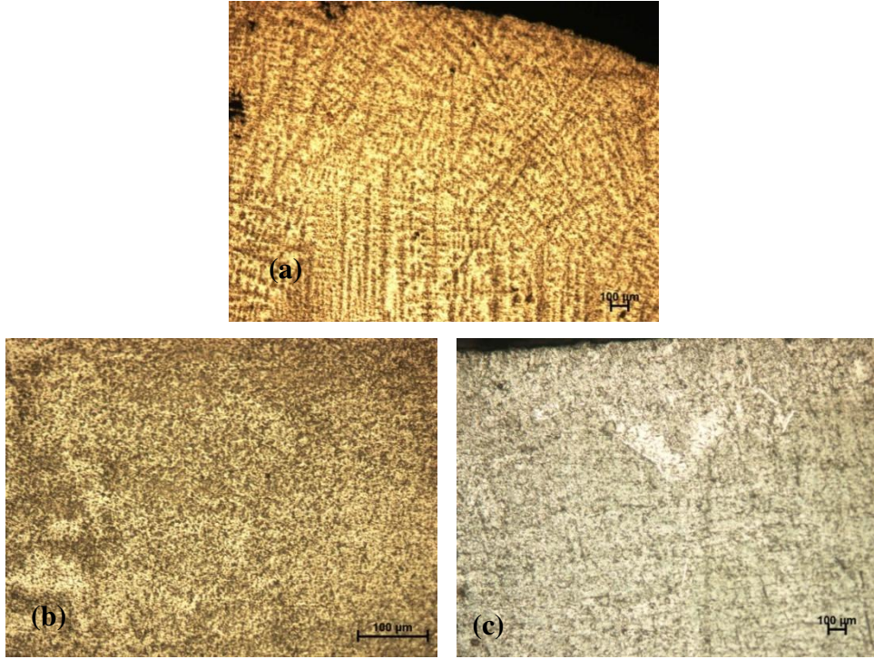
Şekil 6.22 Ti-Nb-Al alaşımının içyapı optik mikroskop görüntüleri (a) döküm sonrası, (b) 1000°C/ 2 saat + sıcak dövme, (c) 1000°C/ 5 saat ısıt işlem
