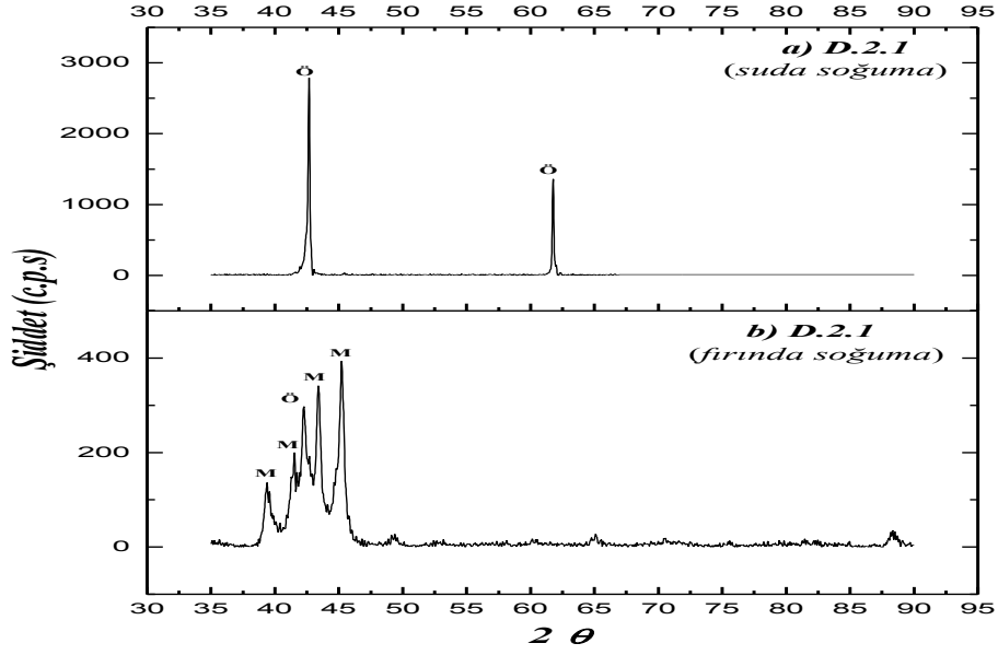
Şekil 6.15 D-2.1 numunesine ait XRD sonuçları (a) 1000°C/29 saat + suda soğutma, (b) 500°C/2 saat + firında soğutma.
