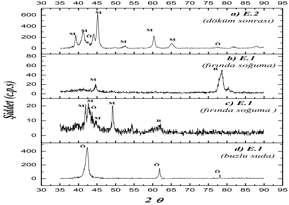
Şekil 6.16 E ingotundan alınan XRD sonuçları (a) Döküm sonrası, (b) 950°C/10+ firında soğutma, (b) 950°C/10+ firında soğutma numunenin farklı yerinden alınan (d) 850°C/5 saat +buzlu suda soğutma
