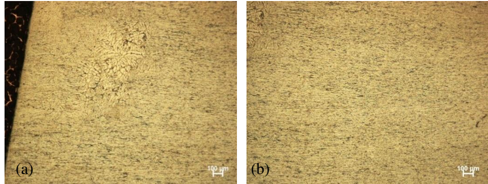
Şekil 6.8 D-2.2 numunesinin 850°C/30dk + buzlu suda soğutma sonrası optik mikroskop görüntüleri
