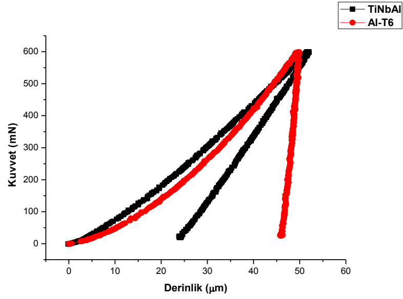
Şekil 6.26 Ti-Nb-Al alaşıımı ve Al-T6 alaşıımı için 600mN maksimum yükteki Kuvvet-Derinlik grafiği
