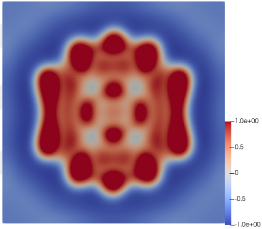
(d) c_1 at t = 0.005
