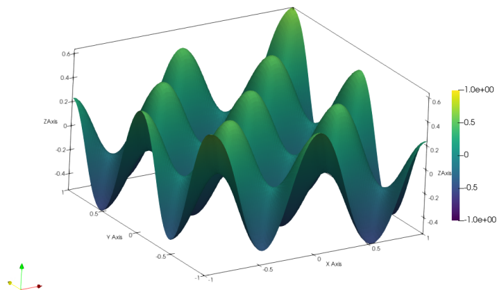
(d) Concentration at t = 10
