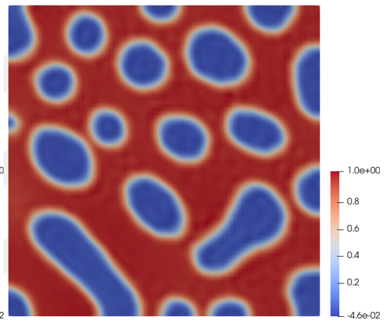
(d) Concentration at t = 0.0005
