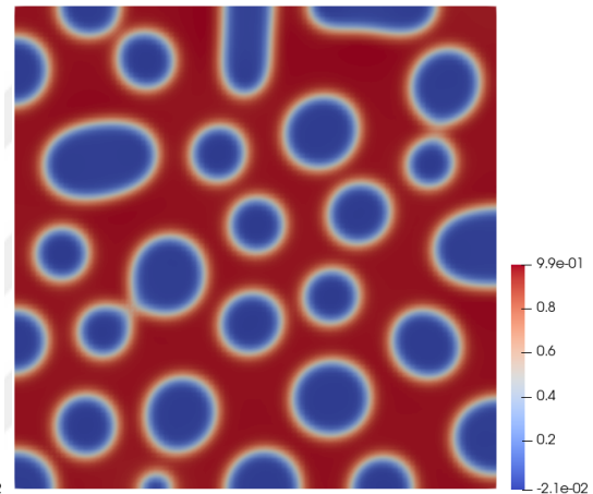
(d) Concentration at t = 0.0005
