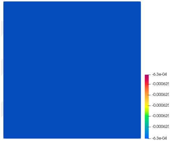
(d) Concentration for f(c) = c^2 - 1
