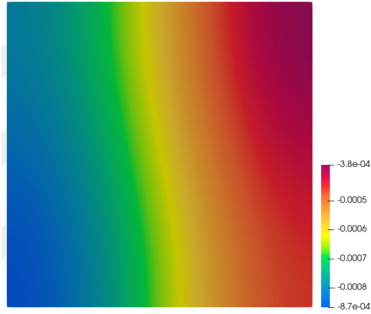
(d) Concentration for f(c) = c^2 - 1
