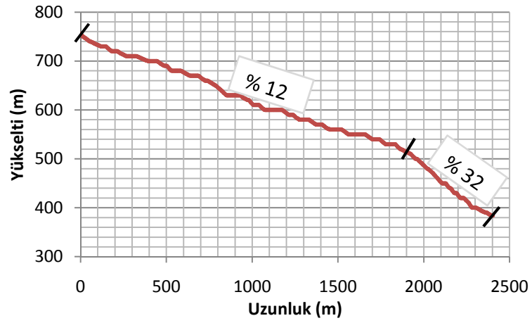
Şekil 3.4: Akbağlık deresi boyuna profili (ölçeksiz)
