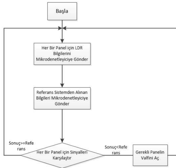
Şekil 3.16 Kontrol algoritması.
