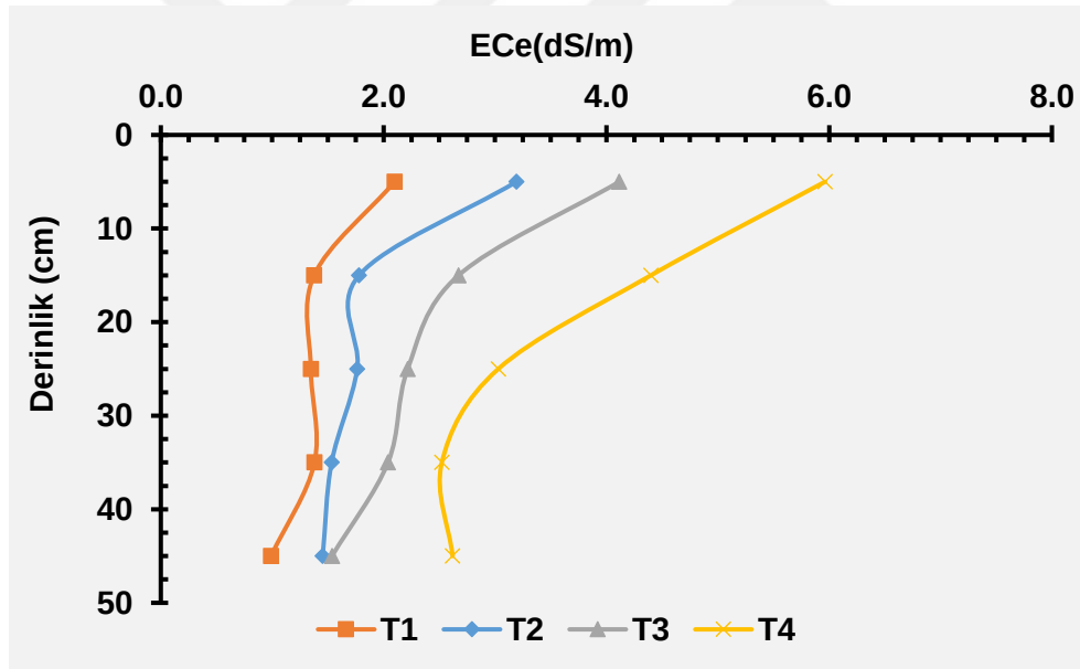
Şekil 3.5. Yıkama başlangıcı sera toprağı tuzluluk (ECe, dS/m) durumu
