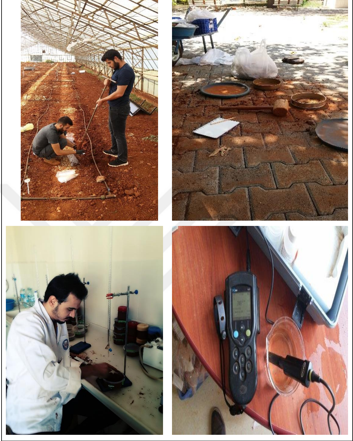
Şekil 3.8. Yıkama işlemleri için toprak örneklerinin alınması, topraların elenmesi, çamurlar süzüklerinin hazırlanması, EC ve pH okumaları
