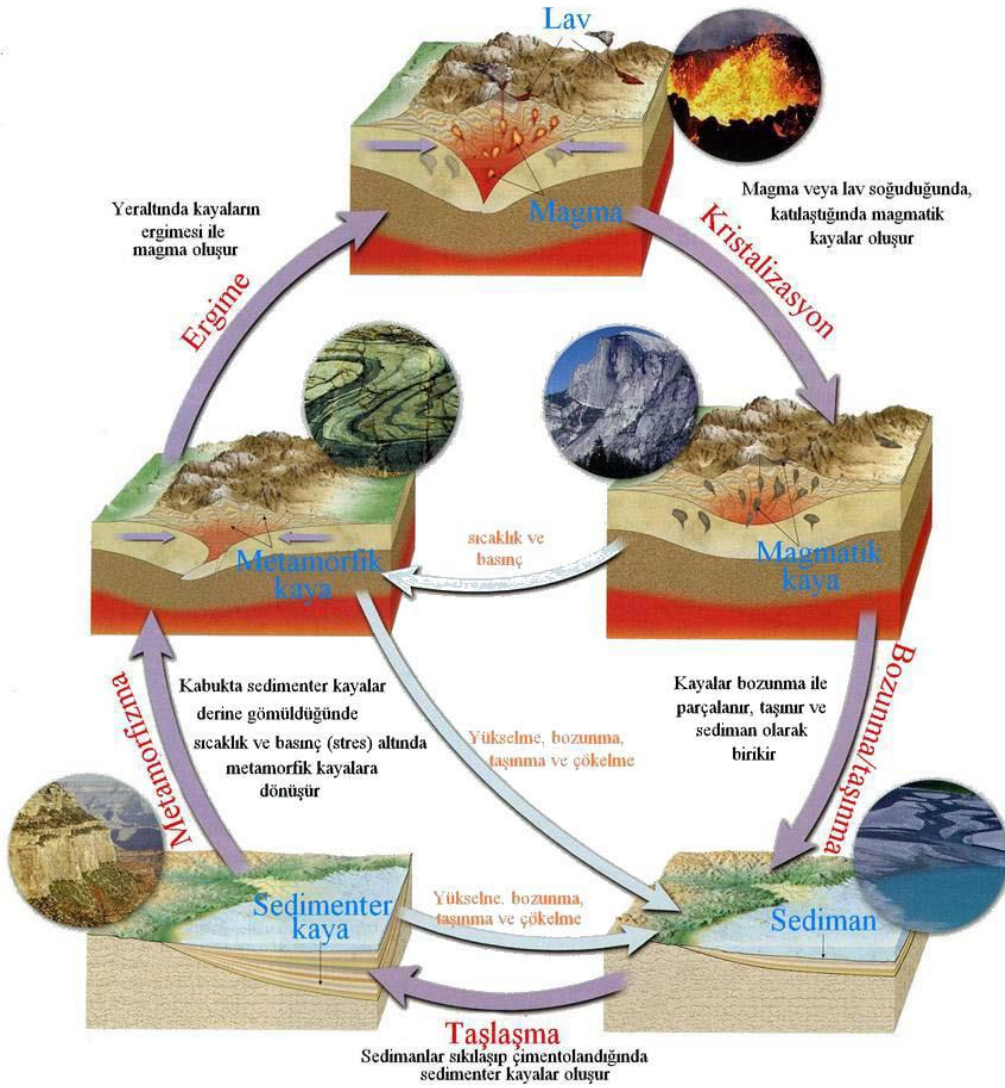
Resim 1. Kaya döngüsü
