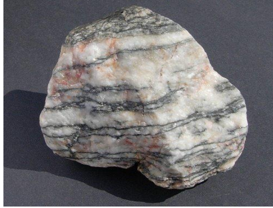
Resim 11. Gnays
