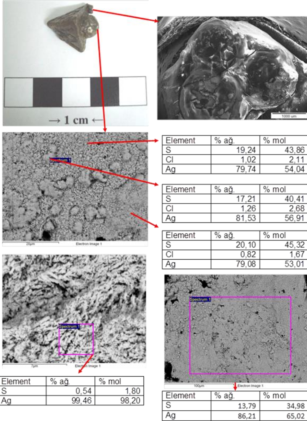
 ekil 4.37. M17 kodlu numunenin SE ve BSE g r nt leri ve  e itli noktaların yarı kantitatif EDX analiz sonu ları (% a ırlık ve % mol)
