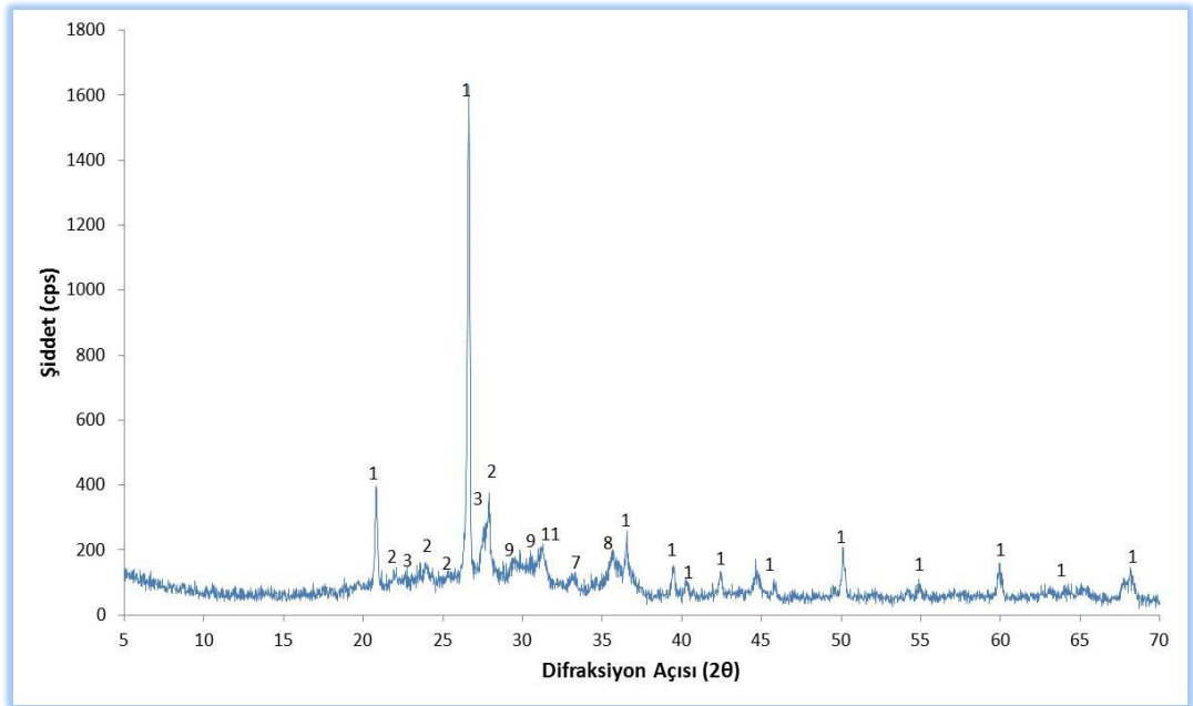
Şekil 4.52. 17 kodlu numuneye ait temsili XRD grafiği
