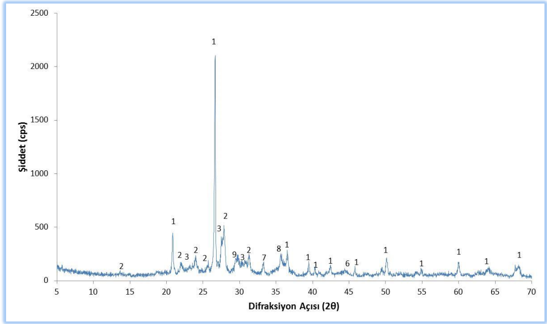
Şekil 4.51. 6-1 kodlu numuneye ait temsili XRD grafiği
