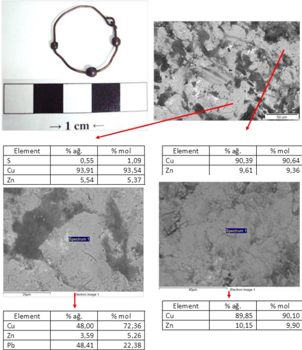
 ekil 4.30. M10 kodlu numunenin BSE g r nt leri ve  e itli noktaların yarı kantitatif EDX analiz sonu ları (% a ırlık ve % mol)
