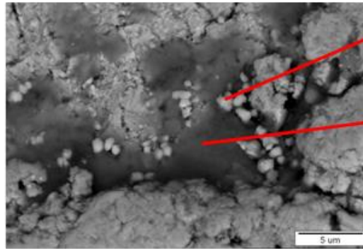
Şekil 4.21. M1 kodlu numunenin SE ve BSE görüntüleri ve çeşitli noktaların yarı kantitatif EDX analiz sonuçları (% ağırlık ve % mol)
