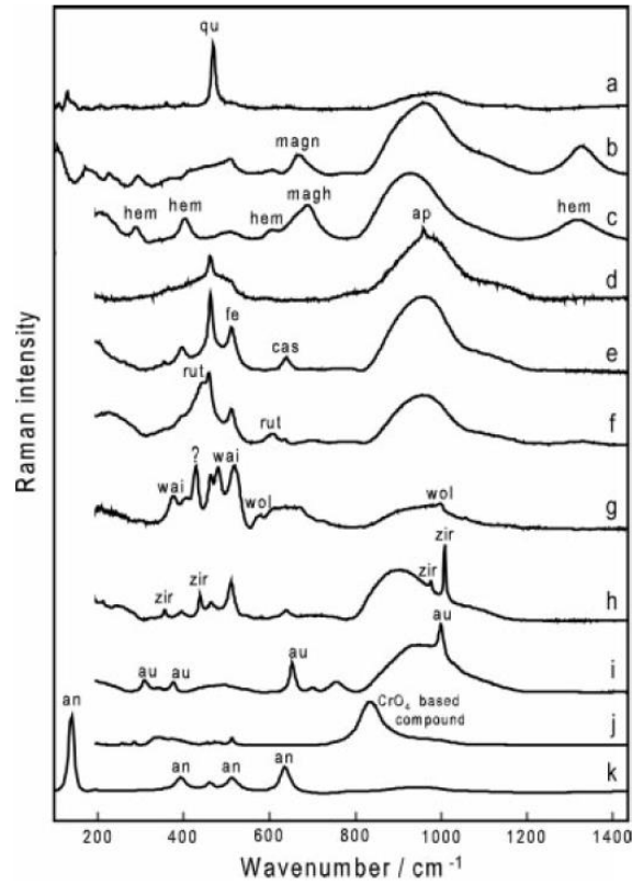
Şekil 4.57. Seramik numunelerinin sırlarında bulunan pigmentlerin mikro-Raman spektrumları
