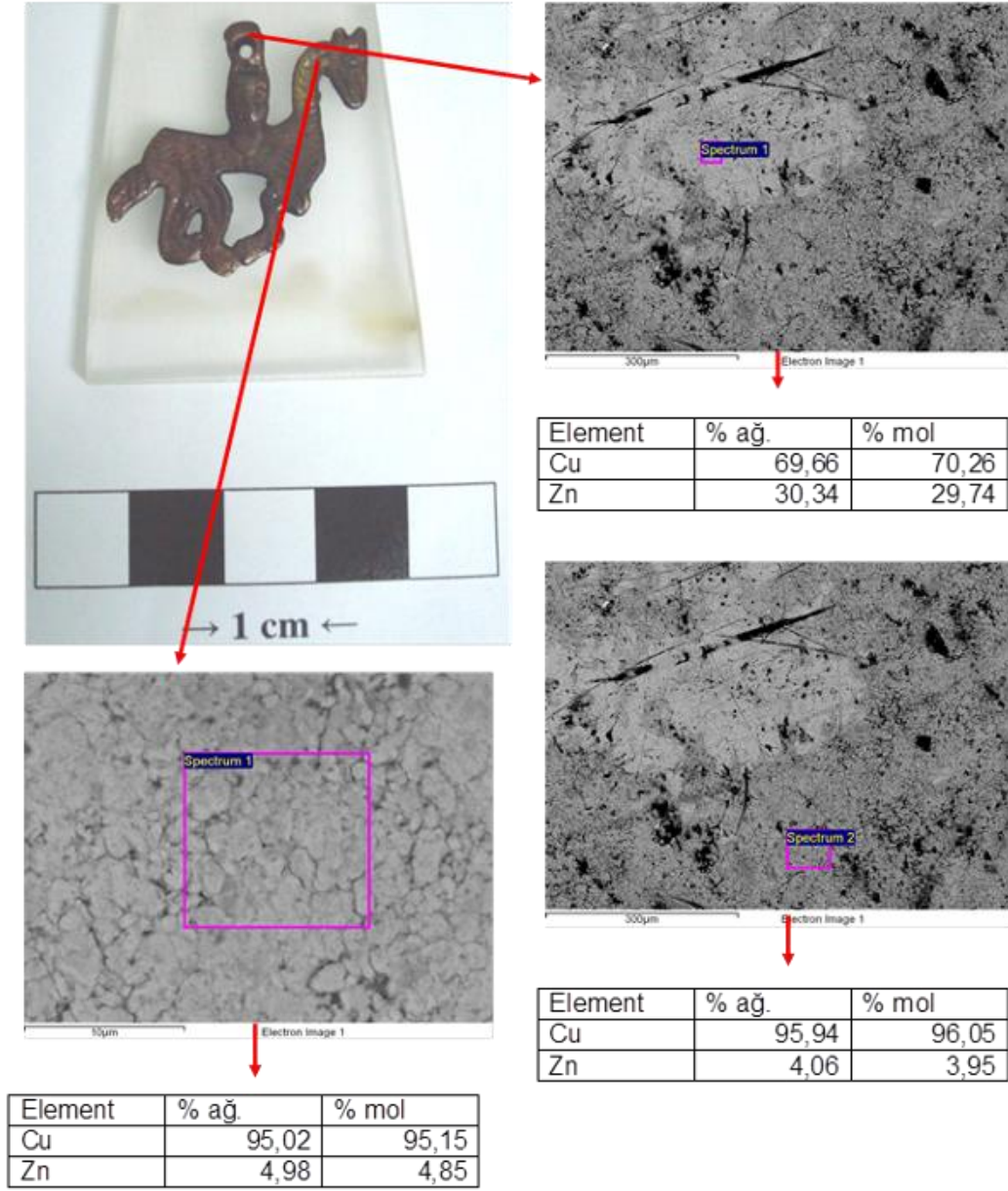
Şekil 4.36. M16 kodlu numunenin BSE görüntüleri ve çeşitli noktaların yarı kantitatif EDX analiz sonuçları (% ağırlık ve % mol)
