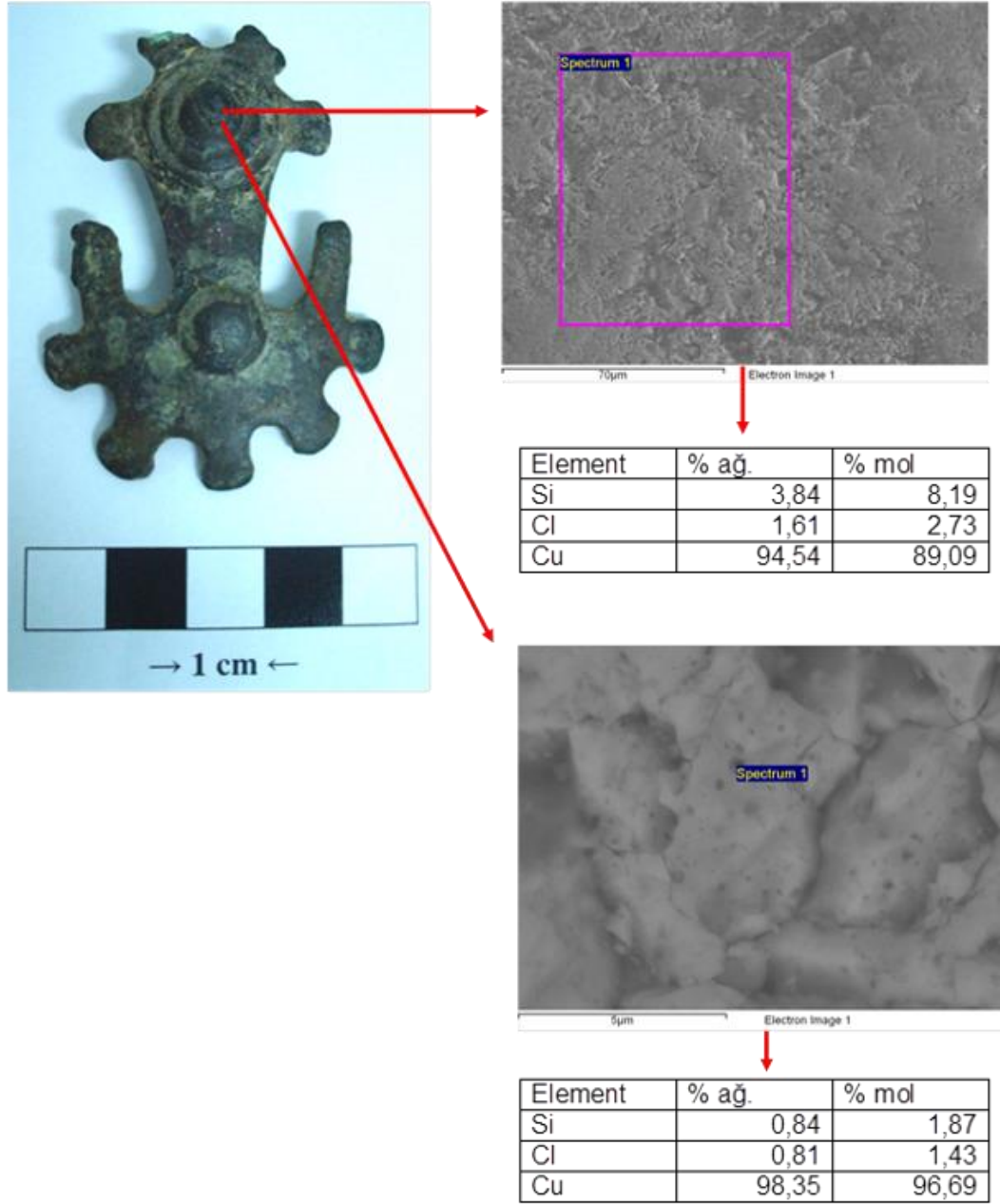
Şekil 4.40. M20 kodlu numunenin SE ve BSE görüntüleri ve çeşitli noktaların yarı kantitatif EDX analiz sonuçları (% ağırlık ve % mol)
