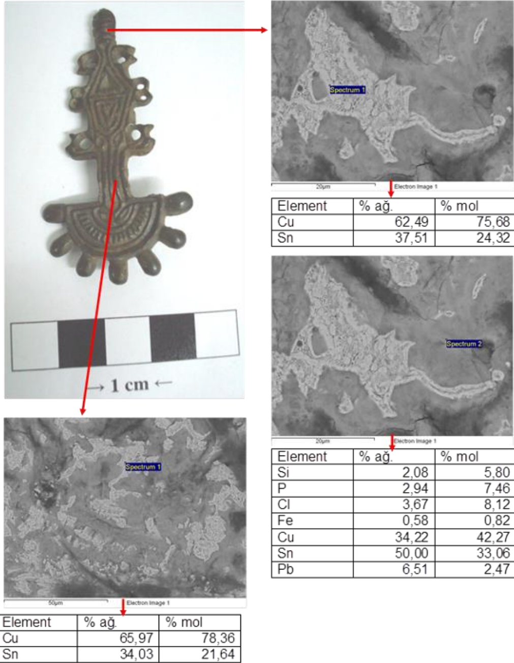
Şekil 4.41. M21 kodlu numunenin BSE görüntüleri ve çeşitli noktaların yarı kantitatif EDX analiz sonuçları (% ağırlık ve % mol)
