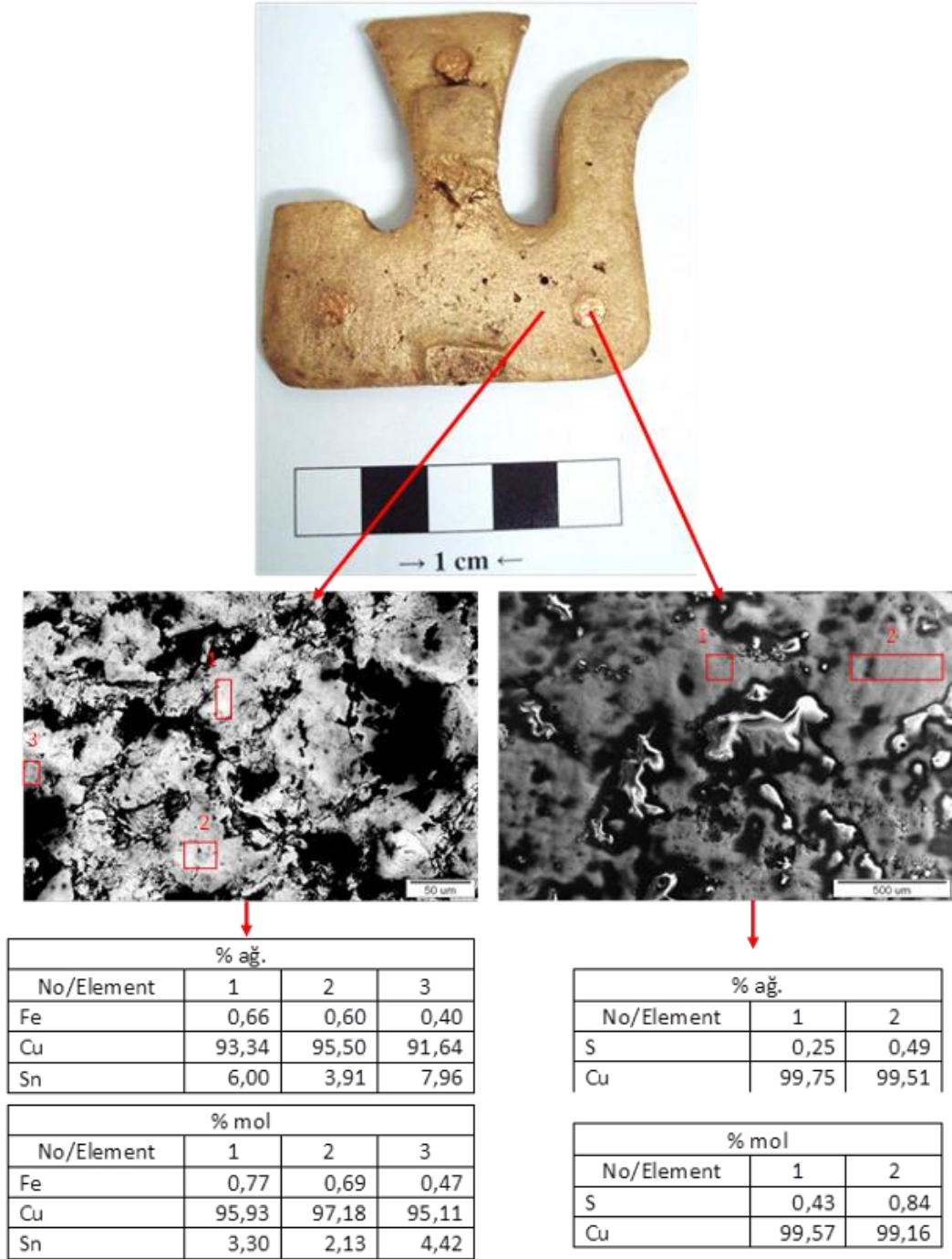
Şekil 4.24. M4 kodlu numunenin SE ve BSE görüntüleri ve çeşitli noktaların yarı kantitatif EDX analiz sonuçları (% ağırlık ve % mol)
