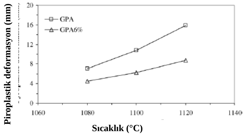
Şekil 3.5. Standart ve cam kırığı ilave edilen bünynenin farklı sıcaklıklarda piroplastik davranışı (Rambaldi ve ark. 2006)
