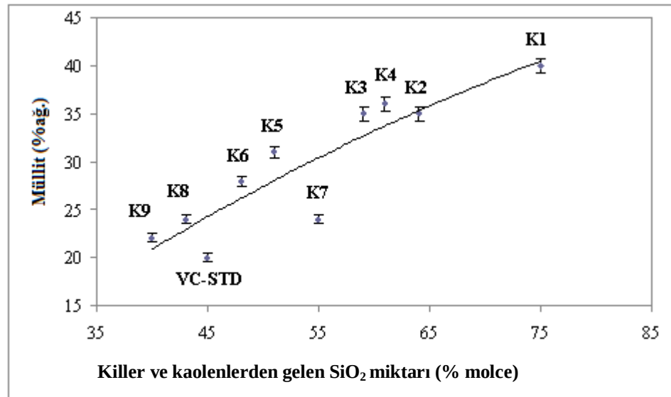
Şekil 5.24. Kil-kaolen bileşiminden gelen \text{SiO}_2 miktarının müllit miktarı üzerine etkisi
