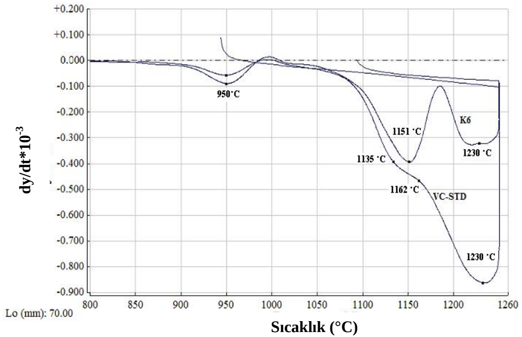
Şekil 5.28. VC-STD ve K6 bünyelerinin deformasyon hızlarını ifade eden türev eğrileri
