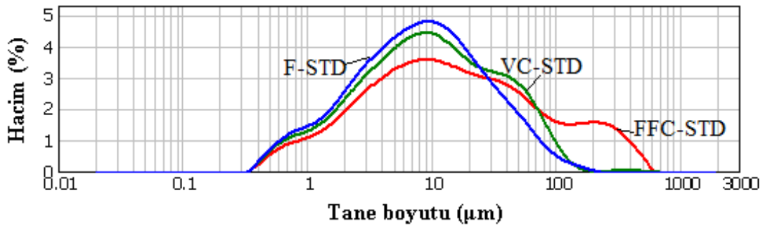
Şekil 5.3. Çamurların tane boyut dağılımı grafikleri
