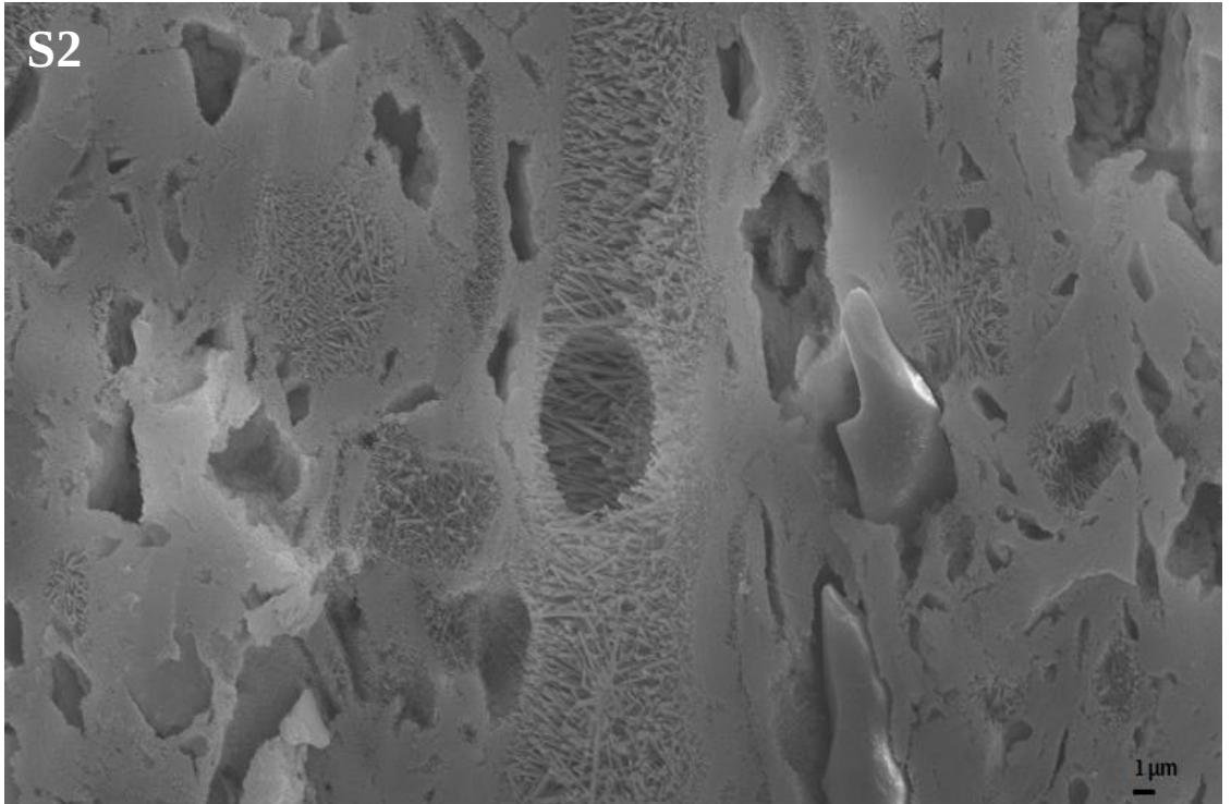
Şekil 6.3. 1250°C’ de pişirilmiş K6 ve S2’ nin dağlanmış kırık yüzeylerine ait 5000x büyütmedeki geri yansıyan elektron görüntüleri
