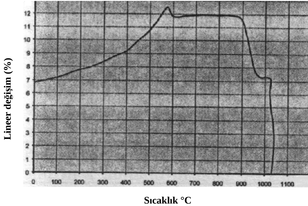
Şekil 2.9. Vitrifiye bünyenin dilatometre eğrisi (Fortuna, 2000)
