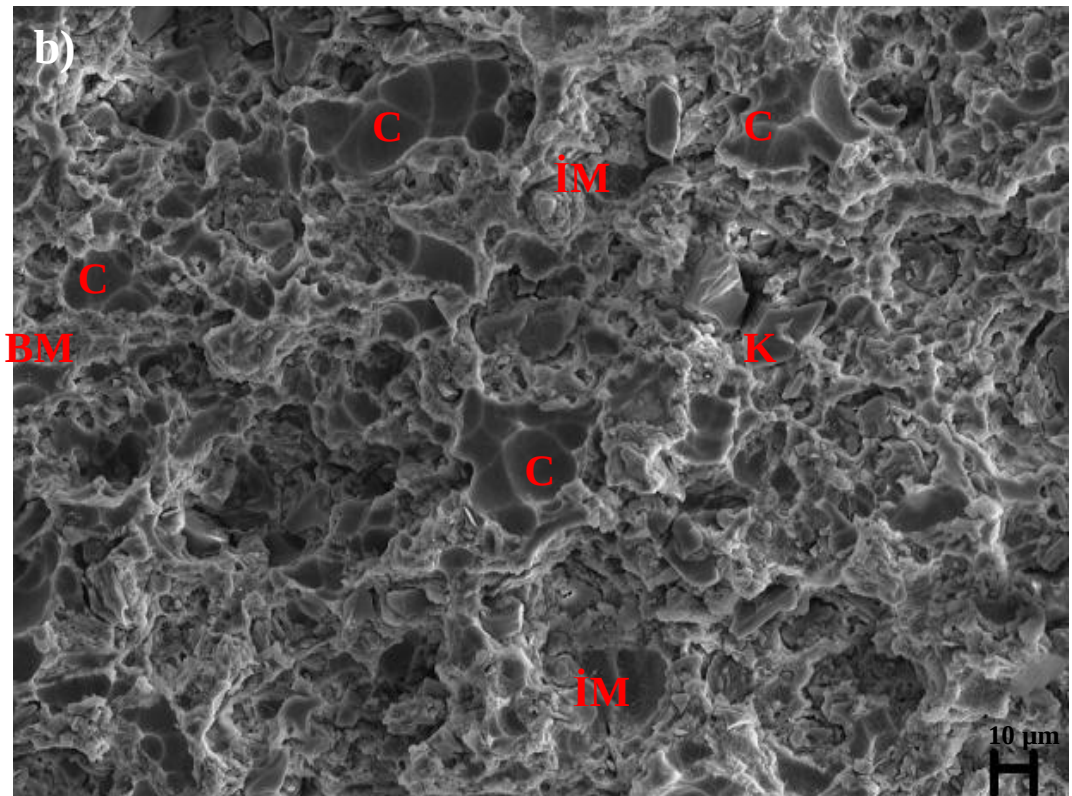
Şekil 5.29. Pişmiş bünyelerin dağlanmış kırık yüzeylerinden alınan geri yansıyan elektron görüntüleri a) K6 bünyesi b) VC-STD bünyesi (C: camsı faz, BM: birincil müllit, İM: ikincil müllit, K:kuvars)
