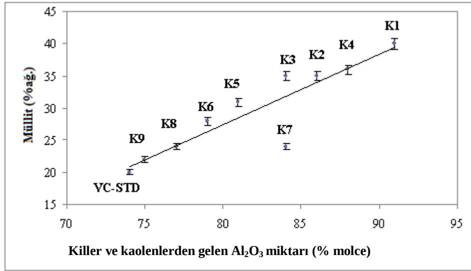
Şekil 5.23. Kil-kaolen bileşiminden gelen \text{Al}_2\text{O}_3 miktarının müllit miktarı üzerine etkisi
