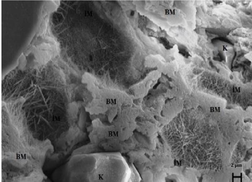
Şekil 5.30. K6' nın 5000X büyütmede alınmış geri yansıyan elektron görüntüleri. (C: camsi faz, BM: birincil müllit, İM: ikincil müllit, K:kuvars)
