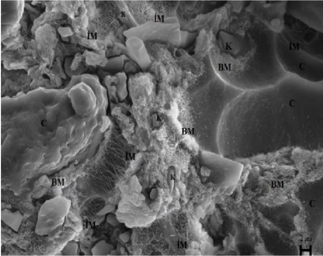
Şekil 5.31. VC-STD' nin 5000X büyütmede alınmış geri yansıyan elektron görüntüleri. (C: camı faz, BM: birincil müllit, İM: ikincil müllit, K:kuvars)
