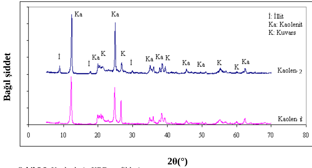
Şekil 5.2. Kaolenlerin XRD grafikleri
