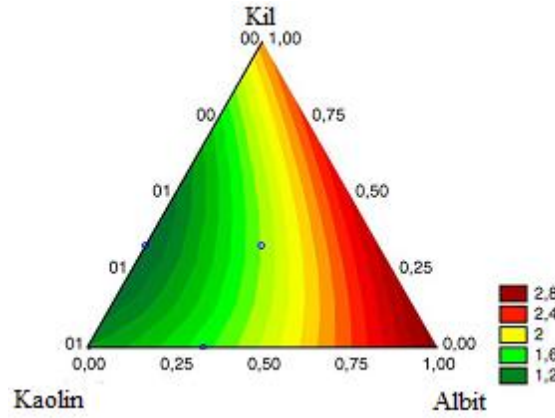
Şekil 3.3. Çalışılan sistemde piropplastik indeks için cevap yüzeyi. Yeşil renkten kırmızıya doğru gidilmesi PI değerlerindeki artışı ifade etmektedir (Bernardin ve ark., 2006)
