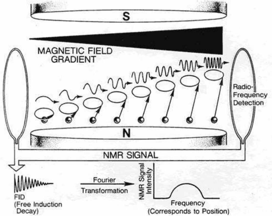
Şekil 12. Elde edilen zaman domain bilgilerinin Fourier transformasyonu ile frekans domain bilgiler haline dönüştürülmesi.
