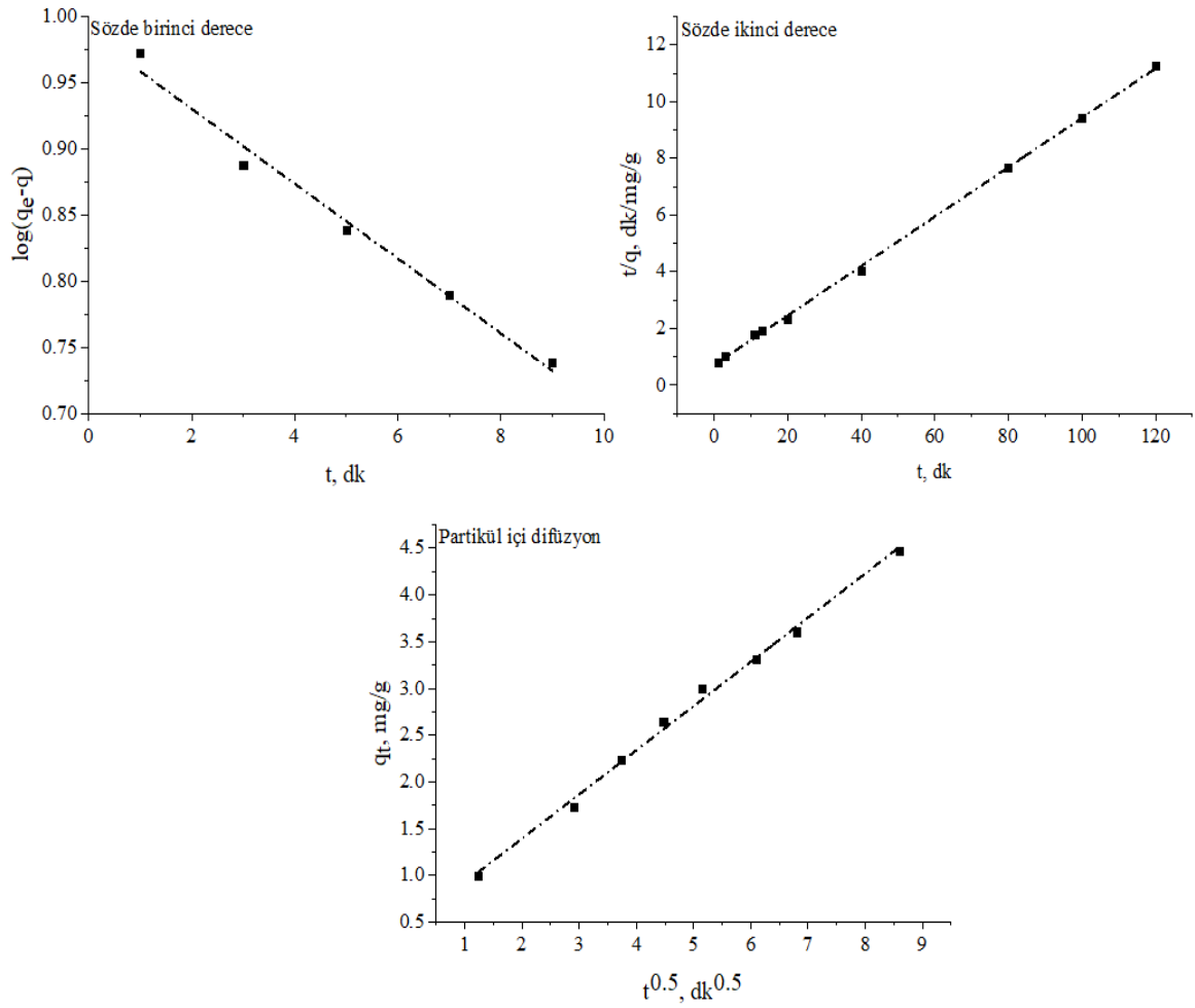
Şekil 3.12. Malahit yeşili boyanın adsorpsiyonu için sözde birinci mertebe, sözde ikinci mertebe ve partikül içi difüzyon kinetik modelleri
