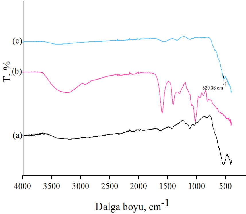
Şekil 3.1. (a) Manyetik \text{Fe}_3\text{O}_4 parçacıkları (b) Aljinat (c) Seryum temelli manyetik partiküllerin FTIR spektrumları
