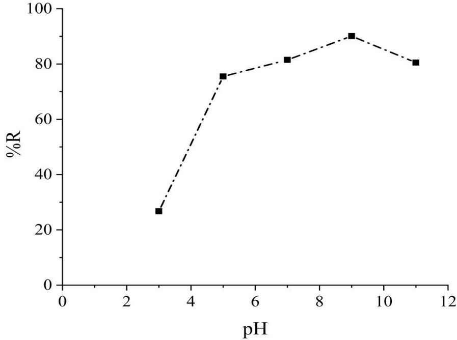
Şekil 3.6. pH'ın malahit yeşili boyanın giderimine etkisi (t:100 dk, m:10 mg, C 0 :10 mg/L, T:298 K)
