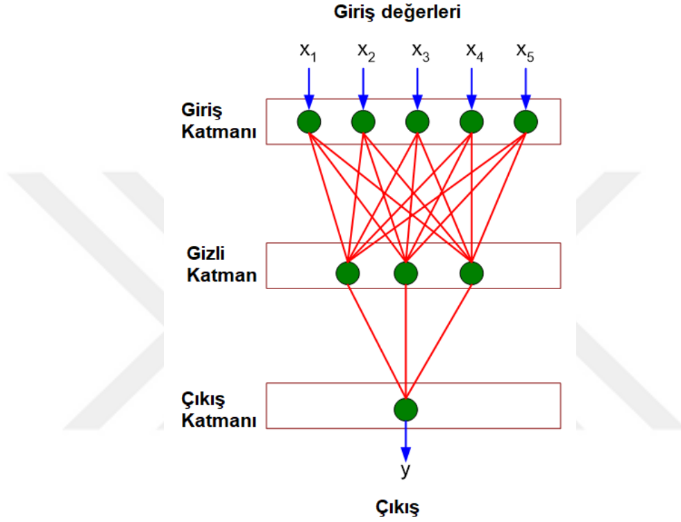
Şekil 2.10. Yapay sinir ağı katmanları
