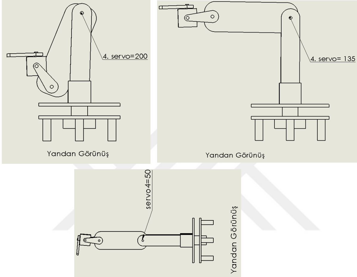
Şekil 3.4. Servo 4 konumları
