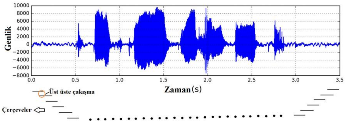
Şekil 2.6. Çerçeveleme örneği
