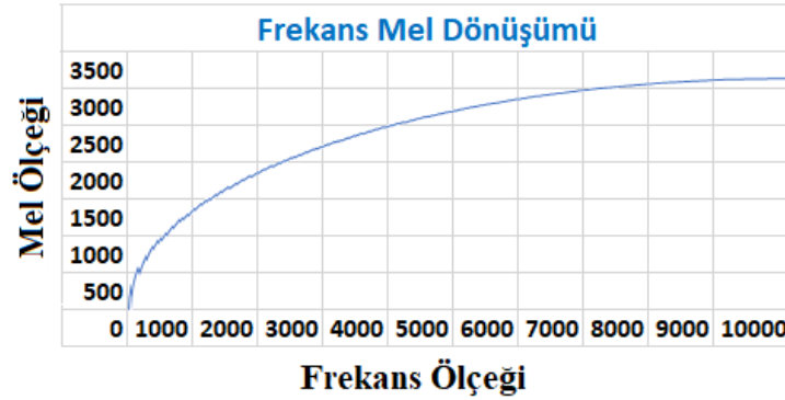
Şekil 2.8. Frekans-Mel Dönüşümü
