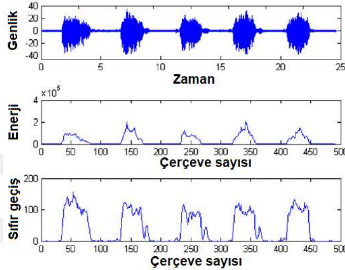
Şekil 2.4. Sinyalin sıfır geçiş ve kısa süreli enerji grafiği
