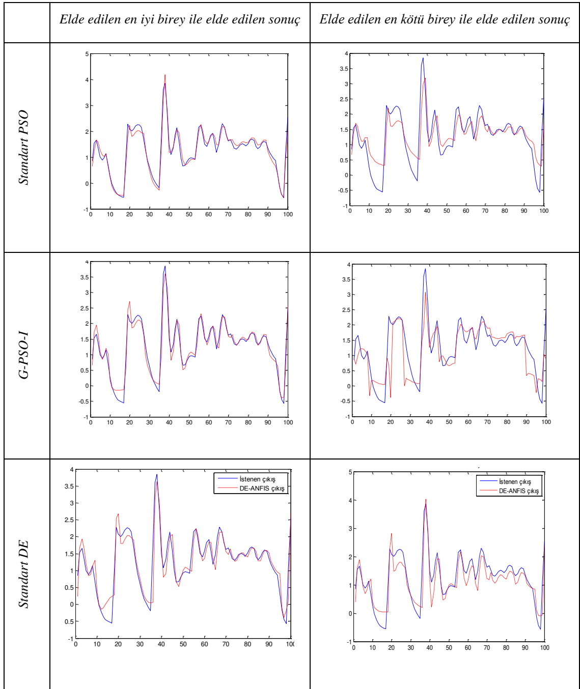
Şekil 4. 25. PSO ve DE öğrenmeli ANFIS ile ÖDS 4 için eğitim fazı sistem tanıma sonuçları
