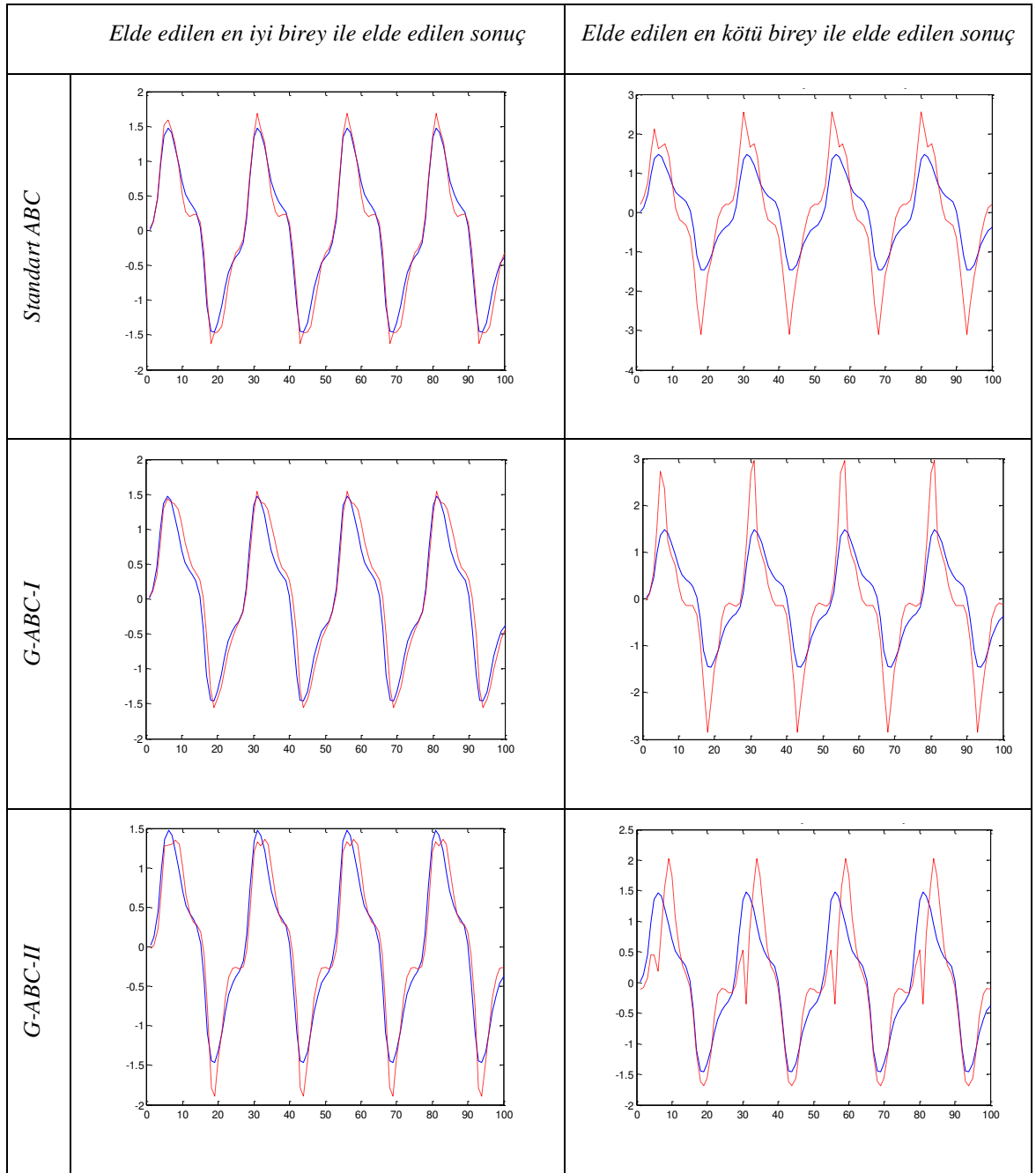
Şekil 4. 13. ABC öğrenmeli ANFIS ile ÖDS 2 için test fazı sistem tanıma sonuçları
