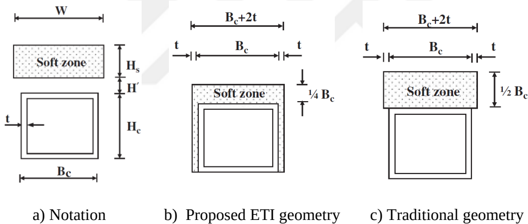
Figure 2.11. Trench applications (Kang, Parker, Kang, et al., 2008)
