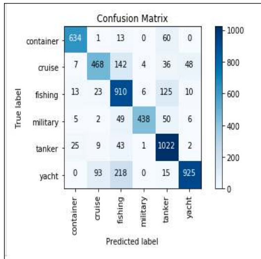
Xception
