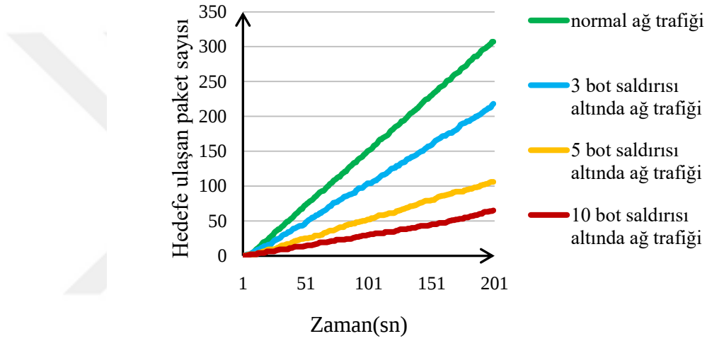
Şekil 7.10. Farklı bot sayıları ve DDoS saldırısı altında ağ trafiği çıkışı
