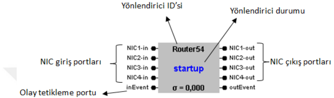
Şekil 3.5. Atomik DEVS modeli
