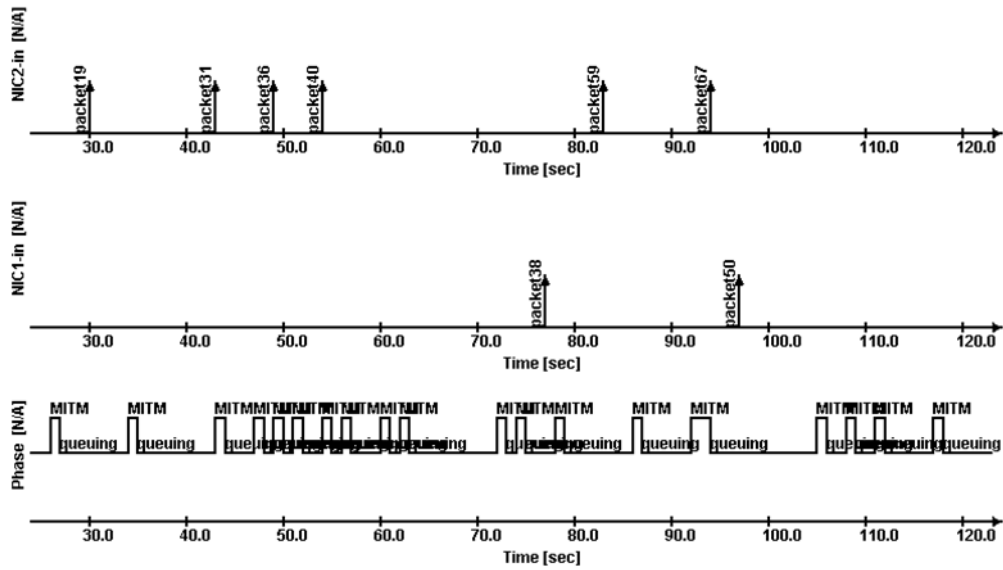
Şekil 6.23. Ortadaki adam saldırısına ait paket ve durum değişim grafikler
