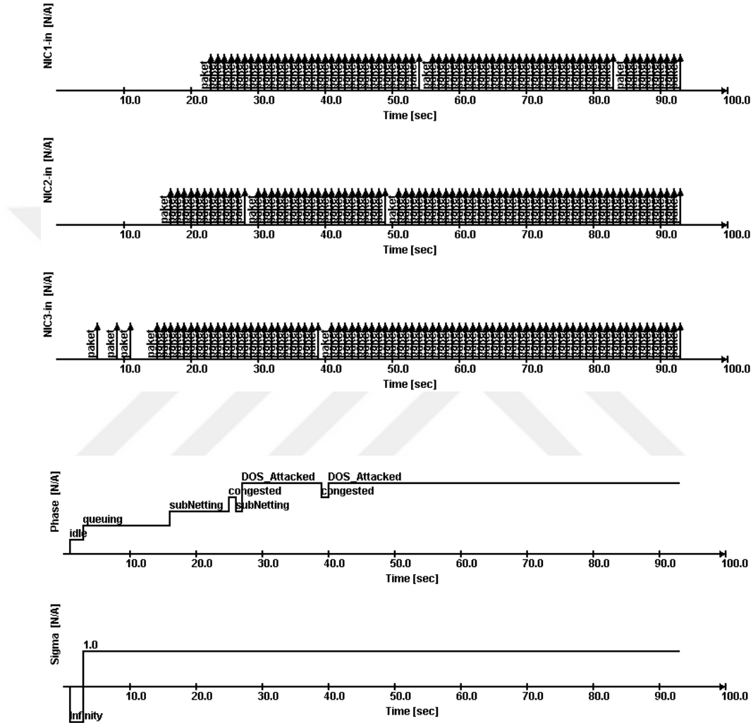
Şekil 6.13. DDoS saldırısına ait hedef düğümün giriş portlarının izleme penceresi ve durum değişim grafiği
