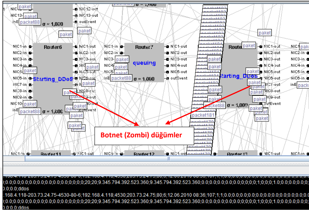
Şekil 6.10. DDoS saldırı aşamasındaki Botnetler
