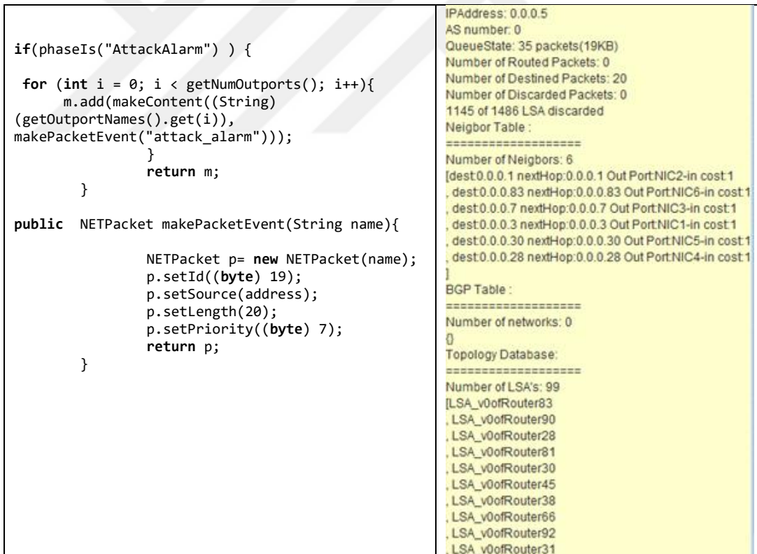
Şekil 6.30. (a) Atomik modelin saldırı alarm paketleri üreten kod kısmı (b) Hedef düğümün komşuluk tablosu
