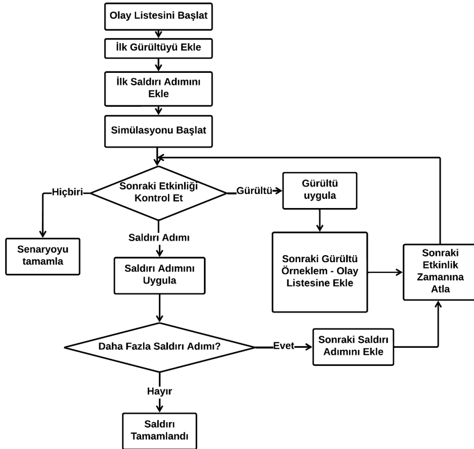
Şekil 5.7. Saldırı senaryosu
