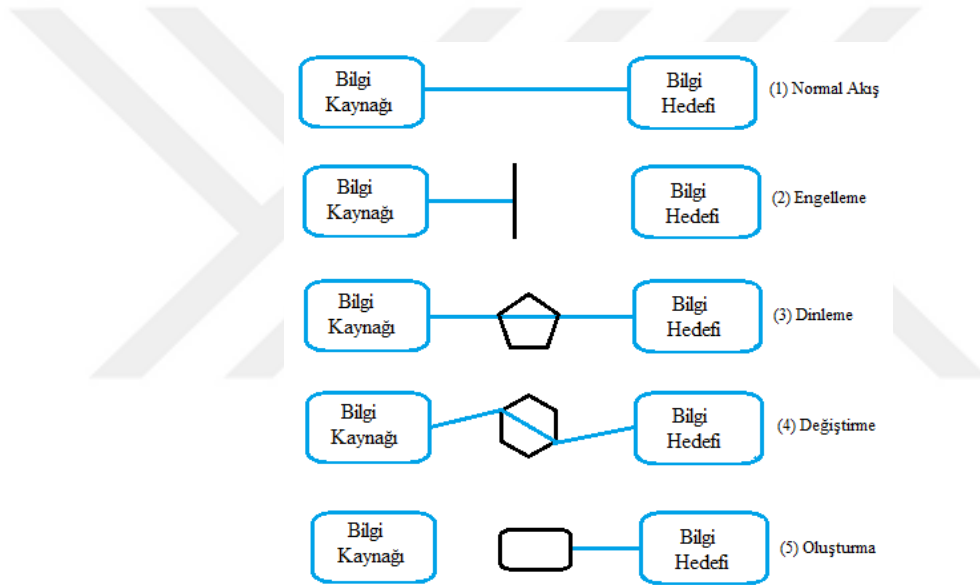
Şekil 2.6. İletişim Hedefli Saldırı Tipleri
