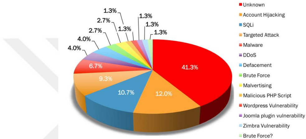
Şekil 2.7. Şubat 2016 Saldırı Kullanılan Saldırı Teknikleri İstatistiği ( [32]'dan alınmıştır).
