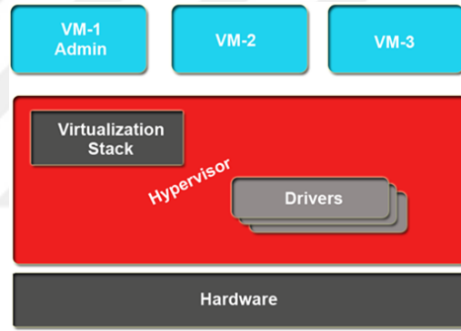
Şekil 2.11. Monolithic Hypervisor [39]
