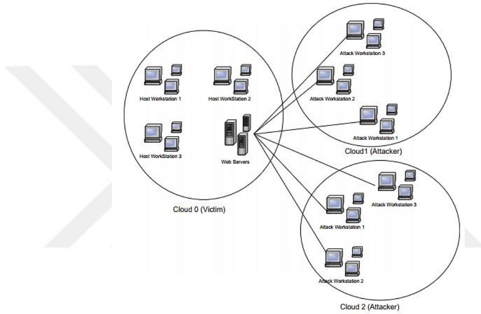
Şekil 2.9. Bulutlar Arası Saldırıları ( [37]’den alınmıştır).
