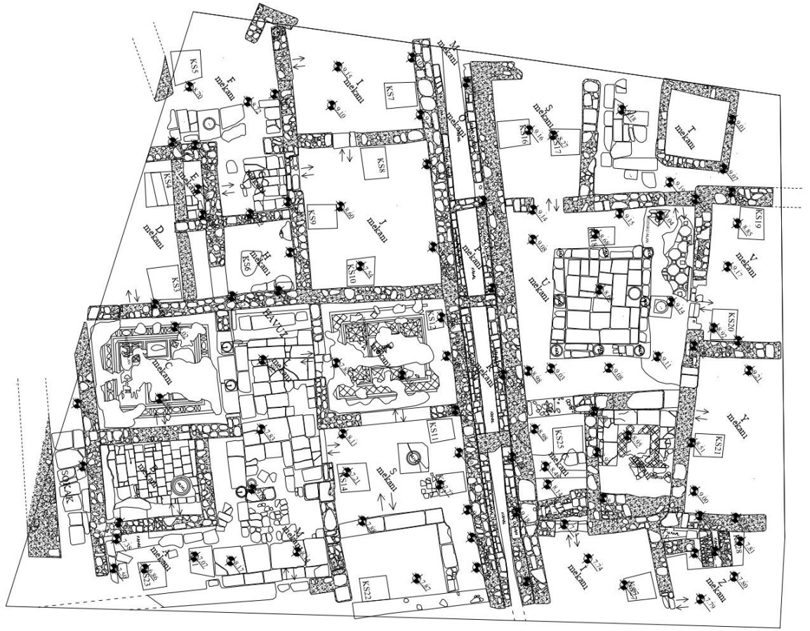
Plan 8: 807 Ada 1 Parsel, Röleve Planı (Side Kazı Arşivi)
