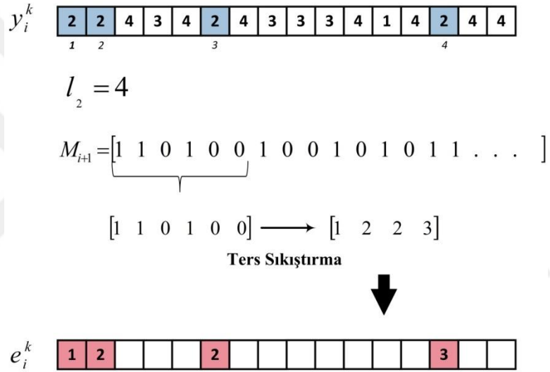
Şekil 2.12. '2' sembolü için orijinal bloğun geri elde edilmesi.
