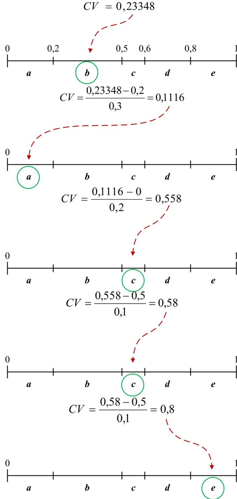
Şekil 2.7. Aritmetik kod çözümü için grafiksel gösterim.
