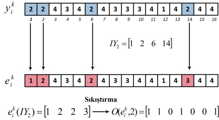
Şekil 2.11. '2' sembolü için yan bilginin oluşturulması.
