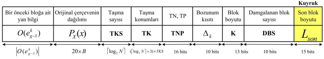
Şekil 3.4. Damgalı bir çerçevenin geri elde edilmesi için gerekli yan bilgi.
