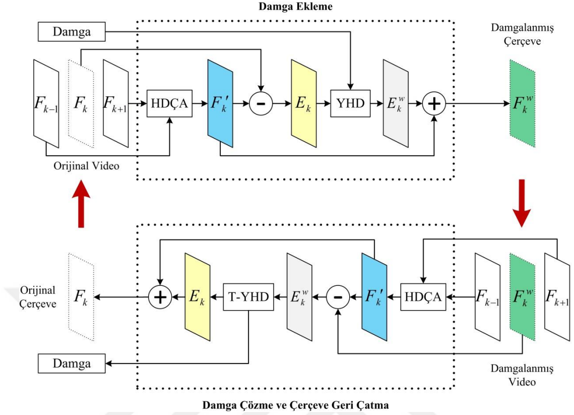
Şekil 3.2. Önerilen yöntemde bir çerçevenin damgalanmasına, geri elde edilmesine ve çerçevedeki damganın çıkartılmasına karşılık gelen blok diyagramı.
