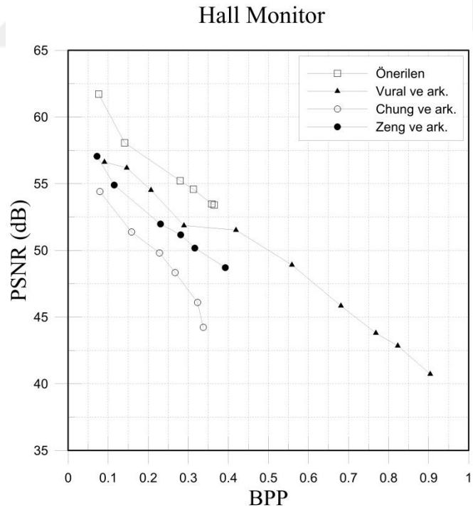
Şekil 3.7. Kapasitenin fonksiyonu olarak önerilen ve mevcut yöntemlerin Hall-Monitor videosu için sağladıkları görsel kalite.
