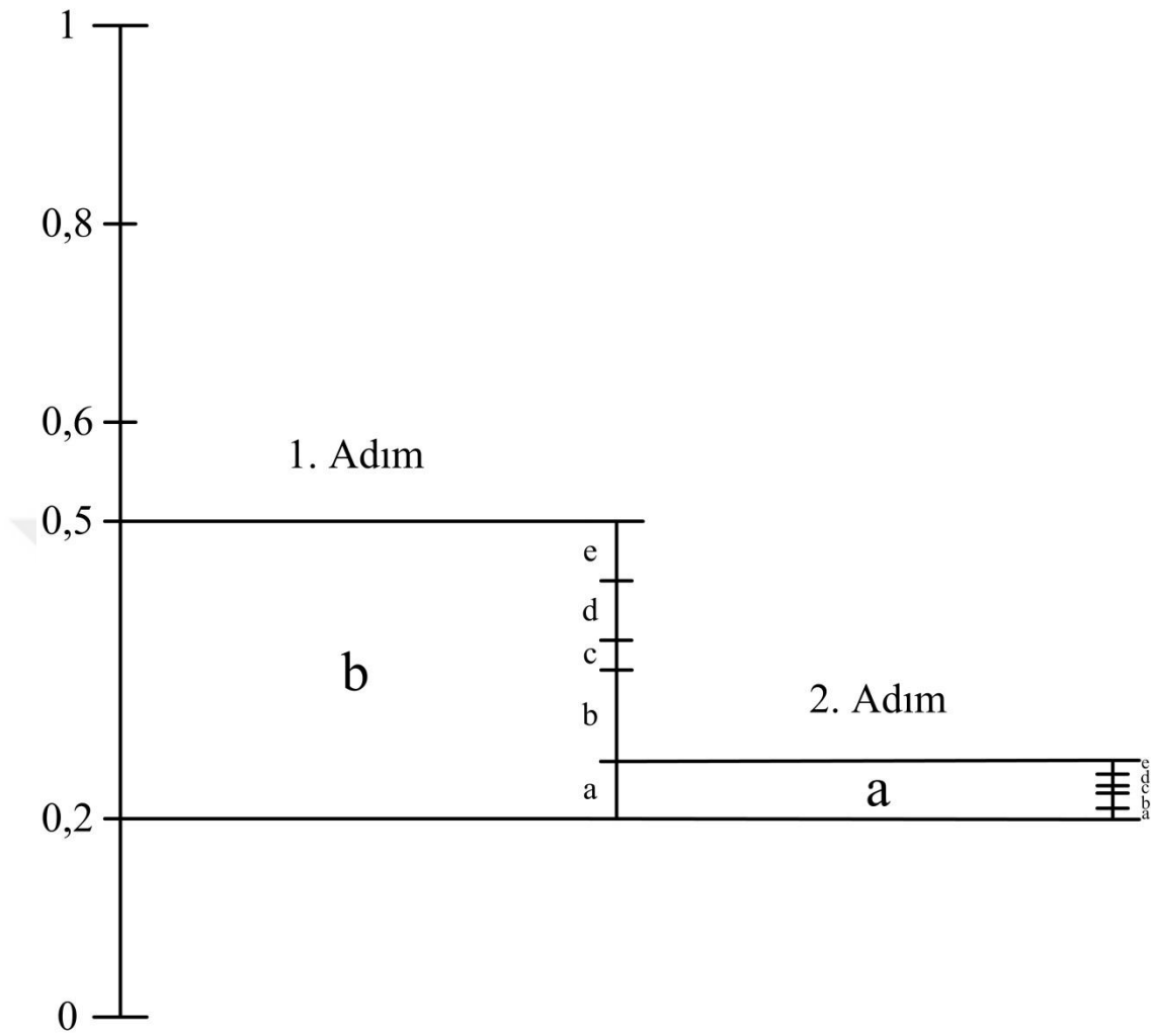
Şekil 2.5. Aritmetik kodlama sürecinin gösterimi.
