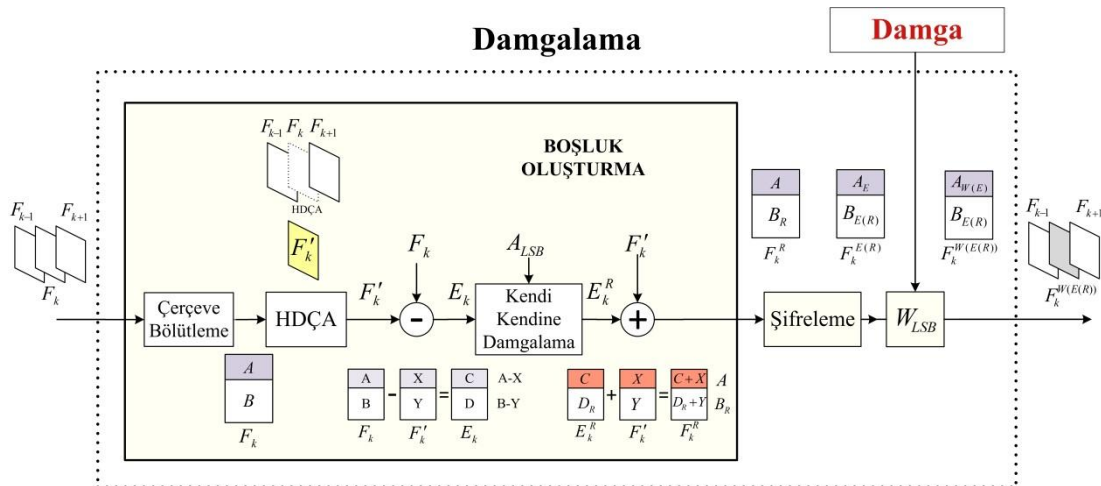
Şekil 4.2. Bir çerçeve için önerilen yöntemin damga ekleme kısmına karşılık gelen detaylı blok diyagramı.
