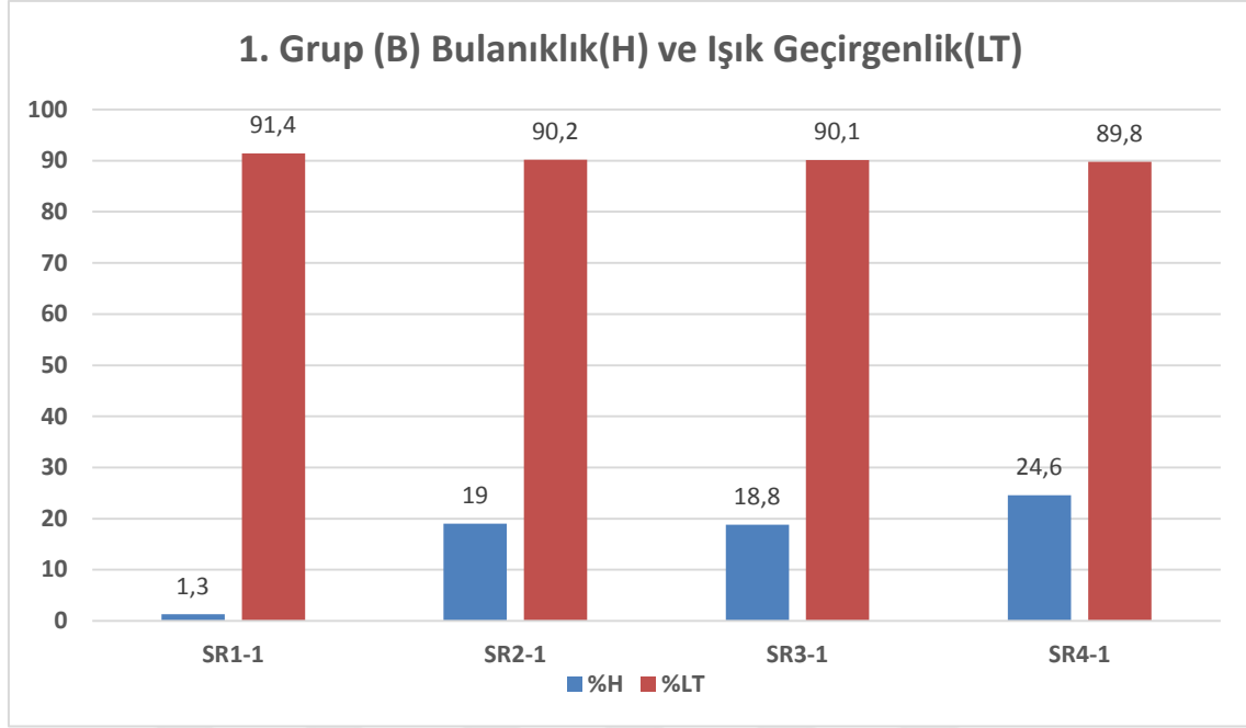
Şekil 4.2 1(B) Grup Ti ve Zr alkoksitli ve BYK katkı hazırlanan bileşimlerin %H ve %LT değerleri.
