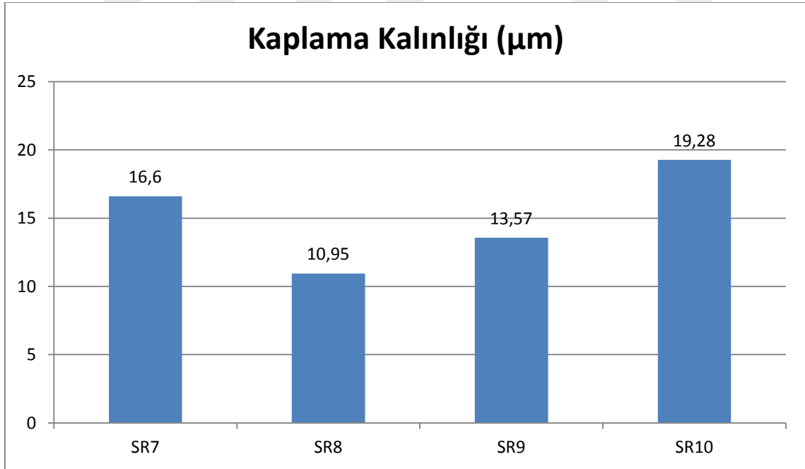
Şekil 4.28 3. Grup DAMO' lu hazırlanan bileşimlerin kaplama kalınlığı.
