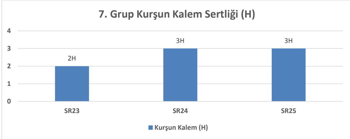
Şekil 4.24 7. Grup TEOS, koloidal silika ve asetil asetonlu hazırlanan bileşimlerin sertlik değerleri.
