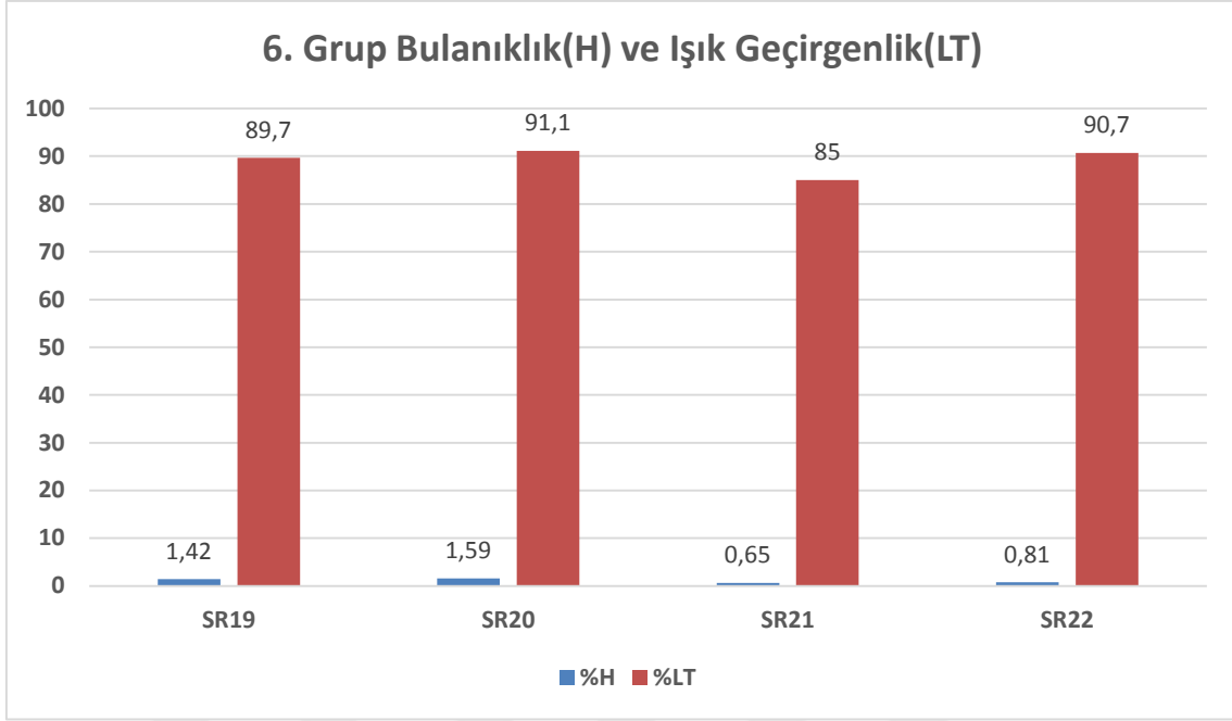
Şekil 4.7 6. Grup \text{Ce}(\text{NO}_3)_3 ve asetil asetonlu hazırlanan bileşimlerin %H ve %LT değerleri.
