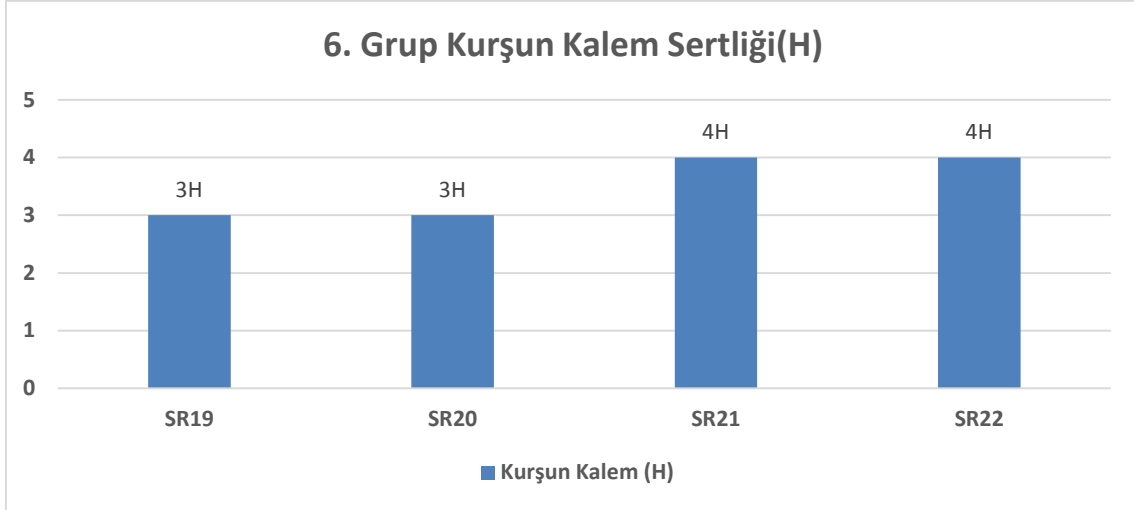
Şekil 4.23 6. Grup \text{Ce}(\text{NO}_3)_3 ve asetil asetonlu hazırlanan bileşimlerin sertlik değerleri.
