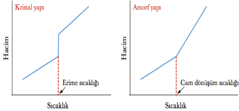
Şekil 2.1 kristal ve amorf katıların sıcaklığa bağlı olarak hacimlerinin değişimi.
