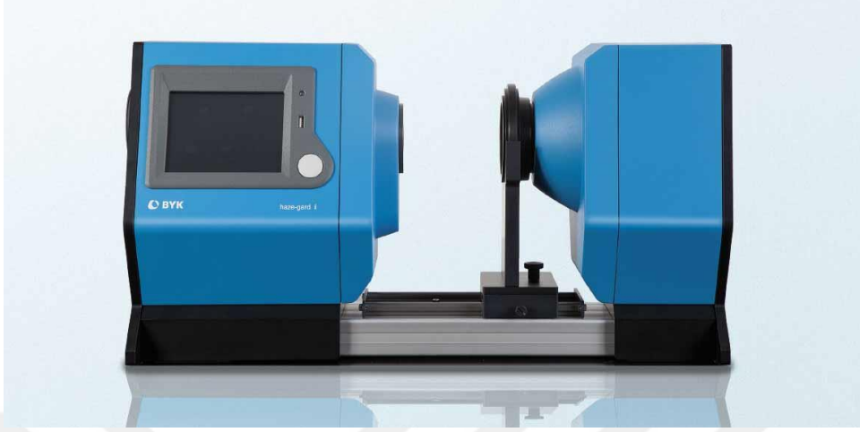
Resim 3.3 Deneyde kullanılan ışık geçirgenlik ve bulanıklık ölçüm cihazı.
