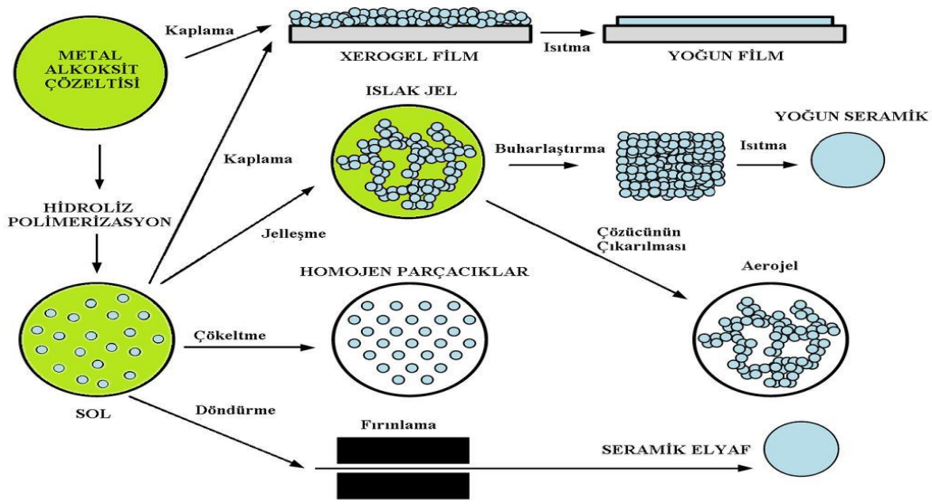
Şekil 2.5 Sol-jel ürünlerin şematik gösterimi.
