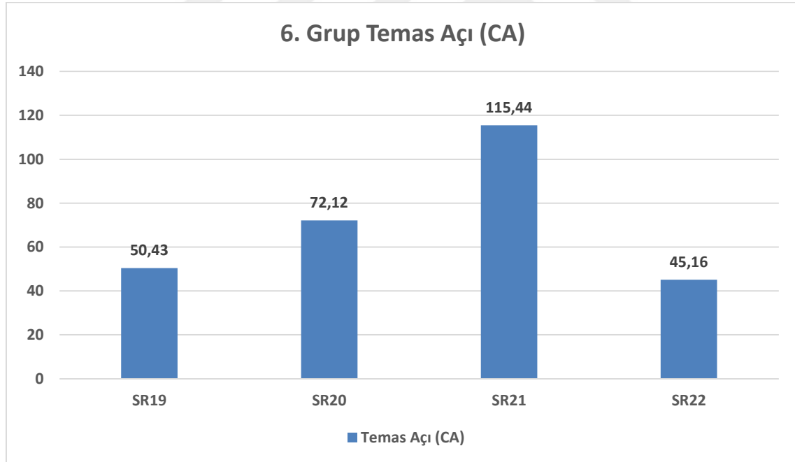
Şekil 4.15 6. Grup \text{Ce}(\text{NO}_3)_3 ve asetil asetonlu hazırlanan bileşimlerin CA değerleri.
