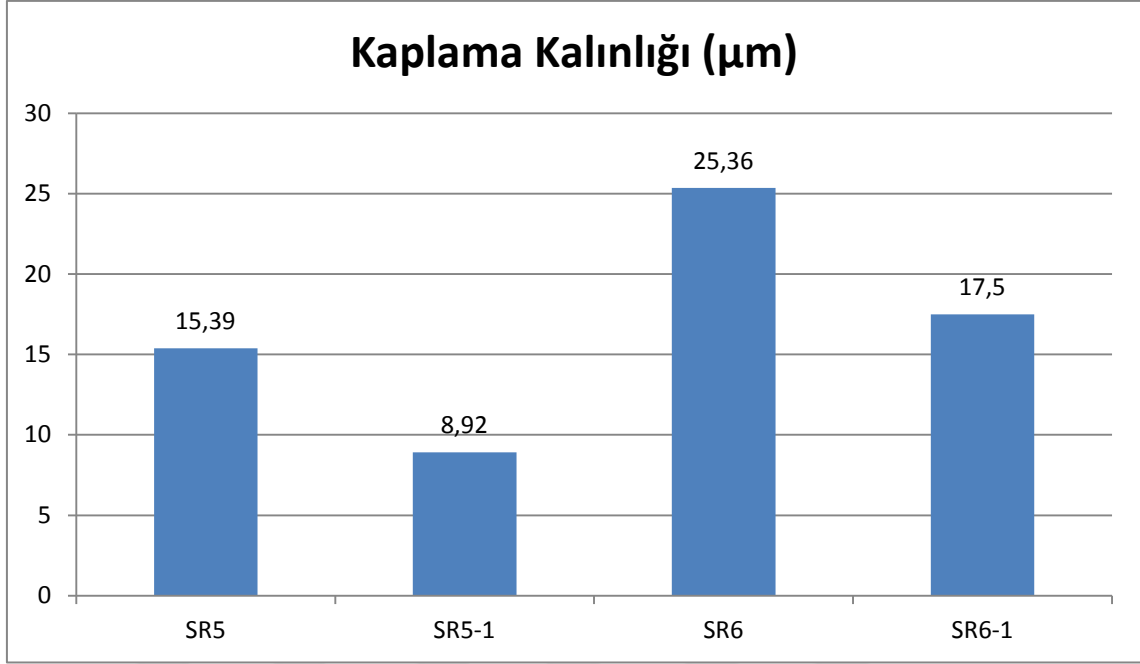
Şekil 4.27 2. Grup kolloidal silikalı hazırlanan bileşimlerin kaplama kalınlığı.
