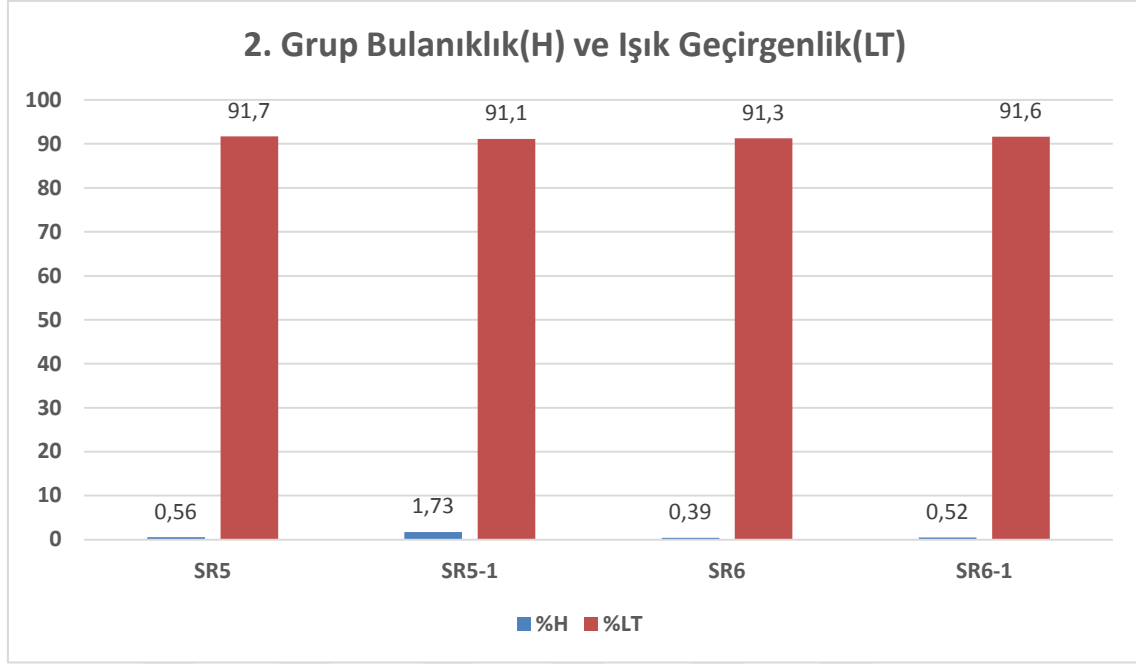
Şekil 4.3 2.Grup kolloidal silikalı hazırlanan bileşimlerin %H ve %LT değerleri.
