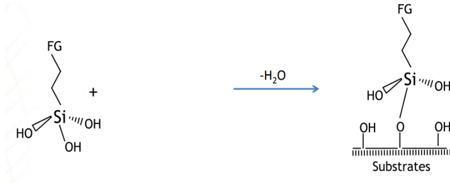
Şekil 2.16 Silanların yoğunlaşması.
