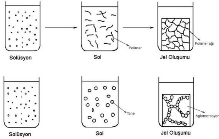
Şekil 2.6 Jelleşme mekanizması.
