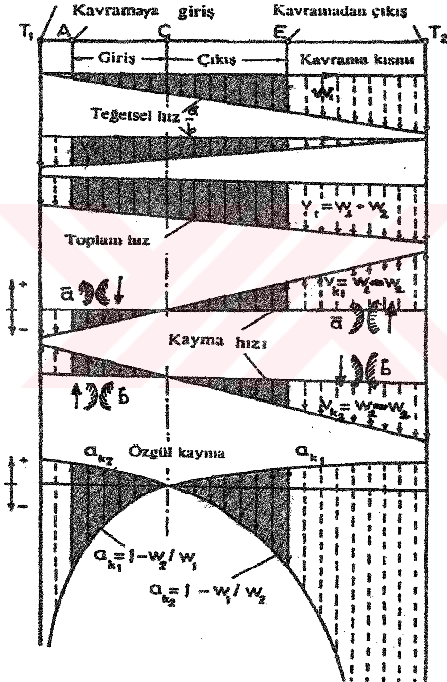
Şekil 1.8 Diş yüzeyinin temas noktalarındaki hızlarının kavrama doğrusu üzerindeki yayılımı (Hohn, Michaelis, Doleschel, 2001.)
