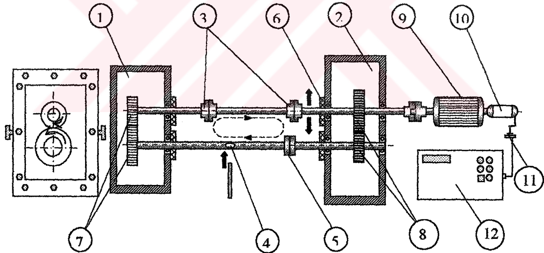
Şekil 5.2 Deney düzeneği
