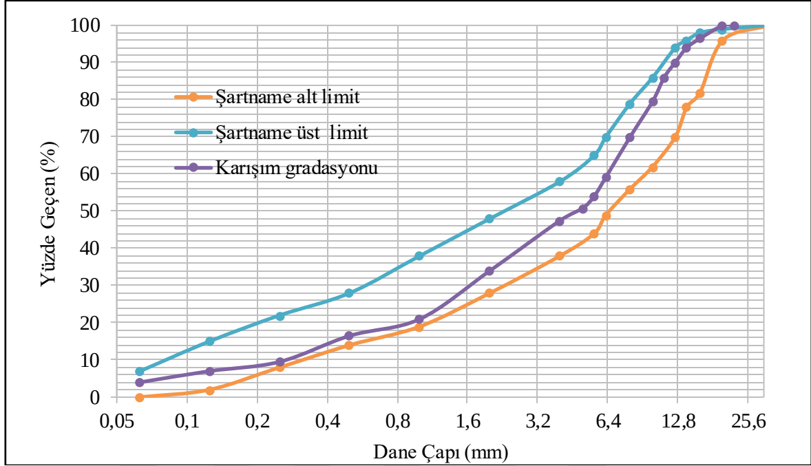
Şekil 4.2. SSB karışımı agrega gradasyonu
