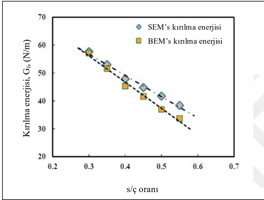
Şekil 2.4. SEM ve BEM başlangıç kırılma enerjisi s/ç oranı ilişkisi (Rahmani ve diğerleri, 2020a)
