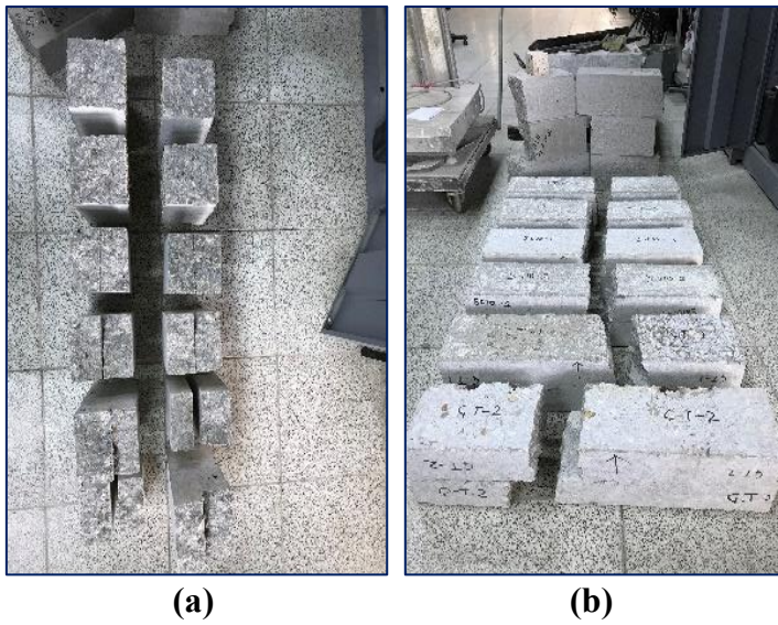
Resim 5.18. Kiriş eğilme dayanımı sonrası numuneler
