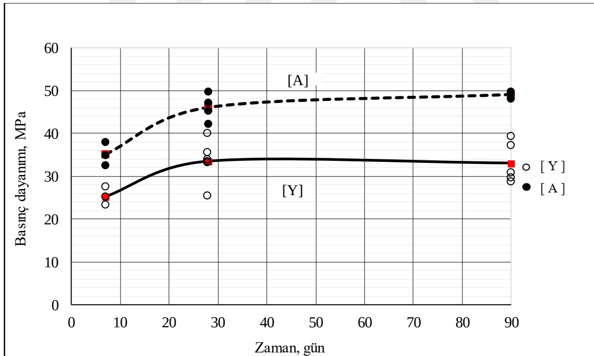
Şekil 4.13. Ara yüzey elemansız [Y] ve Aderans harcı [A] numunelerin basınç dayanımları
