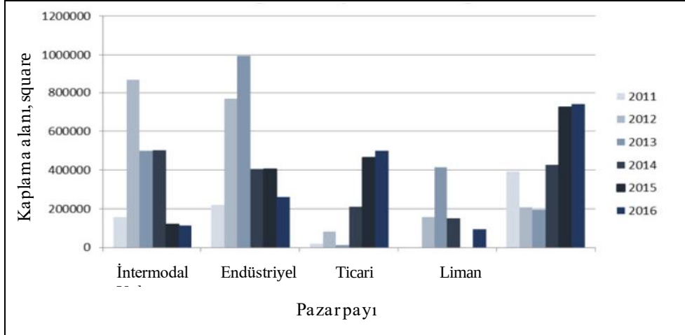
Şekil 1.1. ABD’de SSB proje büyüklüğü-kullanım alanı ilişkisi (Zollinger, 2019)
