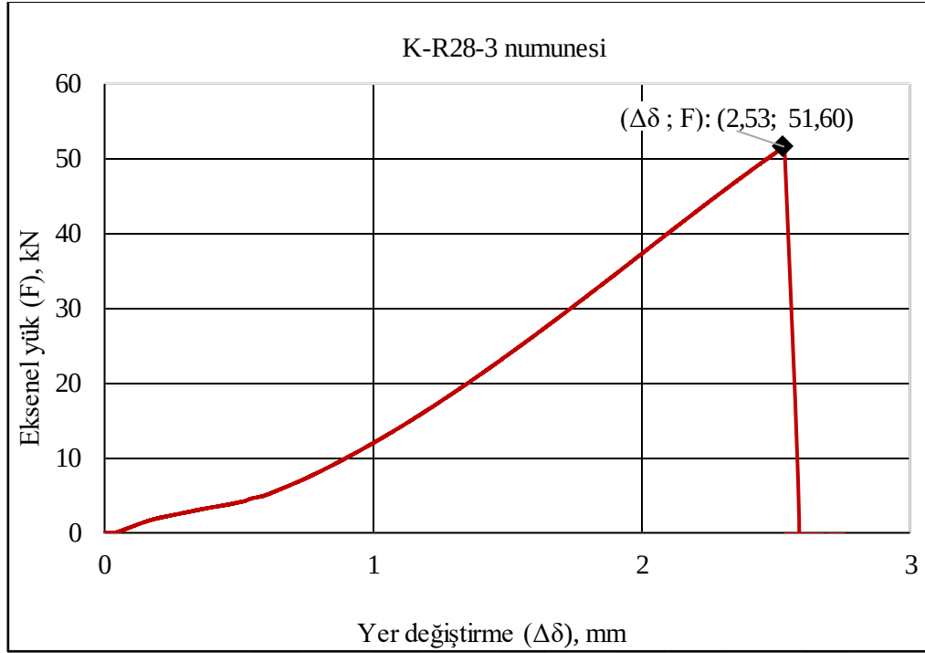
Şekil 1.3. K-R28-3 kiriş numunesi 28 günlük eksenel kuvvet-deplasman ilişkisi
