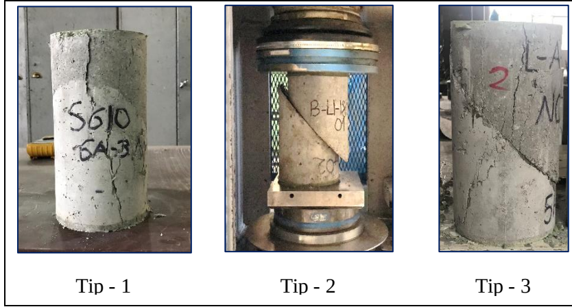
Resim 4.22. 45° eğimli ara yüzeyli silindirik numunelerin kırılma şekilleri
