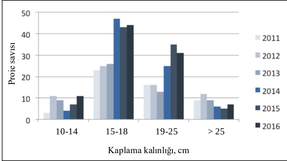
Şekil 1.2. ABD’de SSB kaplama proje sayısı - plak kalınlığı ilişkisi (Zollinger, 2019)
