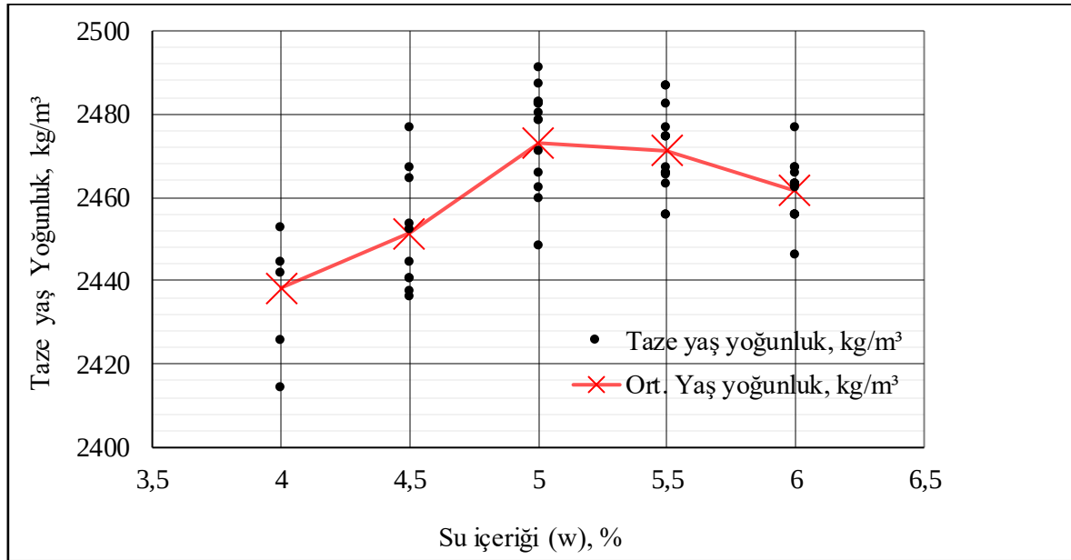
Şekil 4.3. Taze yaş yoğunluk, su içeriği ilişkisi
