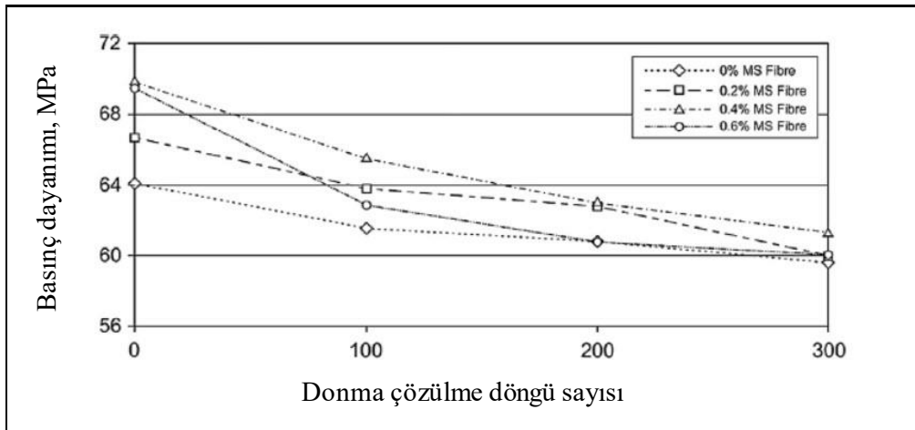
Şekil 2.5. Donma çözülme döngüsü sonrası, MS lif katkılı SSB numunelerinin basınç dayanım değerleri (Algin ve Gerginci, 2020)
