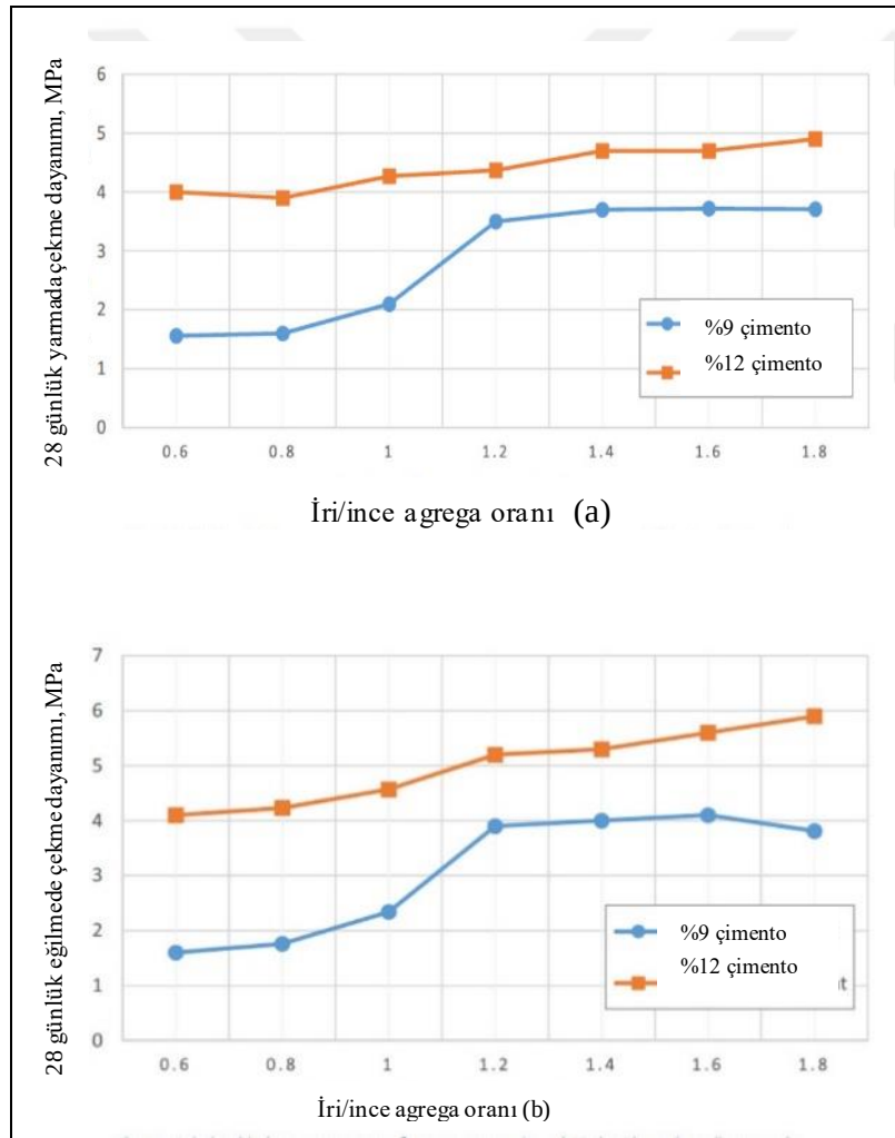
Şekil 2.2. İri/ince agrega oranı - 28 günlük (a) yarmada çekme dayanımı ve (b) eğilmede çekme dayanımı ilişkisi (Hashemi ve diğerleri, 2018)
