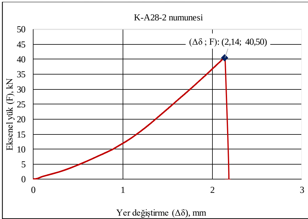
Şekil 1.18. K-A28-2 kiriş numunesi 28 günlük eksenel kuvvet-deplasman ilişkisi
