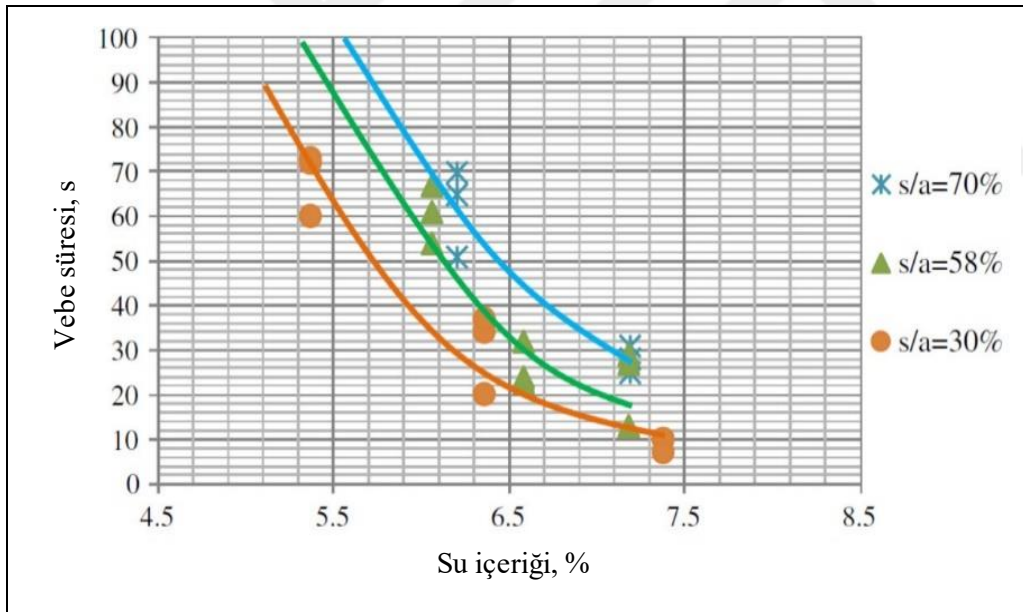
Şekil 2.1. Vebe süresi – su içeriği ve kum/agrega ( s/a=\%30,58 ve 70 ) ilişkisi (Chhorn ve diğerleri, 2017)
