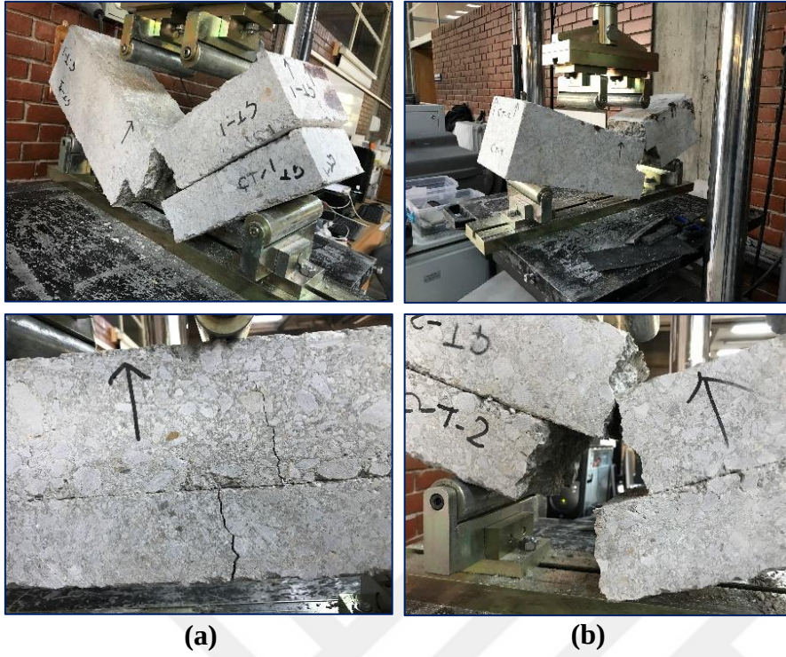
Resim 5.17. Ara yüzey elemansız iki tabaka SSB numuneleri kiriş eğilme deneyleri (a) Ç-K1 numunesi (b) Ç-K2 numunesi
