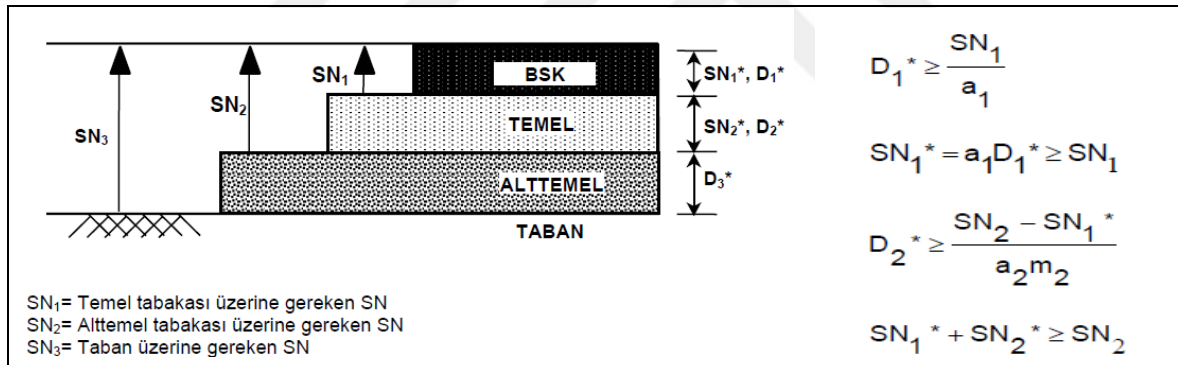
Şekil 3.1. SN ile tabaka kalınlık kontrolü (Güngör ve Sağlık, 2008)
