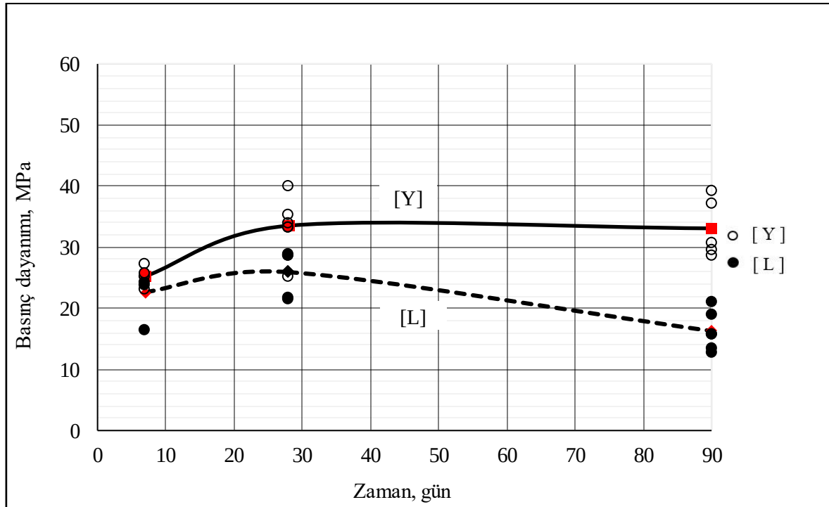
Şekil 4.11. Ara yüzey elemansız [Y] ve Lateks [L] numunelerin basınç dayanımları
