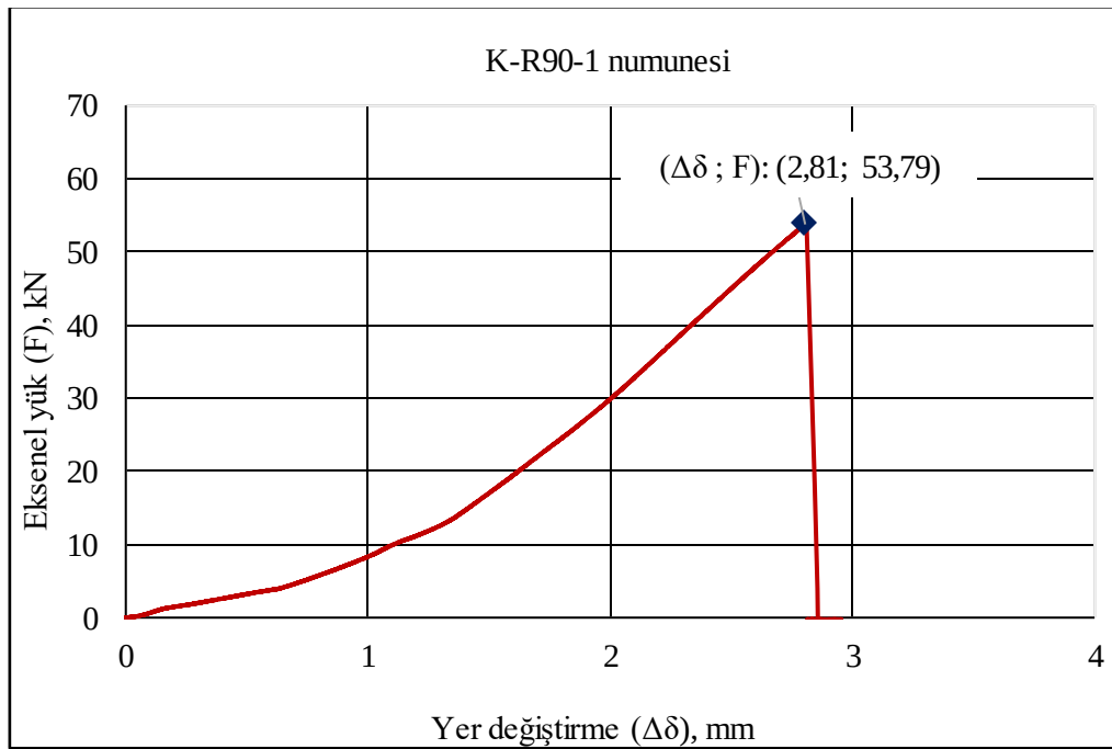
Şekil 1.6. K-R90-1 kiriş numunesi 90 günlük eksenel kuvvet-deplasman ilişkisi
