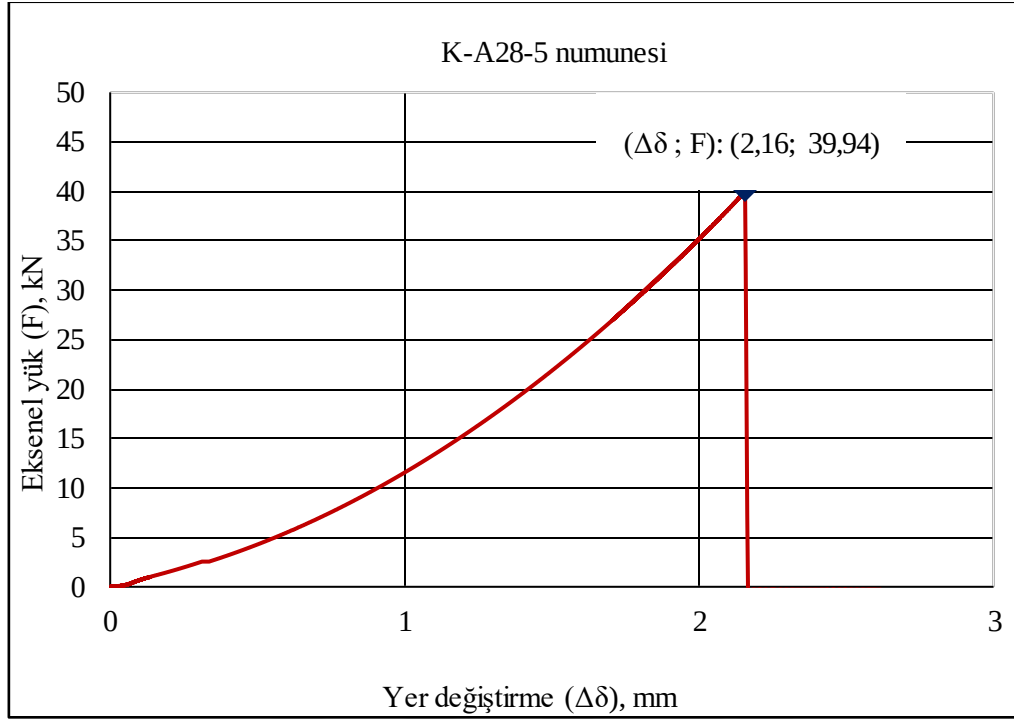
Şekil 1.21. K-A28-5 kiriş numunesi 28 günlük eksenel kuvvet-deplasman ilişkisi
