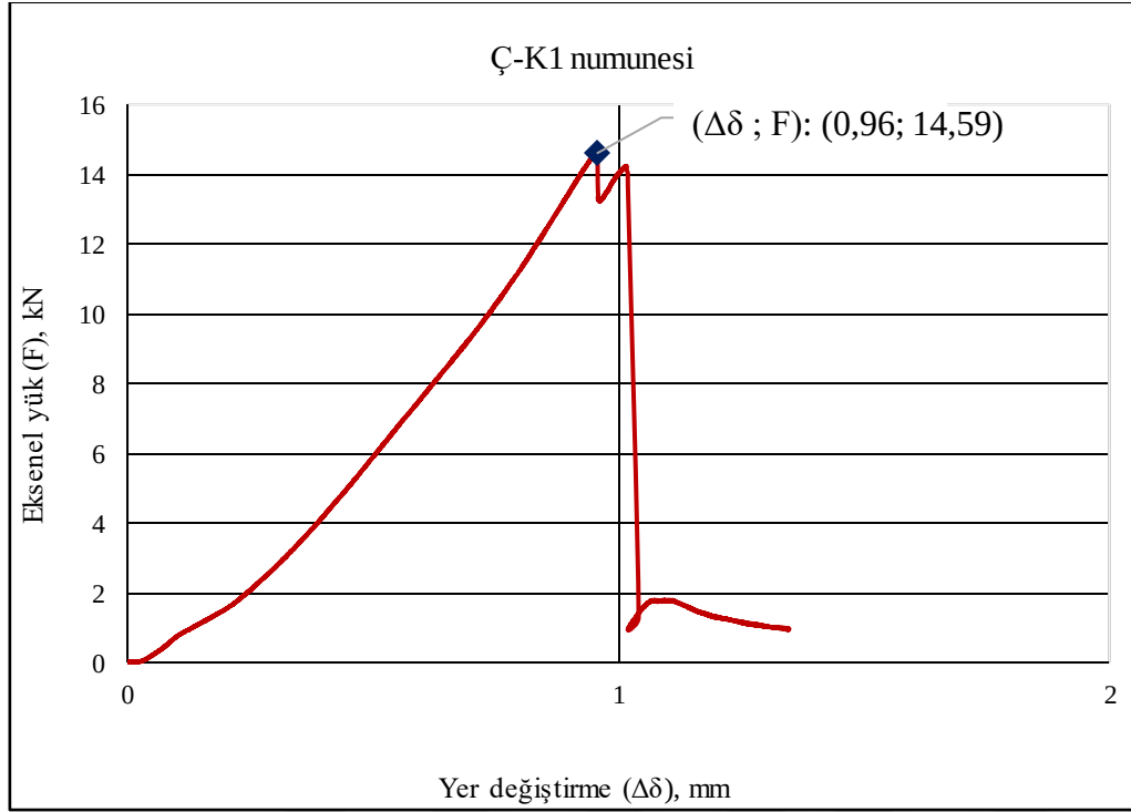
Şekil 1.27. Ç-Y-1 kiriş numunesi 313 günlük eksenel kuvvet-deplasman ilişkisi
