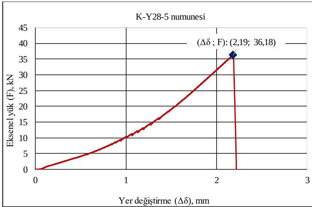
Şekil 1.16. Y-5 kiriş numunesi 28 günlük eksenel kuvvet-deplasman ilişkisi
