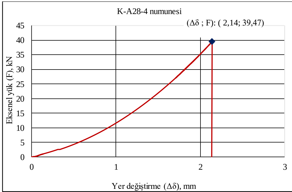
Şekil 1.20. K-A28-4 kiriş numunesi 28 günlük eksenel kuvvet-deplasman ilişkisi
