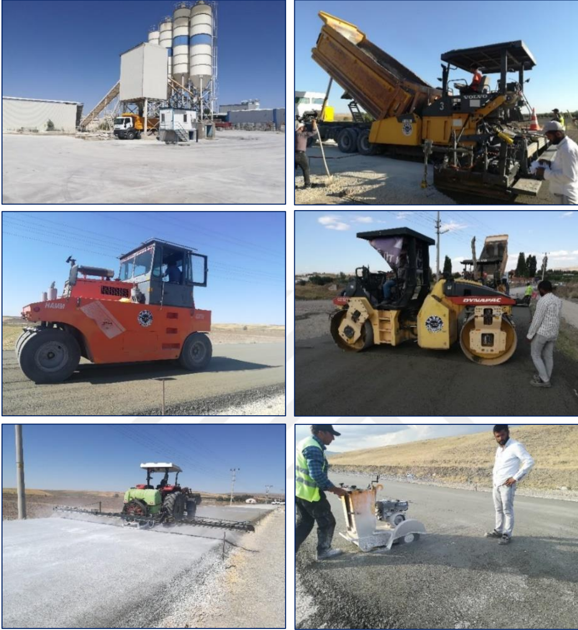
Resim 5.2. SSB uygulamasında kullanılan makina ve ekipmanlar
