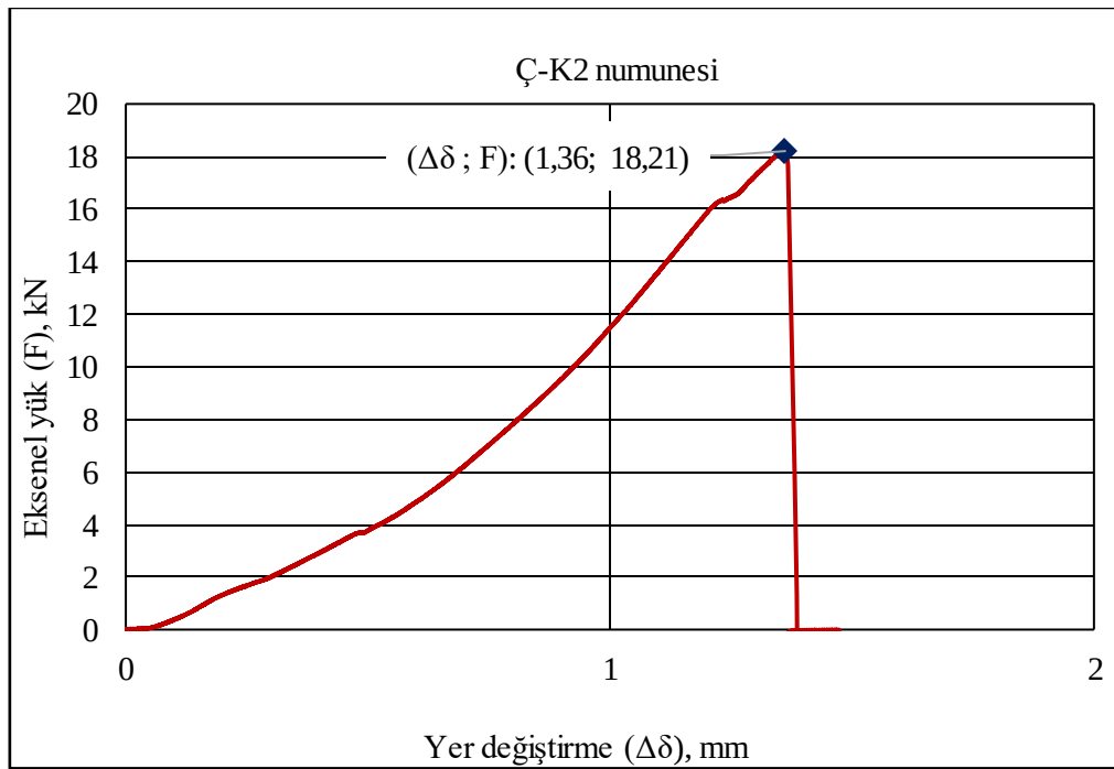
Şekil 1.28. Ç-Y-2 kiriş numunesi 313 günlük eksenel kuvvet-deplasman ilişkisi
