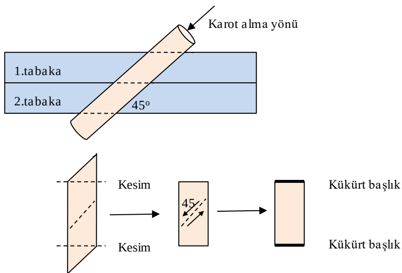
Şekil 5.2. Açılı karot numune alımı ve basınç dayanımı deneyine hazırlanmasının şematik gösterimi
