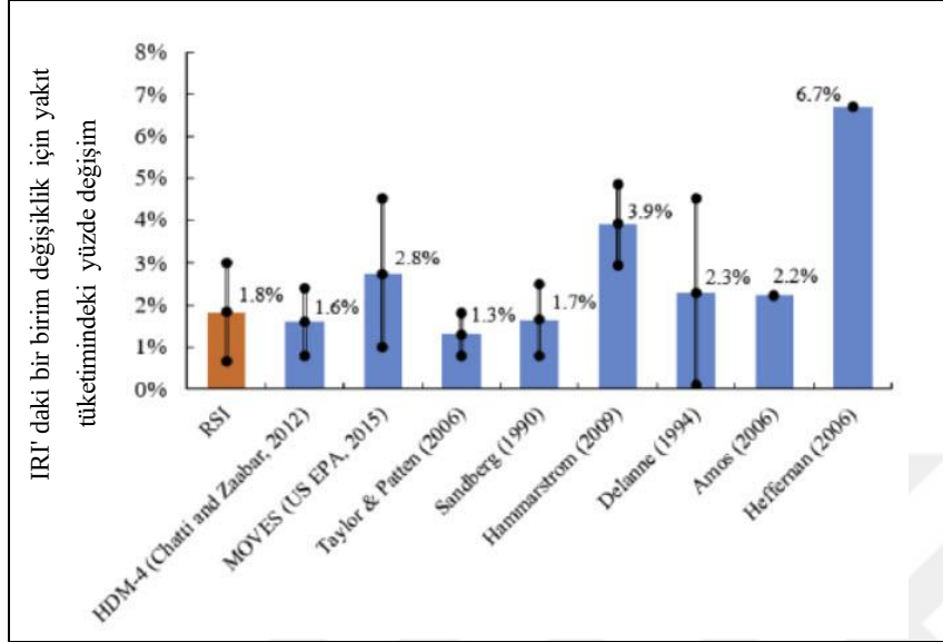
Şekil 1.3. IRI değişiminin yakıt tüketimine etkisi (Ziyadi ve diğerleri, 2017)
