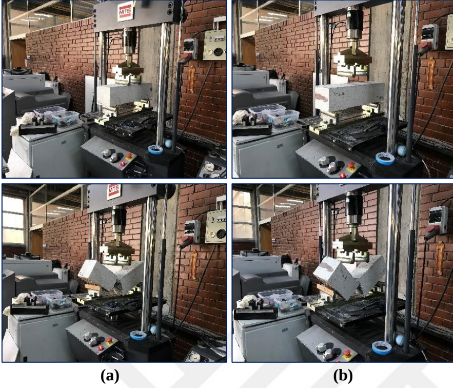
Resim 5.15. Tek tabaka SSB numuneleri kiriş eğilme deneyleri (a) T-K1 numunesi (b) T-K2 numunesi
