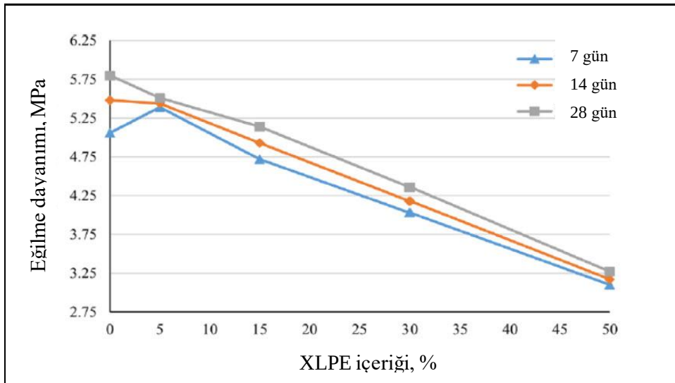
Şekil 2.9. Çapraz bağlı polietilen (XLPE) içeriği - eğilme dayanımı ilişkisi (Shamsaei ve diğerleri, 2017)
