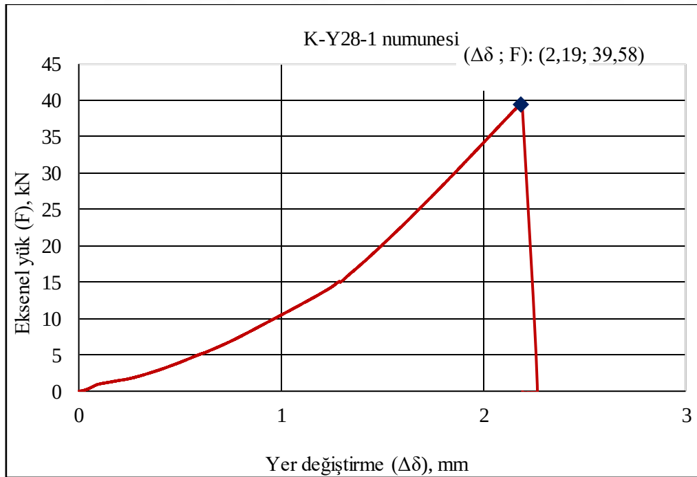
Şekil 1.12. K-Y28-1 kiriş numunesi 28 günlük eksenel kuvvet-deplasman ilişkisi
