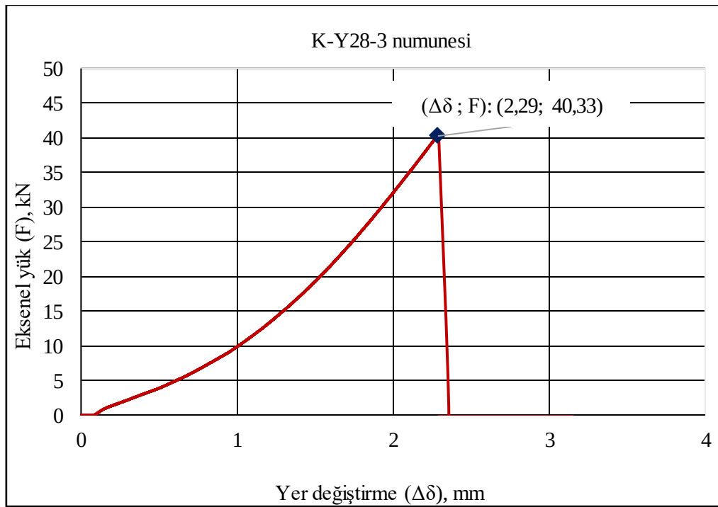
Şekil 1.14. K-Y28-3 kiriş numunesi 28 günlük eksenel kuvvet-deplasman ilişkisi
