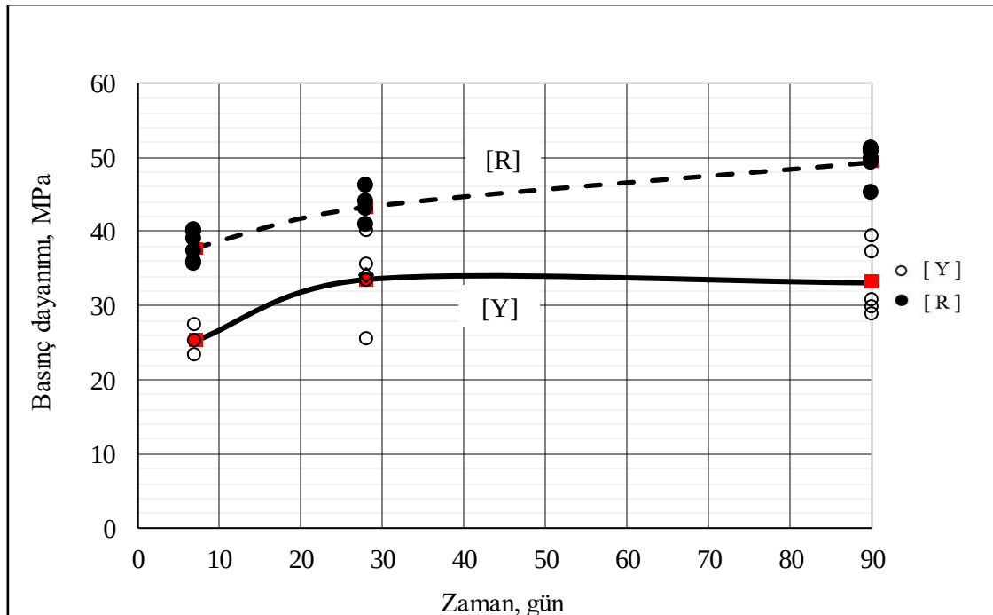
Şekil 4.16. Referans [R] ve Ara yüzey elemansız [Y] numunelerin basınç dayanımları
