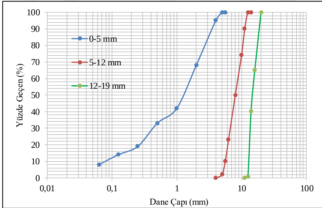
Şekil 4.1. Agrega gruplarına ait dane dağılım eğrileri
