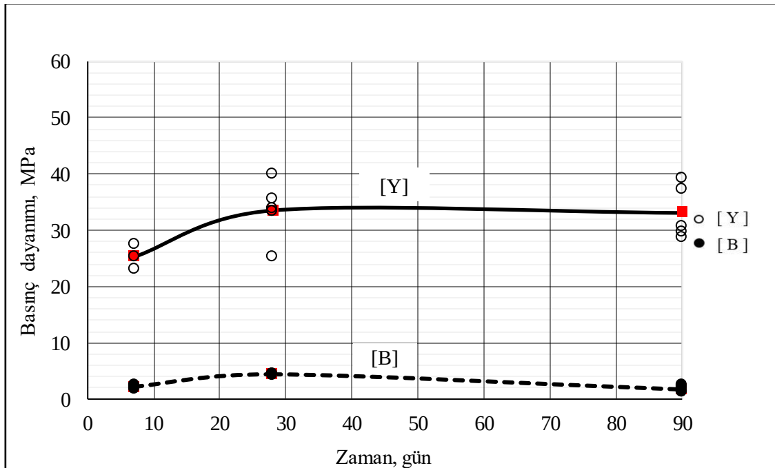
Şekil 4.14. Ara yüzey elemansız [Y] ve Bitümlü yapıştırıcı [B] numunelerin basınç dayanımları
