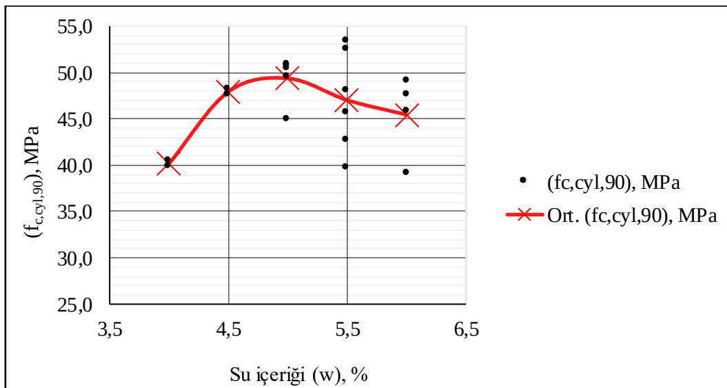
Şekil 4.8. 90 günlük basınç dayanımı su içeriği ilişkisi
