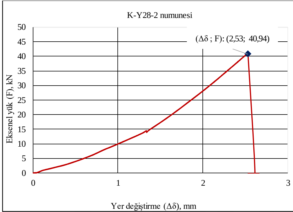
Şekil 1.13. K-Y28-2 kiriş numunesi 28 günlük eksenel kuvvet-deplasman ilişkisi
