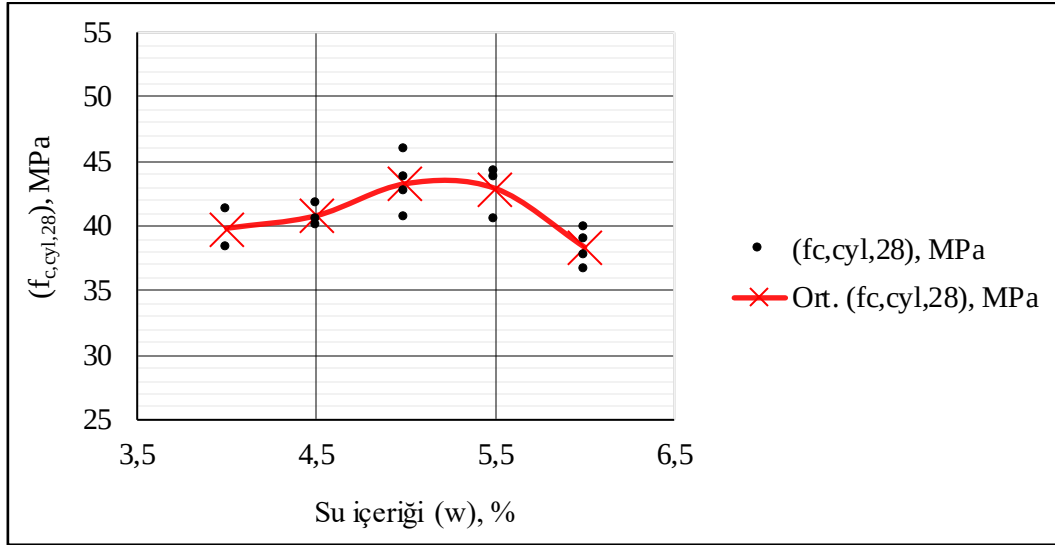
Şekil 4.7. 28 günlük basınç dayanımı su içeriği ilişkisi
