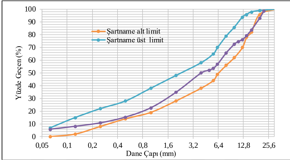
Şekil 5.1. Karışım gradasyonu ve şartname limitleri (uygulama aşaması)
