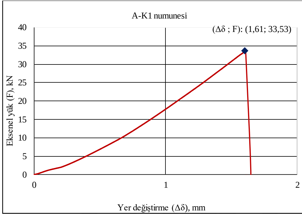
Şekil 1.25. A-K1 kiriş numunesi 313 günlük eksenel kuvvet-deplasman ilişkisi
