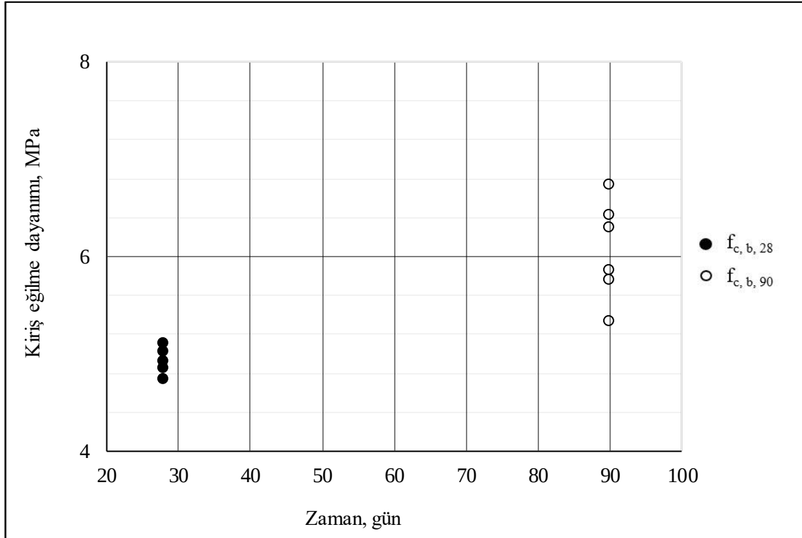
Şekil 4.19. Tek tabaka kiriş numunelerinin kür süresi kiriş eğilme dayanımı ilişkisi
