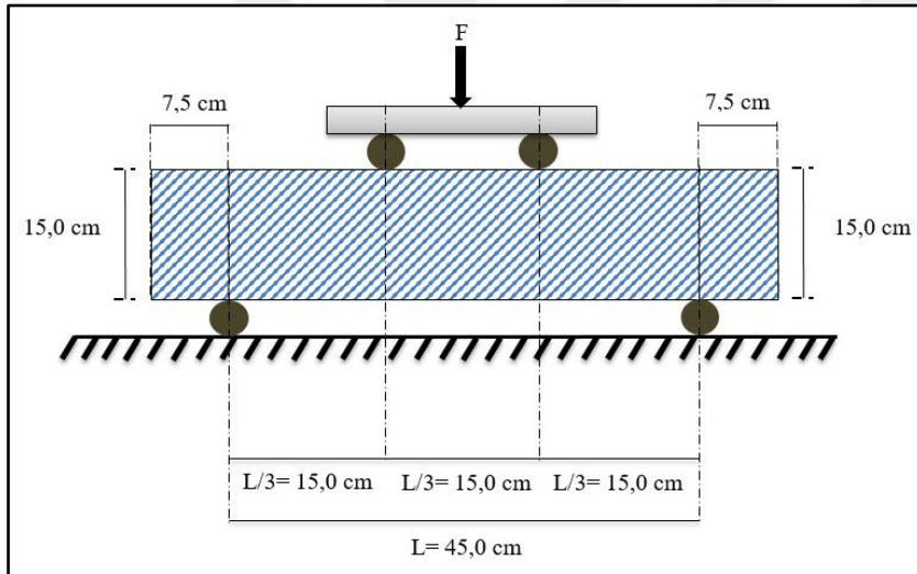
Şekil 4.18. Kiriş eğilme dayanımı deney düzeneği şematiği
