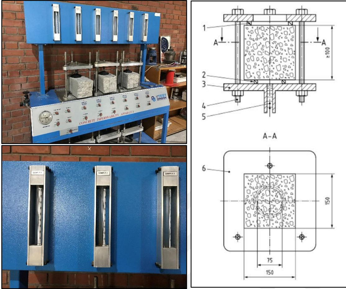
Resim 4.26. Su işleme derinliği tayini deneyi cihazı
