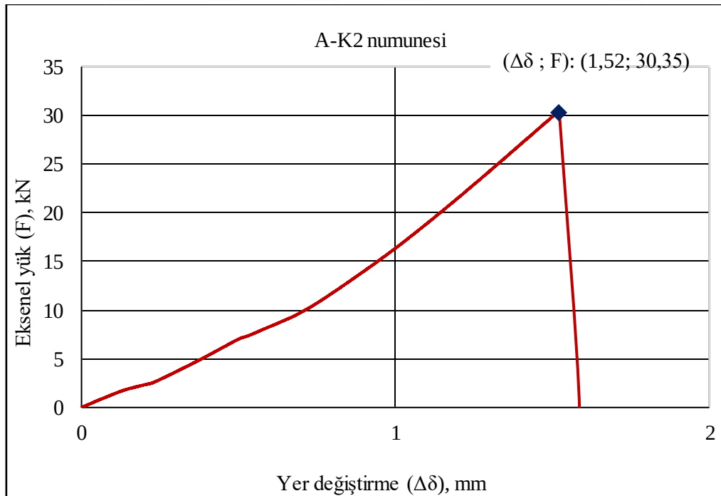
Şekil 1.26. Ç-A-2 kiriş numunesi 313 günlük eksenel kuvvet-deplasman ilişkisi
