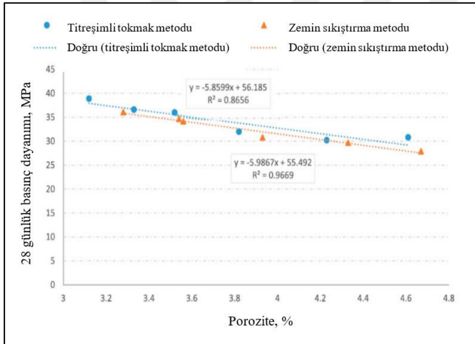
Şekil 2.3. 28 günlük basınç dayanımı ve porozite ilişkisi (Shafigh ve diğerleri, 2019)
