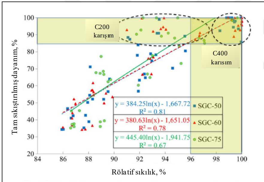
Şekil 2.8. Nominal basınç dayanımı – rölatif sıkılık ilişkisi (Shabani ve diğerleri, 2021)
