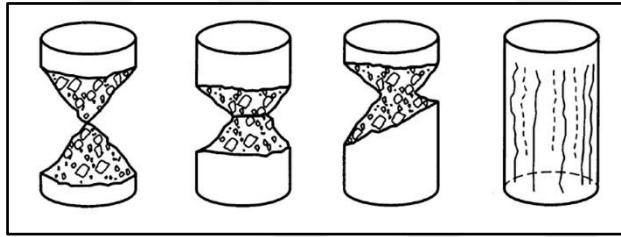
Şekil 4.17. Silindir numunelerin kabul edilebilir kırılma şekilleri (TS EN 12390-3, 2019)
