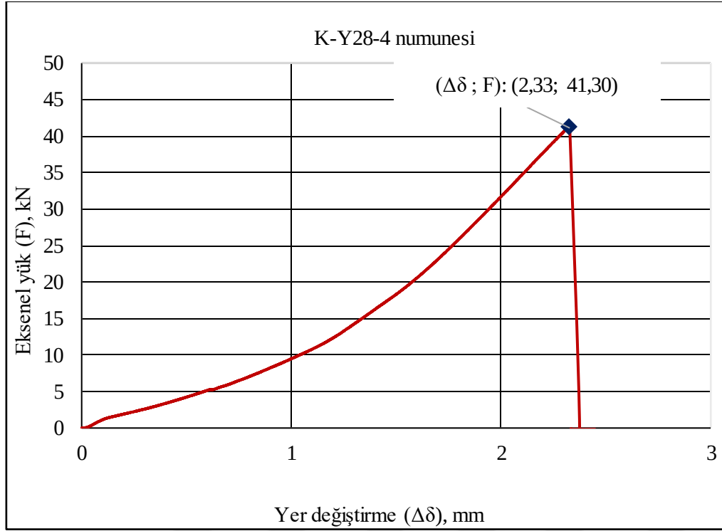
Şekil 1.15. K-Y28-4 kiriş numunesi 28 günlük eksenel kuvvet-deplasman ilişkisi
