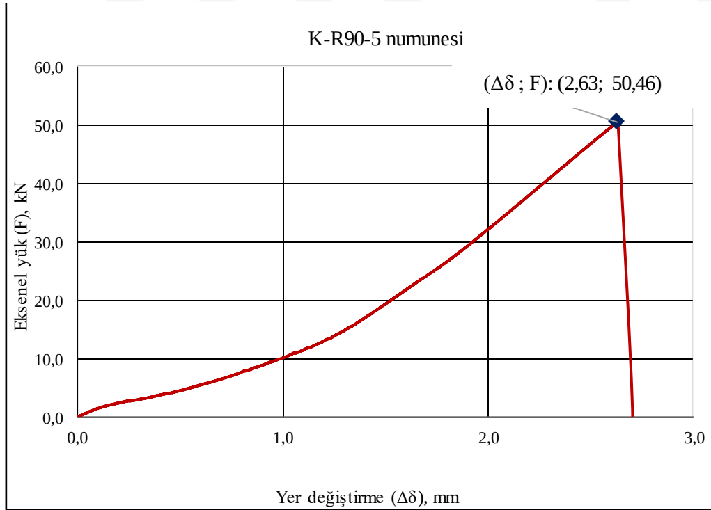
Şekil 1.10. K-R90-5 kiriş numunesi 90 günlük eksenel kuvvet-deplasman ilişkisi
