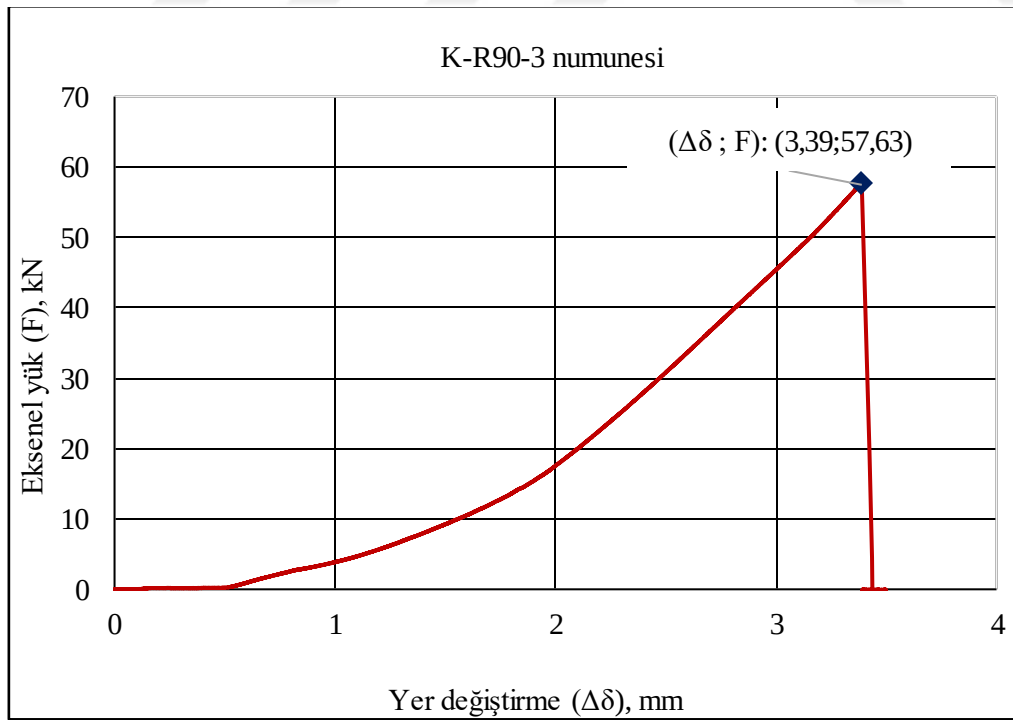
Şekil 1.8. K-R90-3 kiriş numunesi 90 günlük eksenel kuvvet-deplasman ilişkisi
