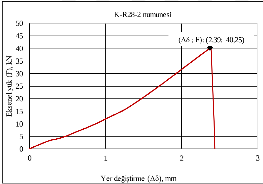
Şekil 1.2. K-R28-2 kiriş numunesi 28 günlük eksenel kuvvet-deplasman ilişkisi
