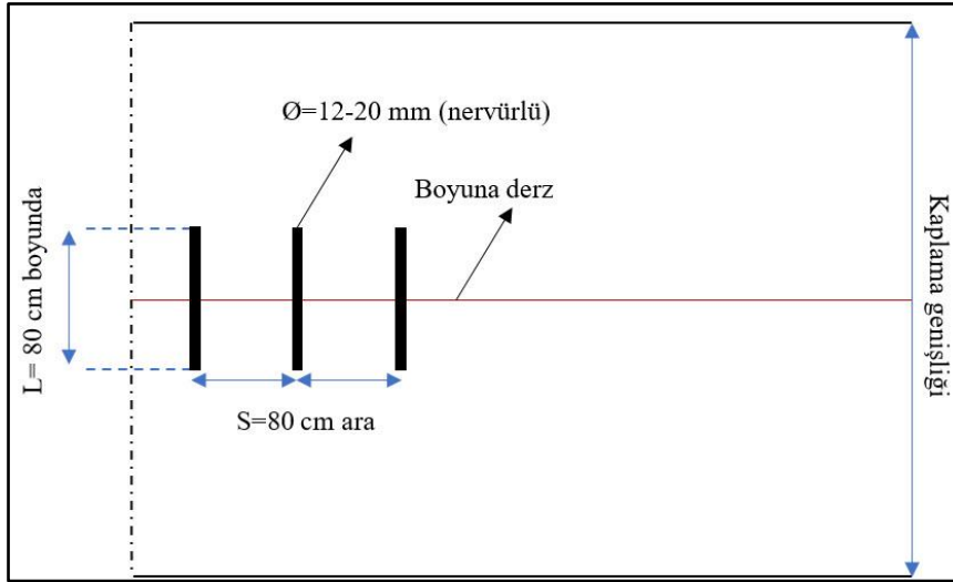
Şekil 3.3. Bağ demiri yerleşimi (Komut ve Kaşak, 2019)
