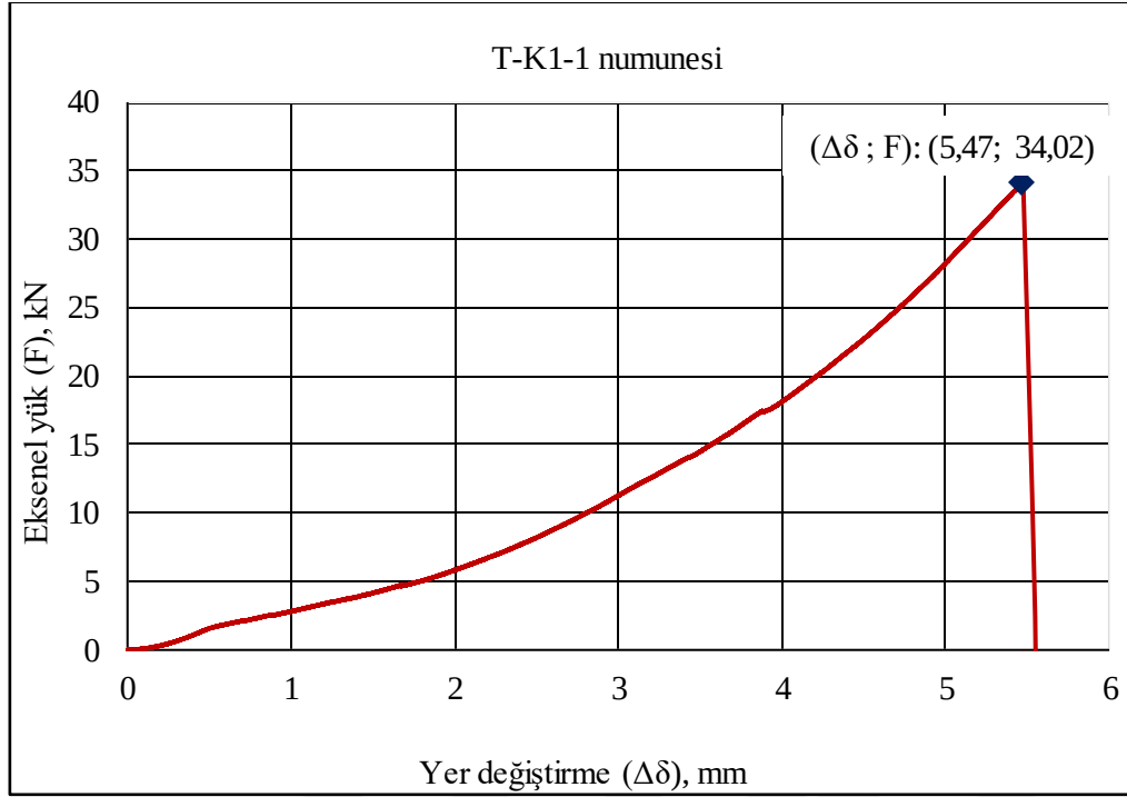
Şekil 1.23. T-K1 kiriş numunesi 313 günlük eksenel kuvvet-deplasman ilişkisi
