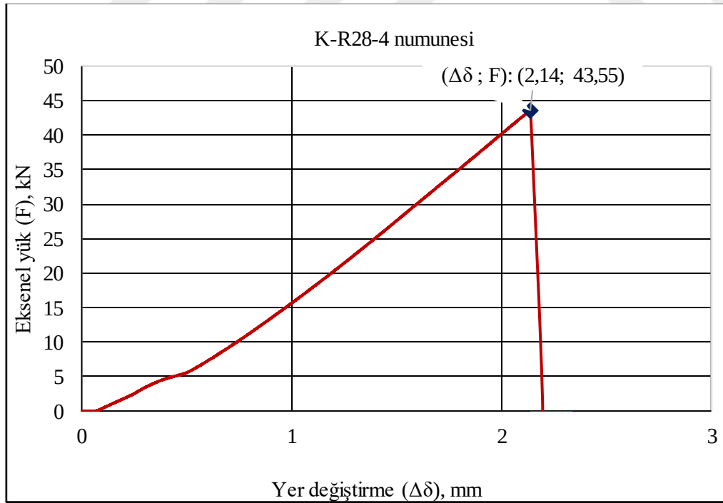
Şekil 1.4. K-R28-4 kiriş numunesi 28 günlük eksenel kuvvet-deplasman ilişkisi
