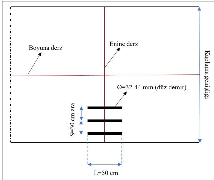
Şekil 3.2. Kayma demiri yerleşimi (Komut ve Kaşak, 2019)
