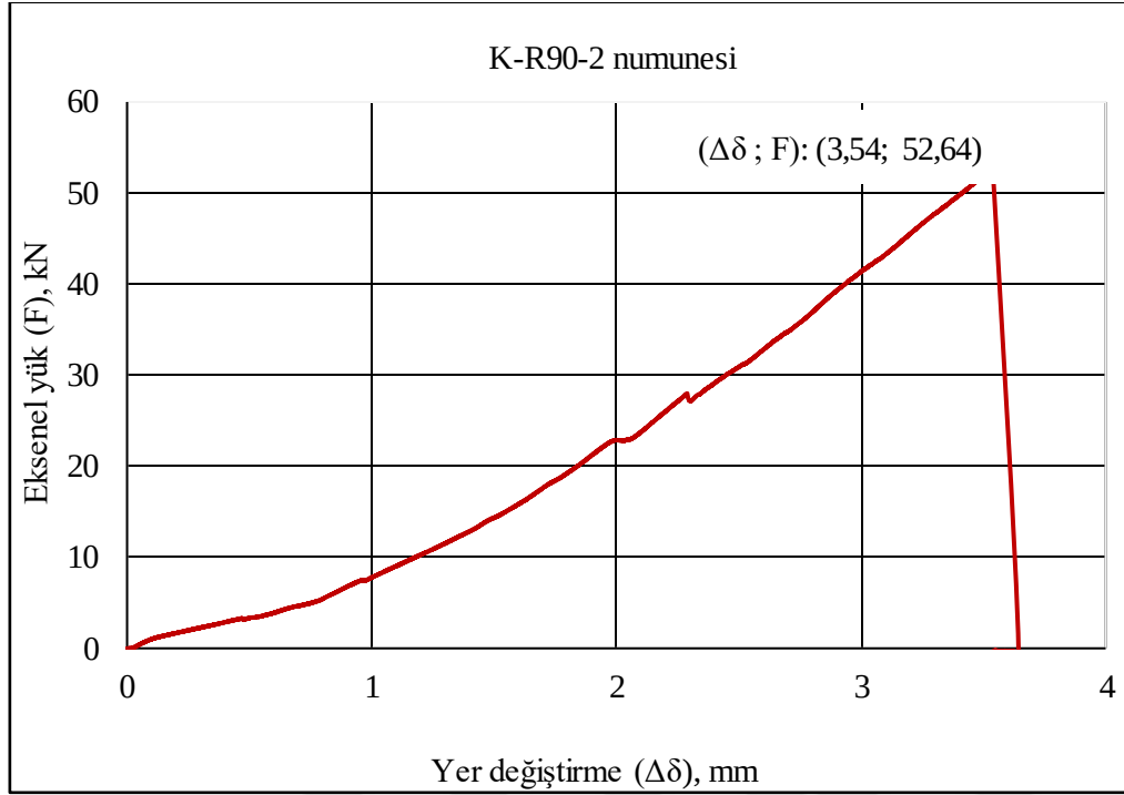
Şekil 1.7. K-R90-2 kiriş numunesi 90 günlük eksenel kuvvet-deplasman ilişkisi
