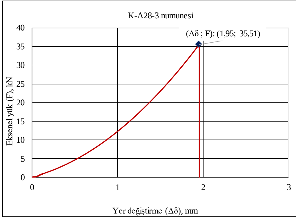
Şekil 1.19. K-A28-3 kiriş numunesi 28 günlük eksenel kuvvet-deplasman ilişkisi
