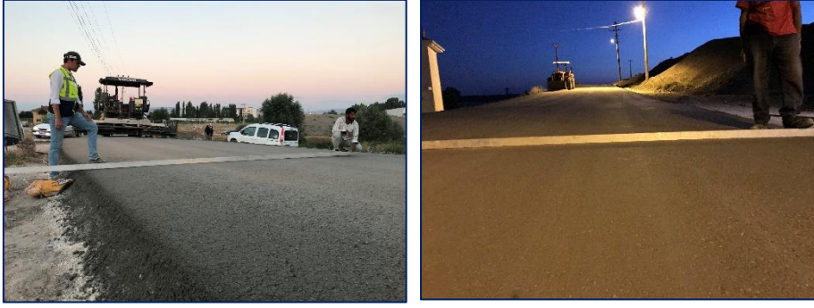
Resim 5.8. Yol düzgünlüğünün 5 m'lik masterla ölçümü
