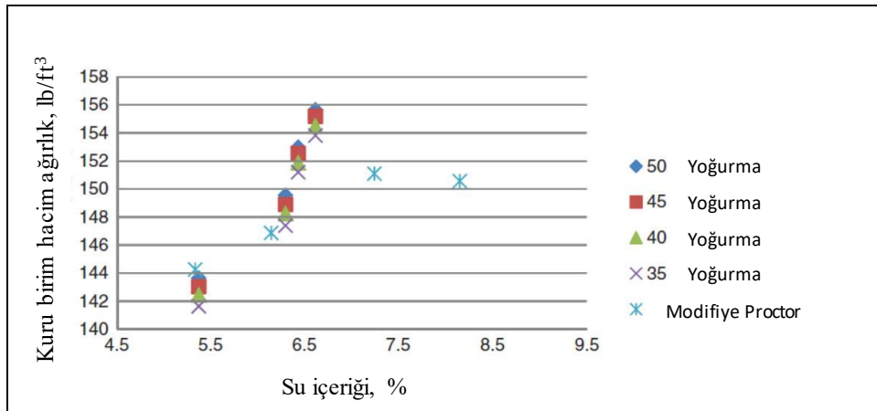
Şekil 2.6. Proctor ve yoğurmalı sıkıştırma (çeşitli yoğurma sayıları için) metodları, su içeriği – yoğunluk ilişkisi (Williams, 2013)
