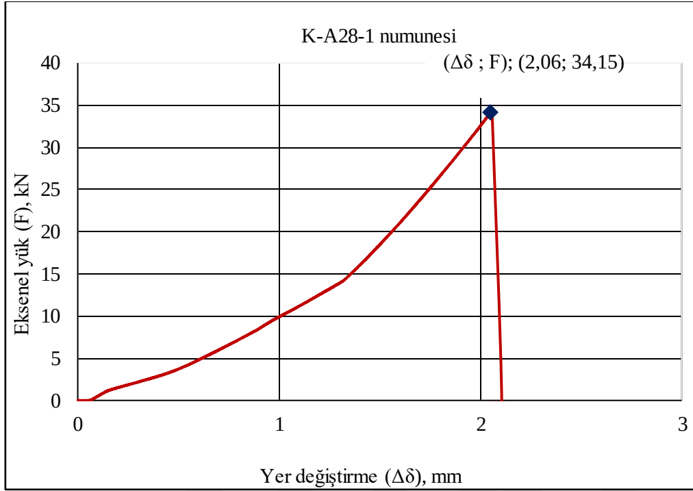
Şekil 1.17. K-A28-1 kiriş numunesi 28 günlük eksenel kuvvet-deplasman ilişkisi
