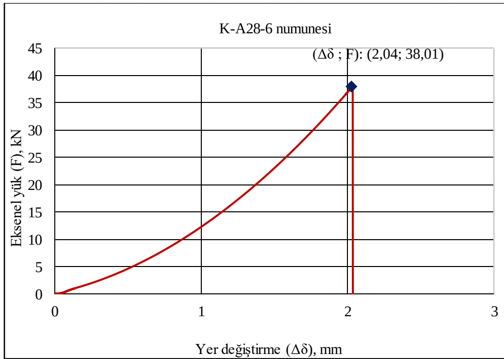
Şekil 1.22. K-A28-6 kiriş numunesi 28 günlük eksenel kuvvet-deplasman ilişkisi
