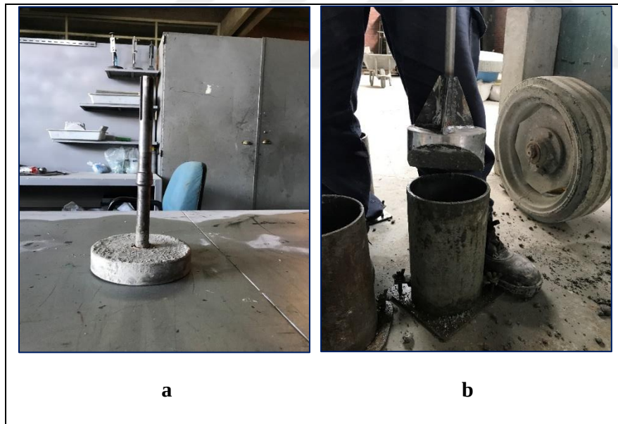
Resim 4.15. Titreşimli tokmak başlıkları
