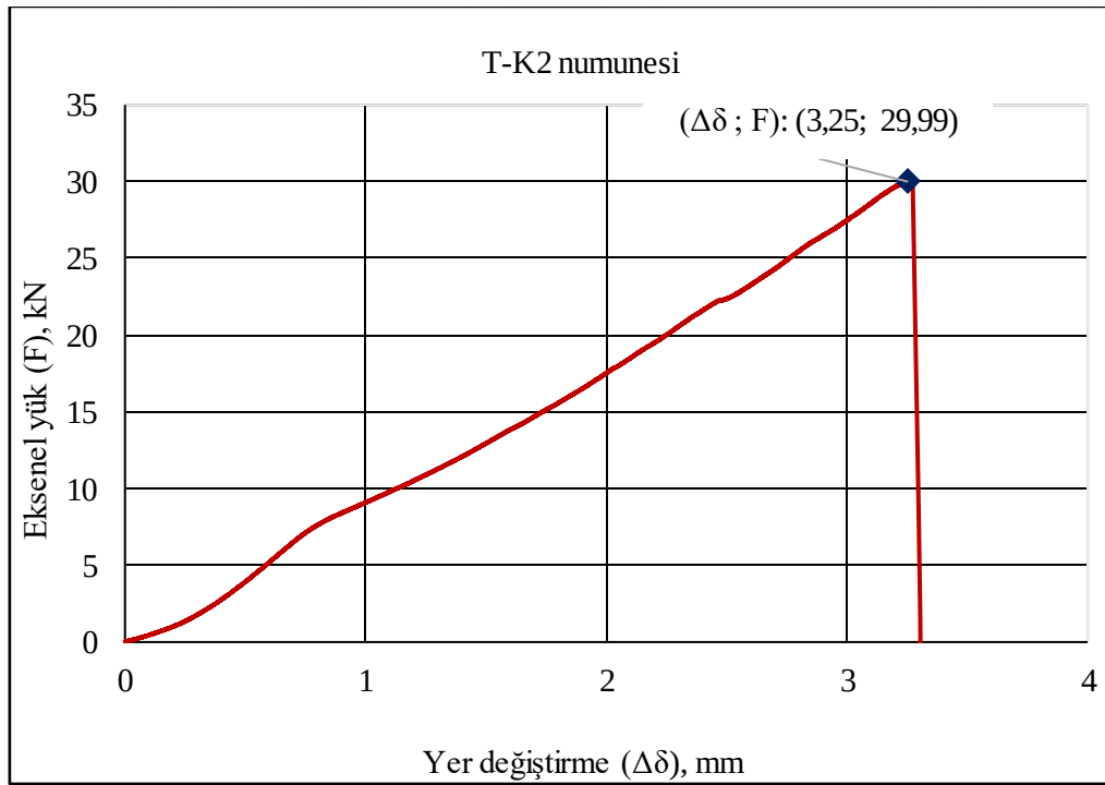
Şekil 1.24. T-K2 kiriş numunesi 313 günlük eksenel kuvvet-deplasman ilişkisi
