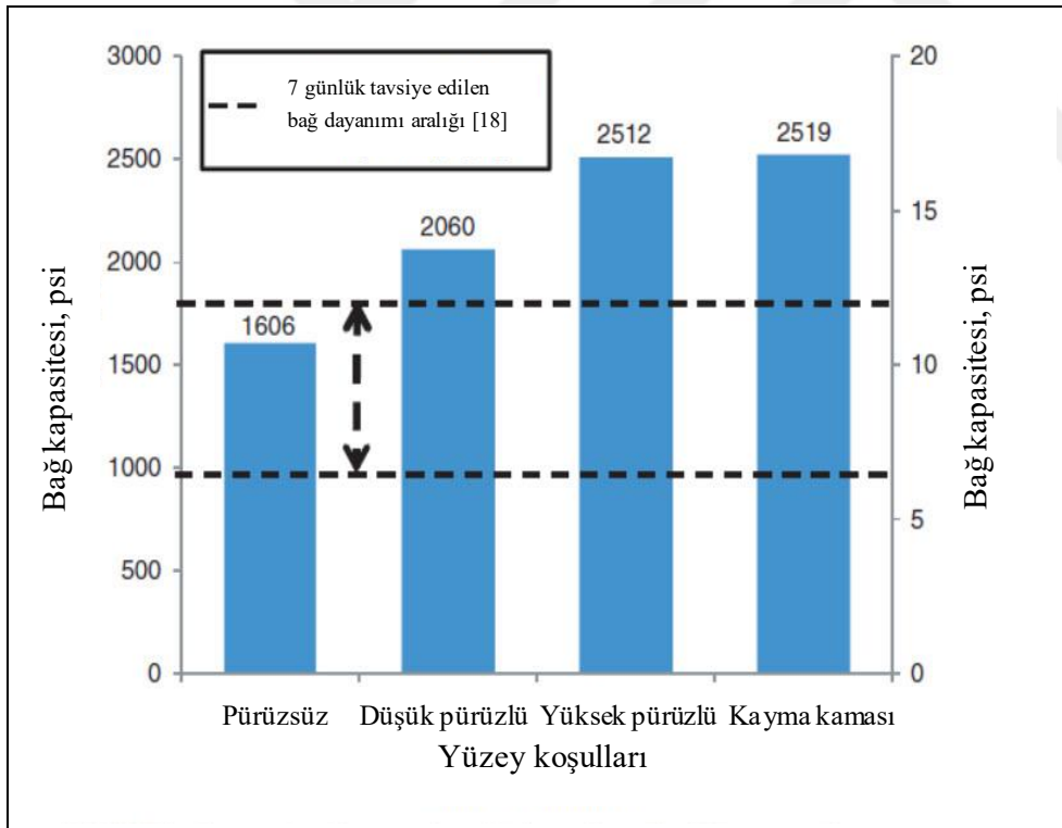
Şekil 2.11. Farklı yüzey dokularında 10 günlük ortalama bağ dayanımı (Harris ve diğerleri, 2011)
