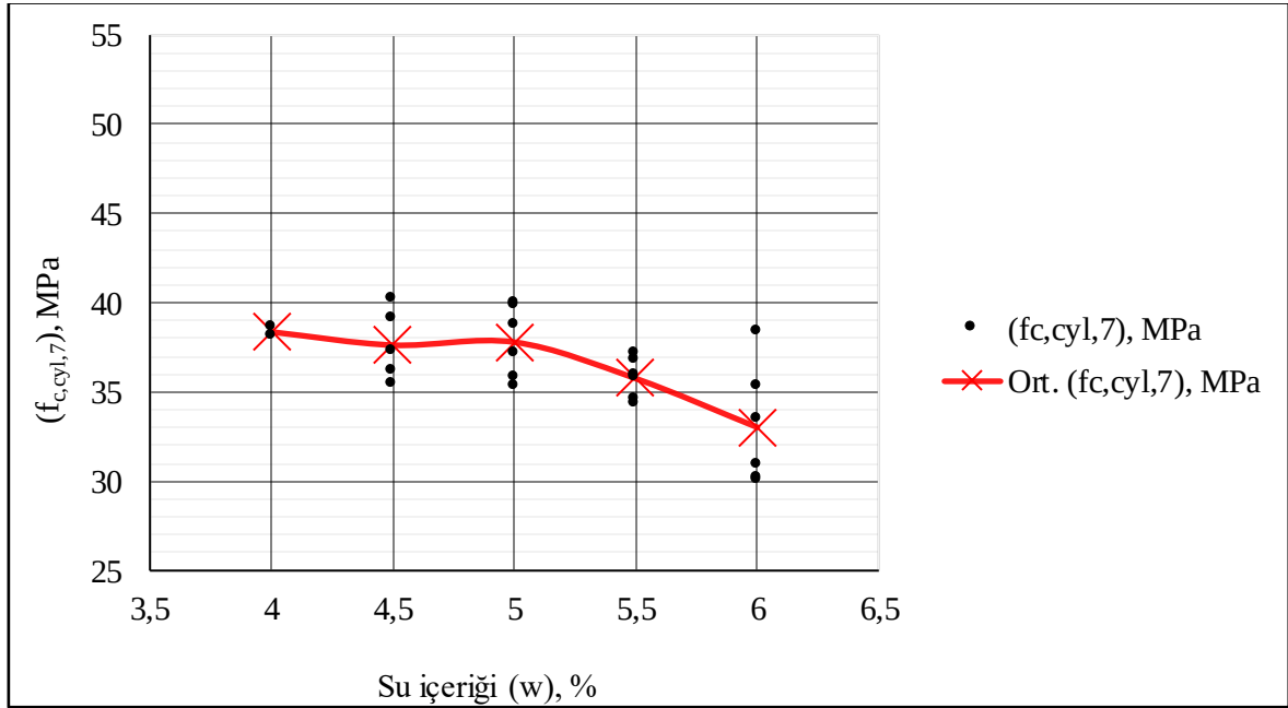
Şekil 4.6. 7 günlük basınç dayanımı su içeriği ilişkisi
