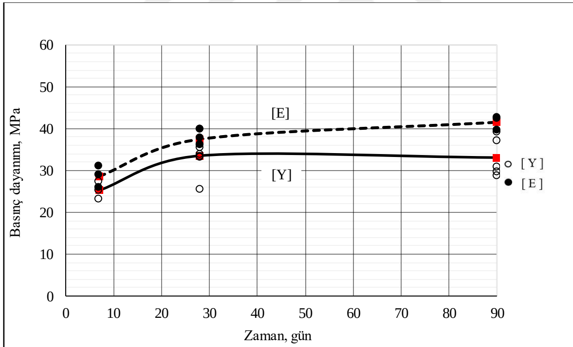
Şekil 4.12. Ara yüzey elemansız [Y] ve Epoksi reçine [E] numunelerin basınç dayanımları
