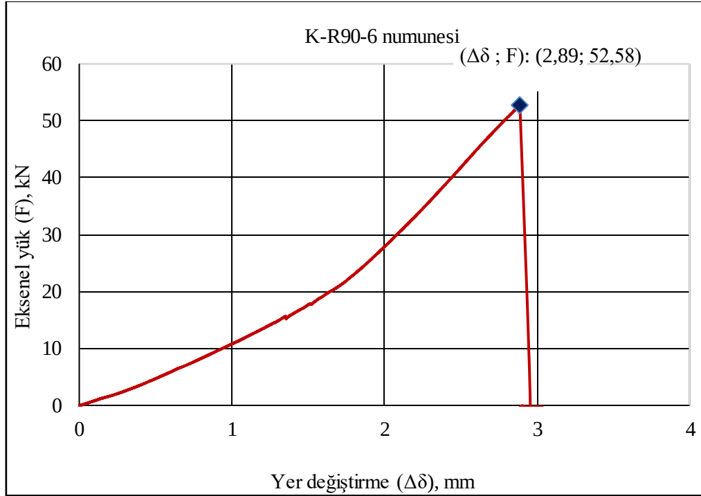
Şekil 1.11. K-R90-6 kiriş numunesi 90 günlük eksenel kuvvet-deplasman ilişkisi
