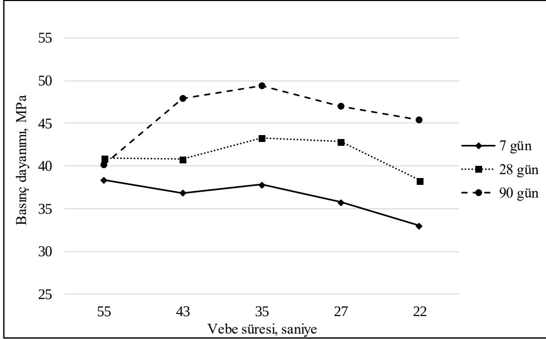
Şekil 4.9. Vebe süresi – basınç dayanımı ilişkisi
