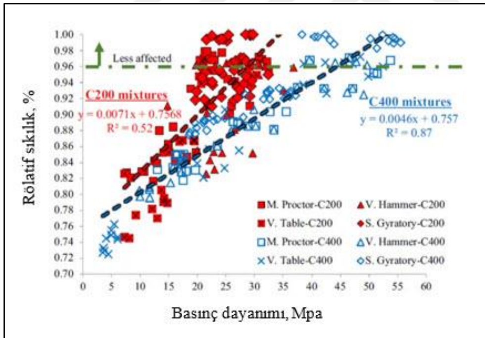
Şekil 2.7. Basınç dayanımı – rölatif sıklık ilişkisi ( 200 \text{ kg/m}^3 ve 400 \text{ kg/m}^3 çimento dozajları için) (Şengün ve diğerleri, 2019)
