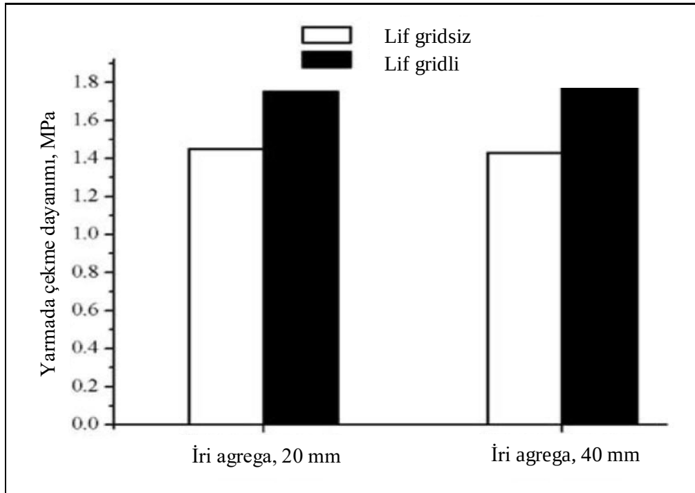
Şekil 2.10. İri agreg boyutunun yarmada çekme dayanımına etkisi (Yan ve diğerleri, 2014)
