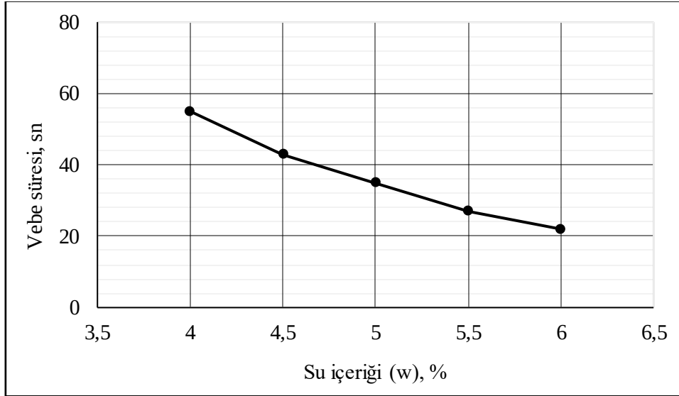
Şekil 4.5. Farklı su içeriğinde hazırlanan karışımların Vebe süreleri
