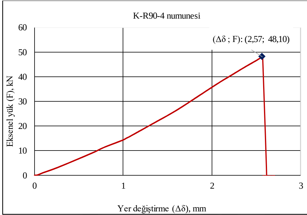
Şekil 1.9. K-R90-4 kiriş numunesi 90 günlük eksenel kuvvet-deplasman ilişkisi
