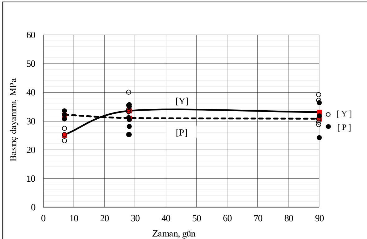
Şekil 4.15. Ara yüzey elemansız [Y] ve Pürüzlü yüzey [P] numunelerin basınç dayanımları
