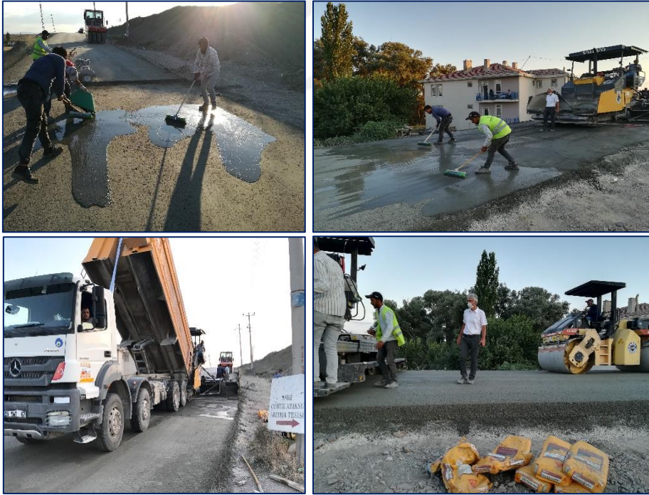
Resim 5.4. Aderans harcı uygulaması ve ikinci tabaka SSB serimi
