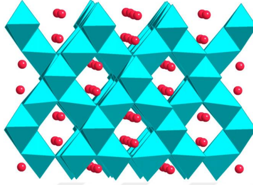
Şekil 2.3. Spinel \text{LiMn}_2\text{O}_4 yapısı [31].
