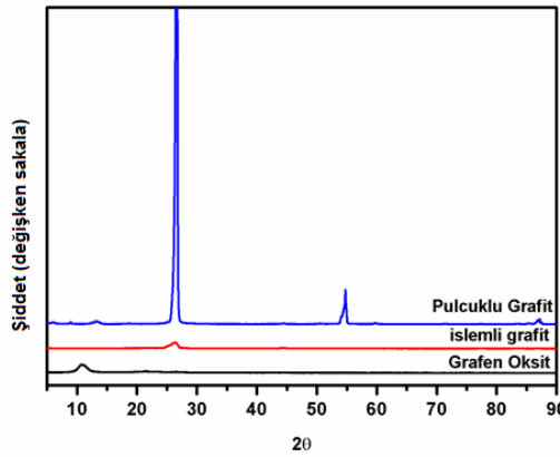
Şekil 7.2. Pulcuklu grafit, ön işlemlı grafit ve grafen oksitin X-ışınları desenleri.
