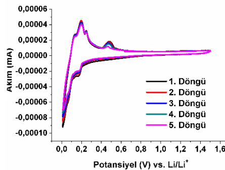
Şekil 7.11. Silisyum yumurta sarısı/kabuk elektrotlarından elde edilmiş çevrimsel voltametri sonuçları.
