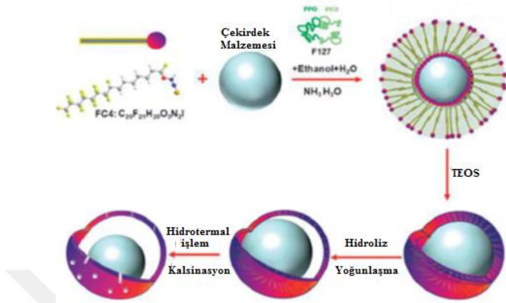
Şekil 4.2. Yüzey aktif madde kullanılarak yumurta sarısı/kabuk nanopartikül sentezi [76].
