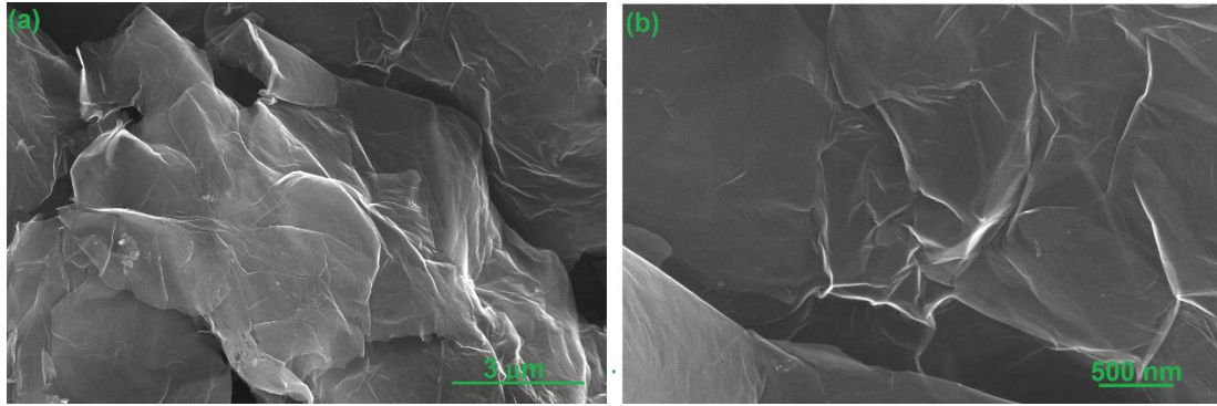
Şekil 7.5. Çok katmanlı grafinin yüzeyine ait farklı büyütmelerde FESEM görüntüleri.
