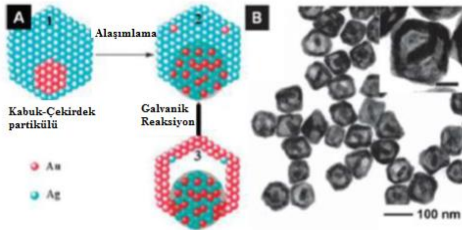
Şekil 4.5. Galvanik yer değiştirme yöntemi [83].
