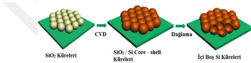
Şekil 5.5. Silisyum içi boş kürelerinin şematik gösterimi [109].
