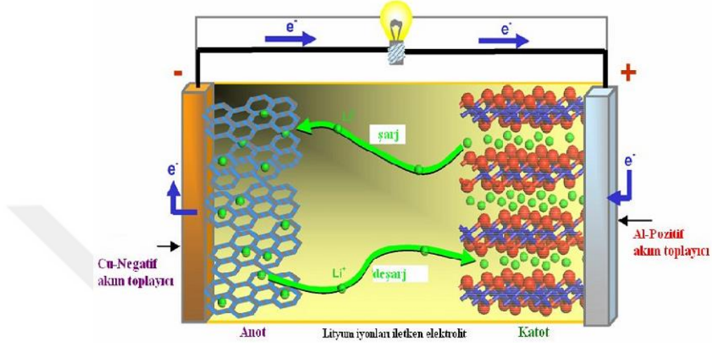
Şekil 2.1. Li iyon pillerin çalışma prensibi [25].
