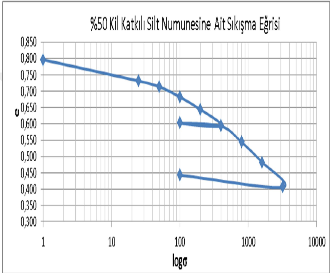
Şekil 5.24. %50 kil katkı silt numunesine ait sıkışma eğrisi
