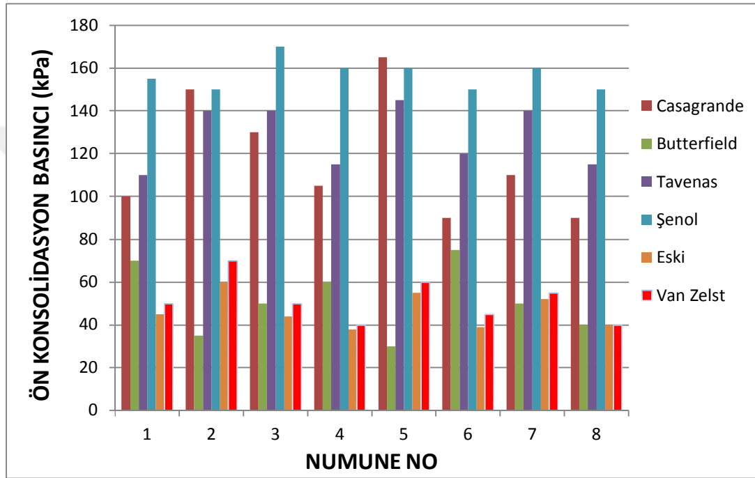
Şekil 5.34. Ön konsolidasyon basıncı değerlerinin farklı yöntemlere göre grafiksel gösterimi
