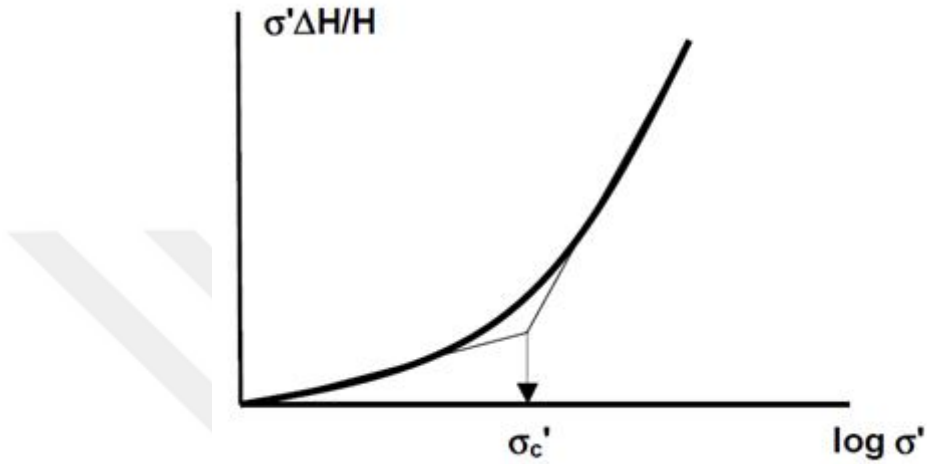
Şekil 3.18. Şenol yöntemi ile ön konsolidasyon basıncının belirlenmesi [21]
