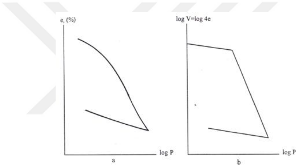
Şekil 3.12. Mexico-City kiline ait bir çalışma [16]
