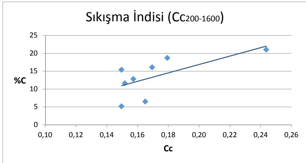
Şekil 5.27. Numunelerin sıkışma indisi değerlerinin kil oranı ile değişimi
