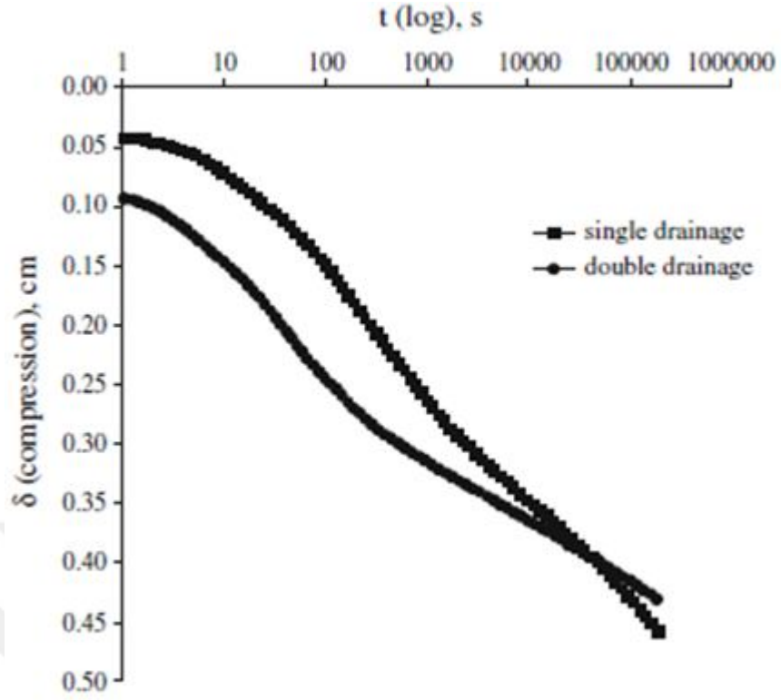
Şekil 4.3. Adapazari silt için zaman - sıkıştırma eğrileri ( r = 100-200 kPa) [24]
