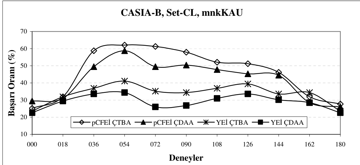
Şekil 3.33. Yürüyüş örüntülerinin ve özellik çıkarıcıların karşılaştırılması: CASIA-B veritabanı set-CL'de, pCFEİ ve YEİ'nin ÇTBA ve ÇDAA yaklaşımlarıyla başarımları
