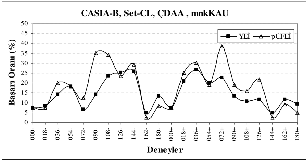
Şekil 3.36. Yürüyüş örüntülerinin karşılaştırılması: CASIA-B Set-CL’de komşu açı test sonuçları
