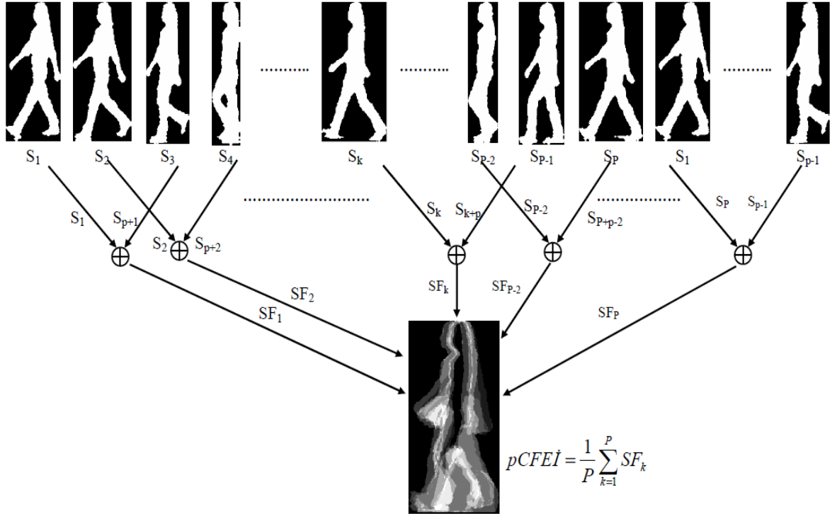
Şekil 2.4. pCFEI'nin üretilişi
