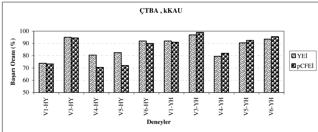
Şekil 3.27. YEİ ve pCFEİ'nin karşılaştırılması: CMU veritabanında ÇDAA+kKAU yaklaşımıyla sınıflandırma
