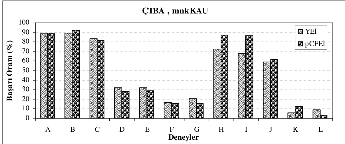
Şekil 3.31. Yürüyüş örüntülerinin karşılaştırılması: USF V2 veritabanında ÇTBA+mnkKAU yaklaşımıyla sınıflandırma
