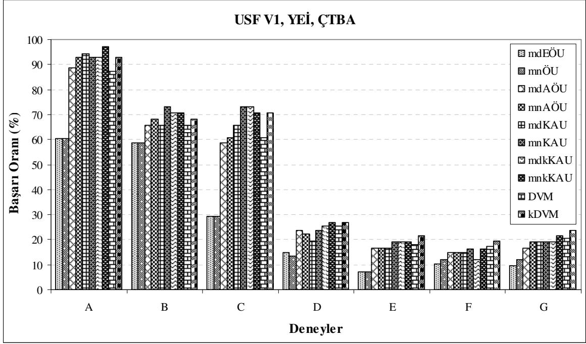
Şekil 3.9. Sınıflandırıcıların karşılaştırılması: USF V1 veritabanında YEİ örüntülerinden, ÇTBA ile çıkarılan özneliliklerin sınıflandırılması
