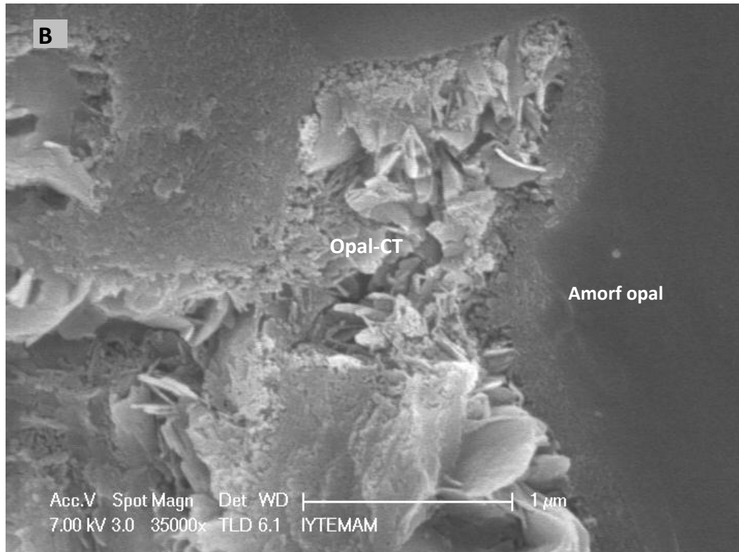
Şekil 3.26 Simav bölgesi ateş opallerinde amorf opalleri ornatan opal-CT oluşumların SEM görüntüleri.
