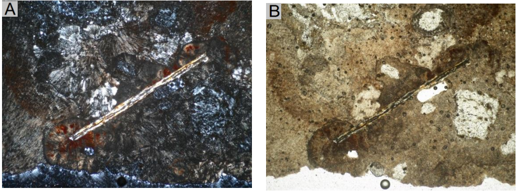
Şekil 3.12 Simav bölgesi ateş opallerin ince kesit mikroskop görüntüleri. A ve B ‘de spherolitik dokular ve kalsedonik matriks bulunur (A, haç nikol; B, paralel nikol).
