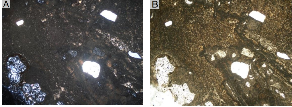
Şekil 3.11 Simav bölgesi ateş opallerin ince kesit mikroskop görüntüleri. A ve B’ de zeolitik boşluk dolguları vardır. Parlak beyaz olanlar kuvarstır. Az miktarda sanidin (K-feldispat) vardır (A, haç nikol; B, paralel nikol).
