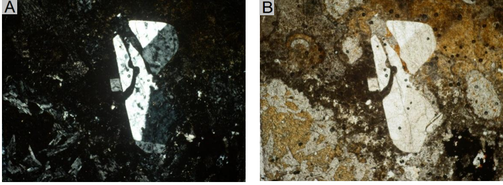
Şekil 3.13 Simav bölgesi ateş opallerin ince kesit mikroskop görüntüleri. Sanidin ikizlenme vardır. A’de siyah olarak gözüken opaller B’de sarı renkte belirgindir (A, haç nikol; B, paralel nikol)
