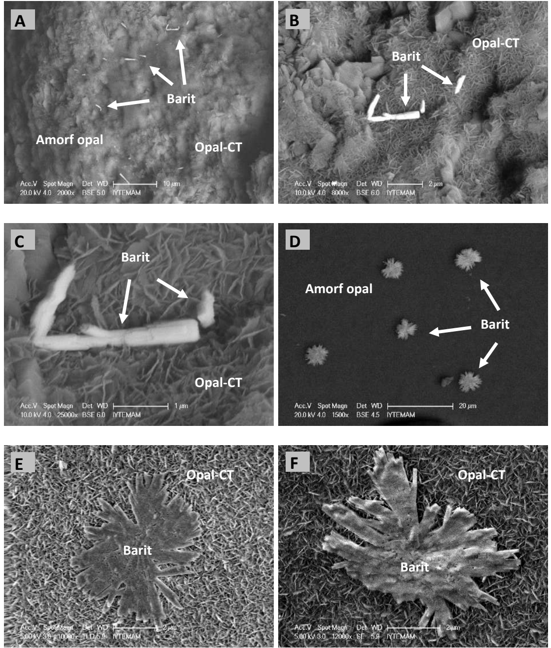
Şekil 3.30 Simav bölgesi ateş opalleri içinde gözlenen özşekli ve rozet yapılı-ışınsal barit oluşumlarının SEM görüntüleri.
