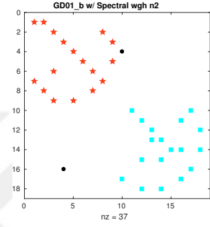
(d) Weighted, nproc = 2, spy rep.
