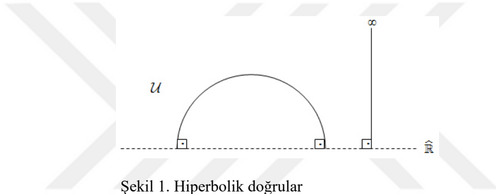
Şekil 1. Hiperbolik doğrular
