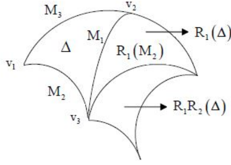
Şekil 5. R_1(\Delta) , R_1R_2(\Delta) \mathbb{H} -üçgenleri
